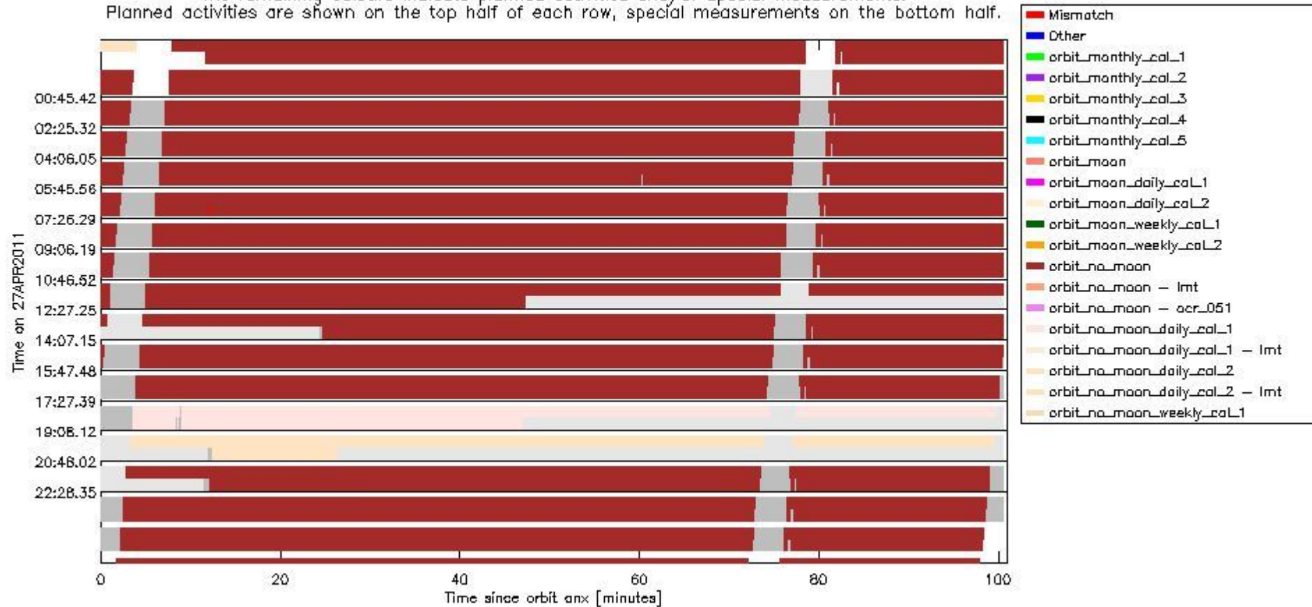
sciamachy_daily_report_level0_KSPT_L0_4504_N_20110427_6.PNG
