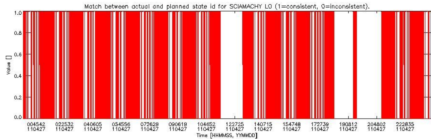
sciamachy_daily_report_level0_KSPT_L0_4504_N_20110427_5.PNG
