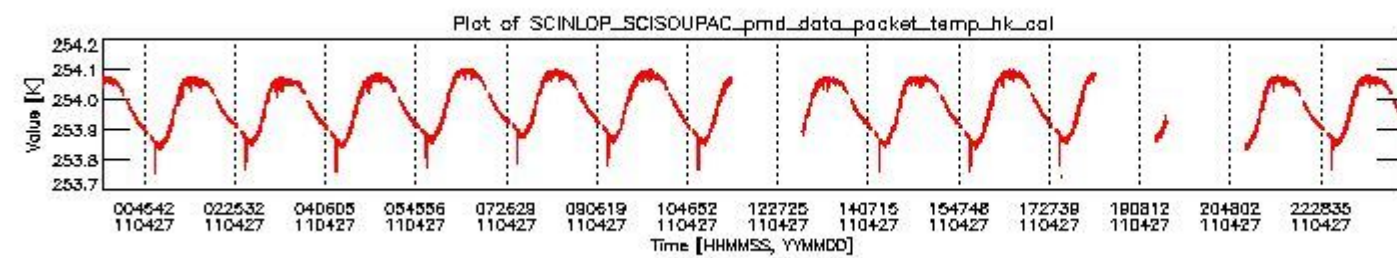
sciamachy_daily_report_level0_KSPT_L0_4504_N_20110427_3.PNG
