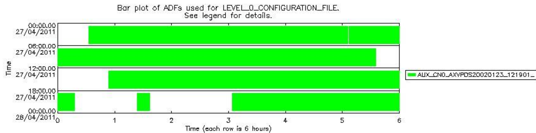
sciamachy_daily_report_level0_KSPT_L0_4504_N_20110427_7.PNG
