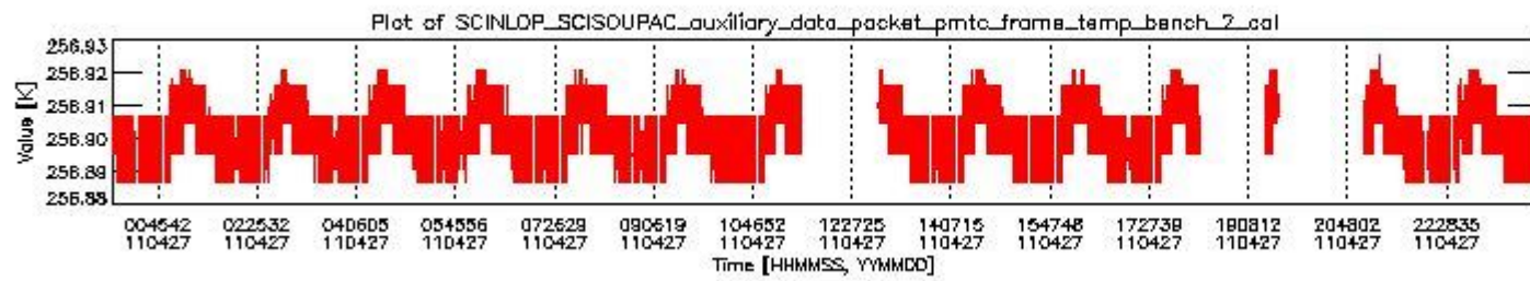
sciamachy_daily_report_level0_KSPT_L0_4504_N_20110427_1.PNG
