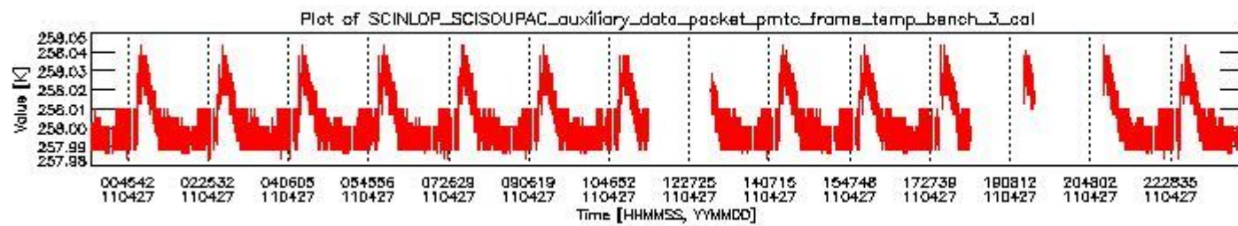
sciamachy_daily_report_level0_KSPT_L0_4504_N_20110427_2.PNG
