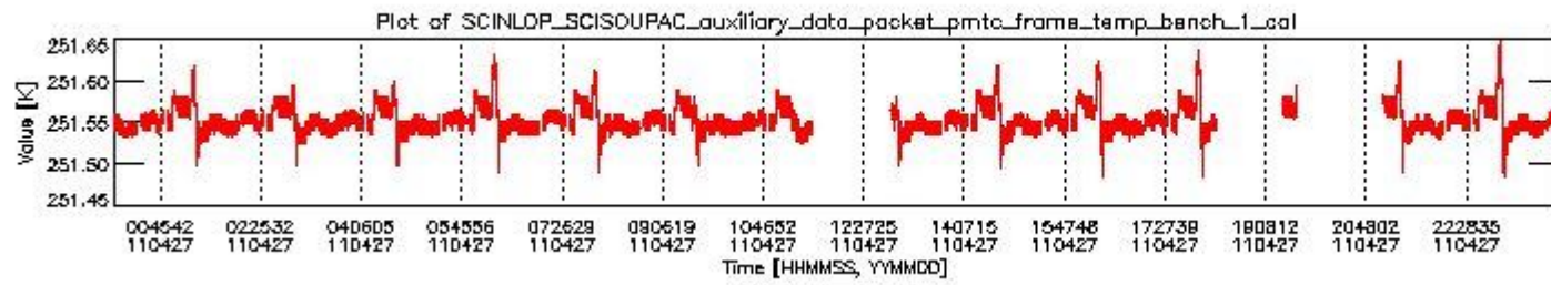
sciamachy_daily_report_level0_KSPT_L0_4504_N_20110427_0.PNG
