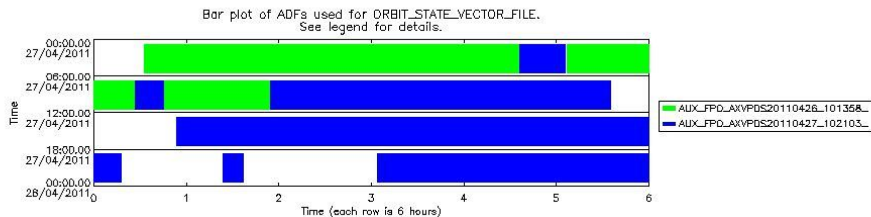
sciamachy_daily_report_level0_KSPT_L0_4504_N_20110427_8.PNG
