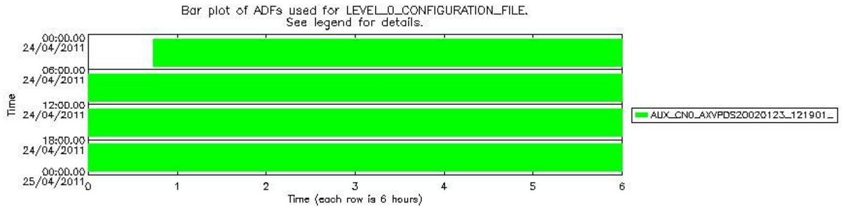
sciamachy_daily_report_level0_KSPT_L0_4504_N_20110424_7.PNG
