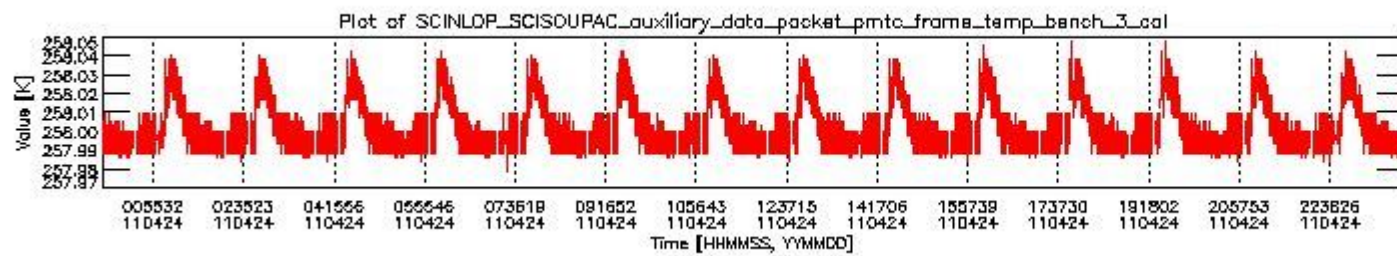
sciamachy_daily_report_level0_KSPT_L0_4504_N_20110424_2.PNG
