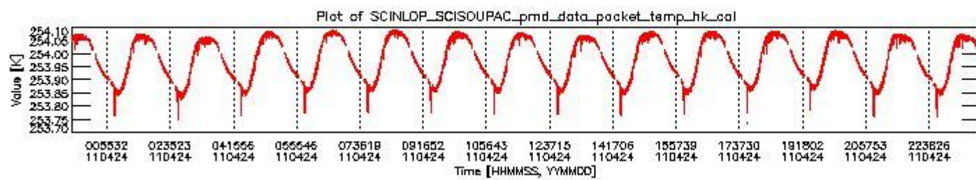
sciamachy_daily_report_level0_KSPT_L0_4504_N_20110424_3.PNG
