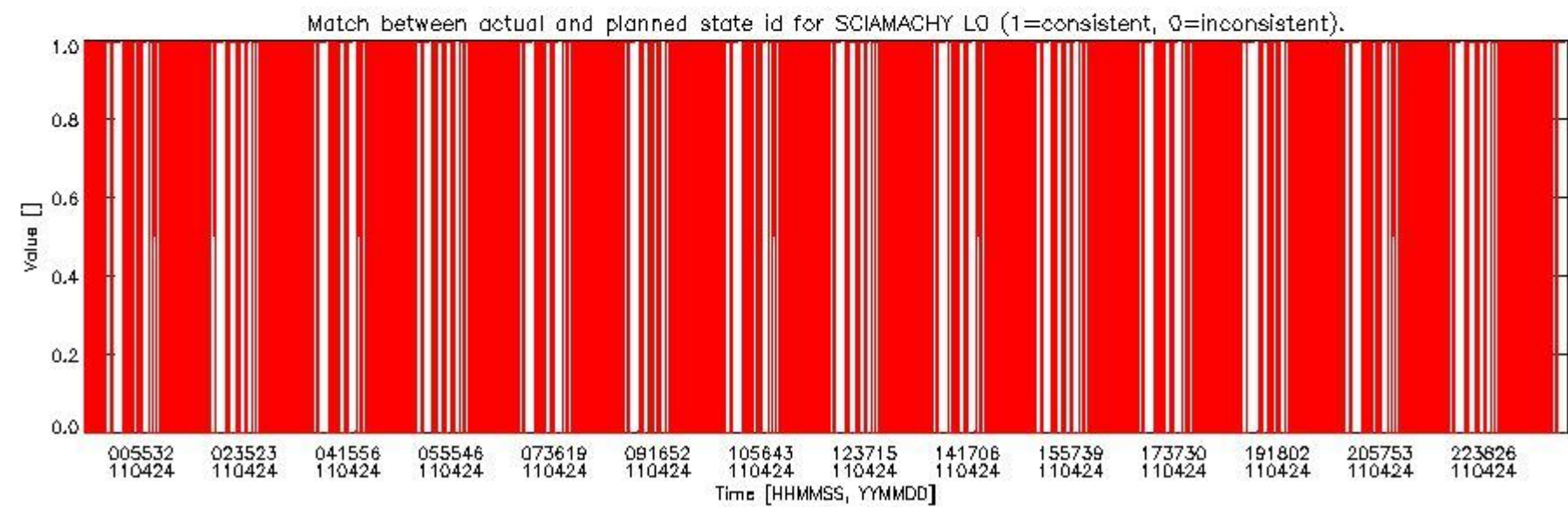
sciamachy_daily_report_level0_KSPT_L0_4504_N_20110424_5.PNG
