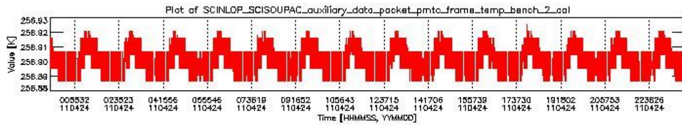
sciamachy_daily_report_level0_KSPT_L0_4504_N_20110424_1.PNG
