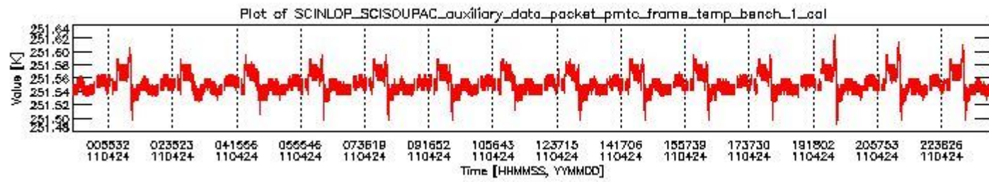
sciamachy_daily_report_level0_KSPT_L0_4504_N_20110424_0.PNG
