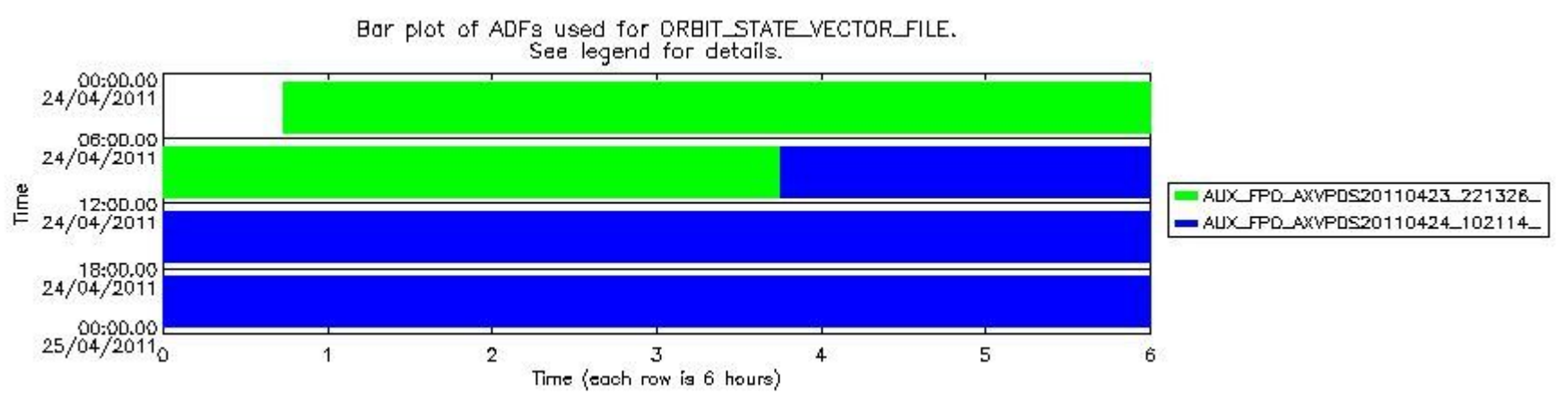
sciamachy_daily_report_level0_KSPT_L0_4504_N_20110424_8.PNG
