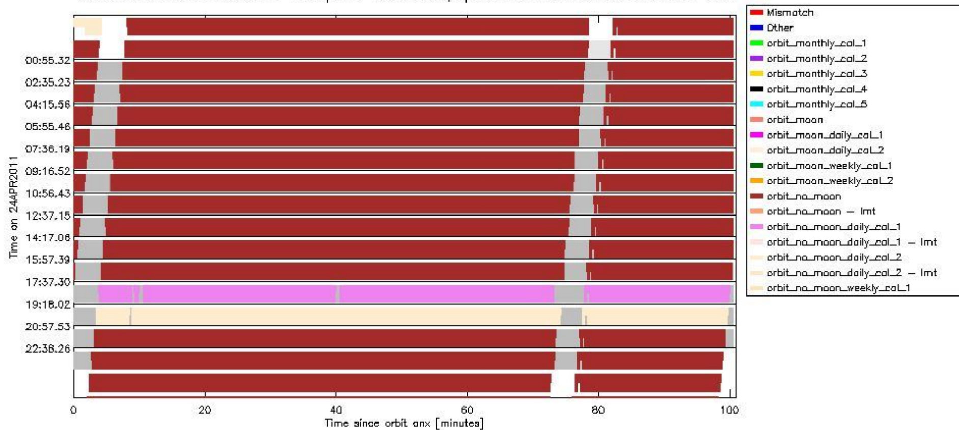
sciamachy_daily_report_level0_KSPT_L0_4504_N_20110424_6.PNG
