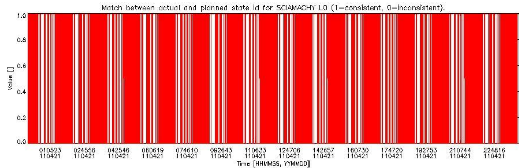
sciamachy_daily_report_level0_KSPT_L0_4504_N_20110421_5.PNG
