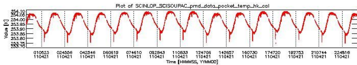
sciamachy_daily_report_level0_KSPT_L0_4504_N_20110421_3.PNG
