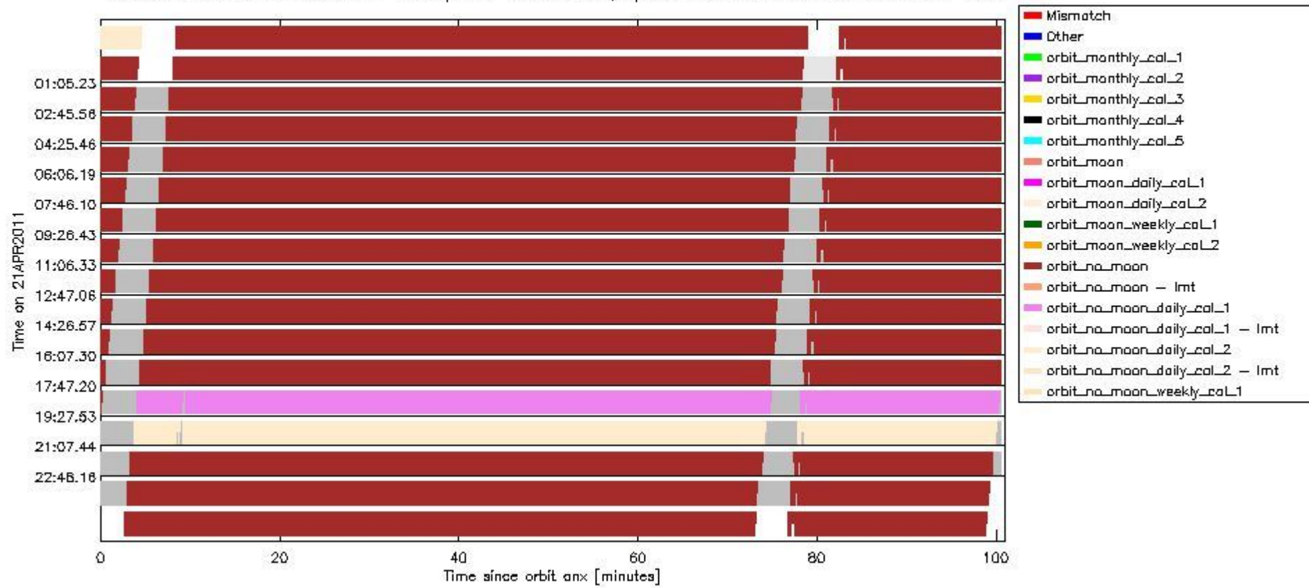
sciamachy_daily_report_level0_KSPT_L0_4504_N_20110421_6.PNG
