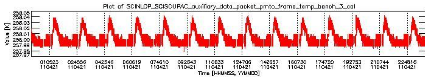
sciamachy_daily_report_level0_KSPT_L0_4504_N_20110421_2.PNG
