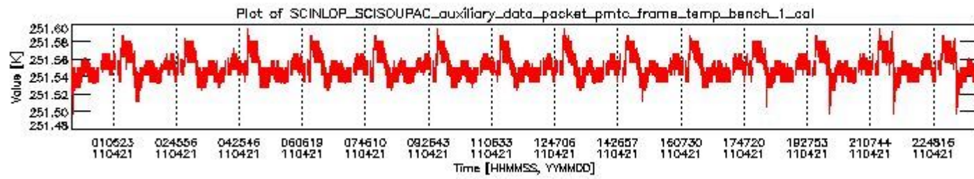
sciamachy_daily_report_level0_KSPT_L0_4504_N_20110421_0.PNG
