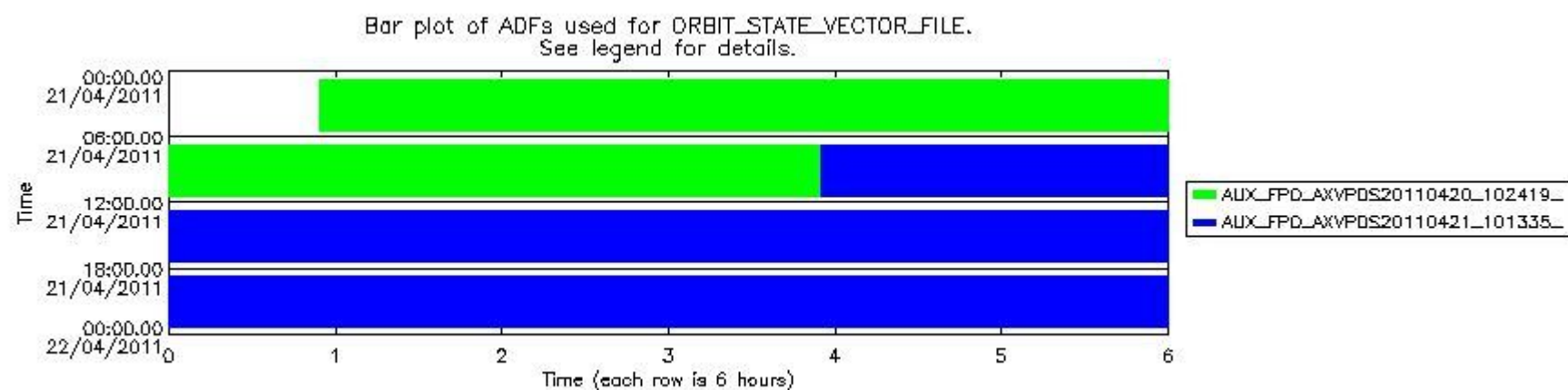
sciamachy_daily_report_level0_KSPT_L0_4504_N_20110421_8.PNG
