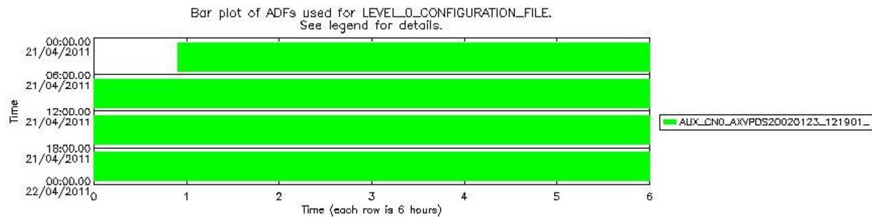
sciamachy_daily_report_level0_KSPT_L0_4504_N_20110421_7.PNG
