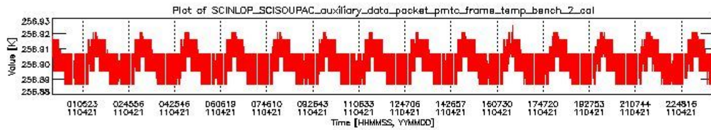
sciamachy_daily_report_level0_KSPT_L0_4504_N_20110421_1.PNG
