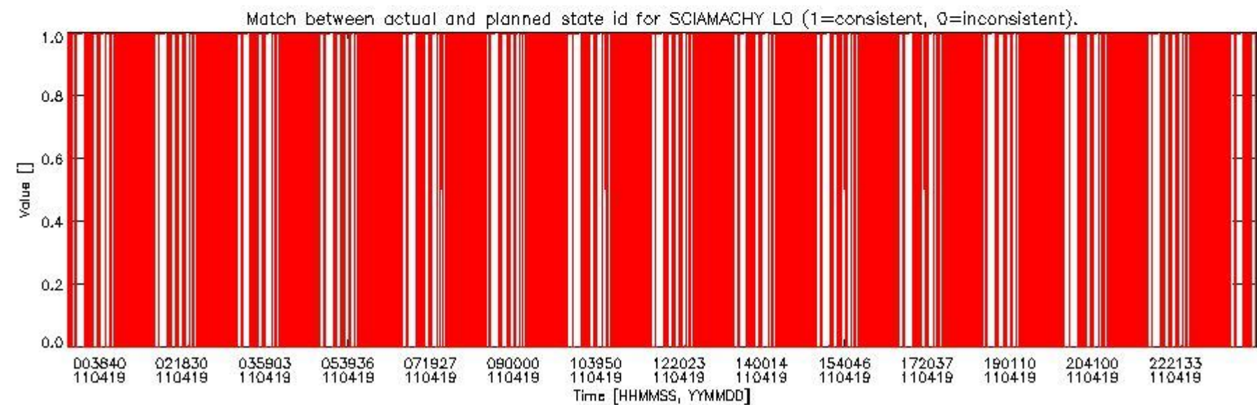
sciamachy_daily_report_level0_KSPT_L0_4504_N_20110419_5.PNG
