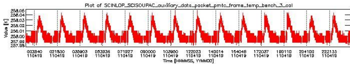
sciamachy_daily_report_level0_KSPT_L0_4504_N_20110419_2.PNG
