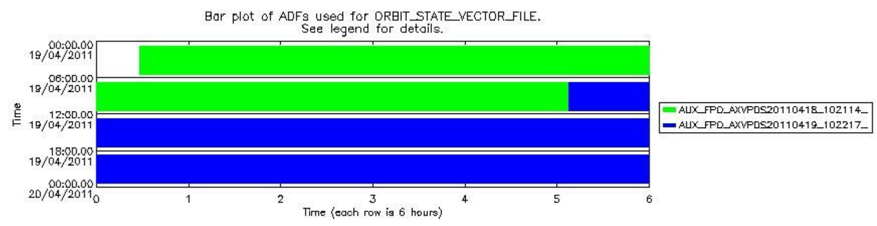
sciamachy_daily_report_level0_KSPT_L0_4504_N_20110419_8.PNG
