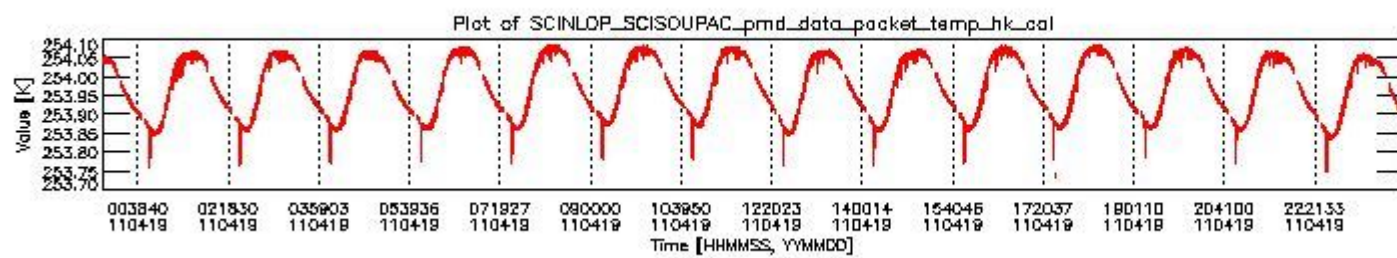
sciamachy_daily_report_level0_KSPT_L0_4504_N_20110419_3.PNG
