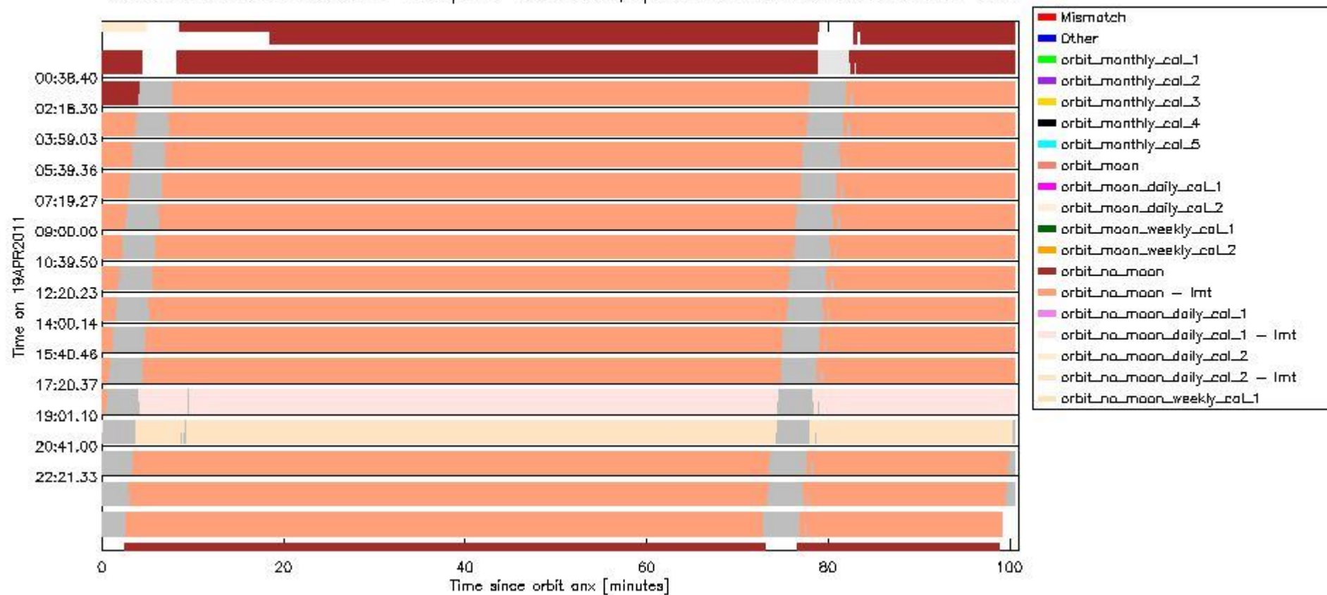
sciamachy_daily_report_level0_KSPT_L0_4504_N_20110419_6.PNG
