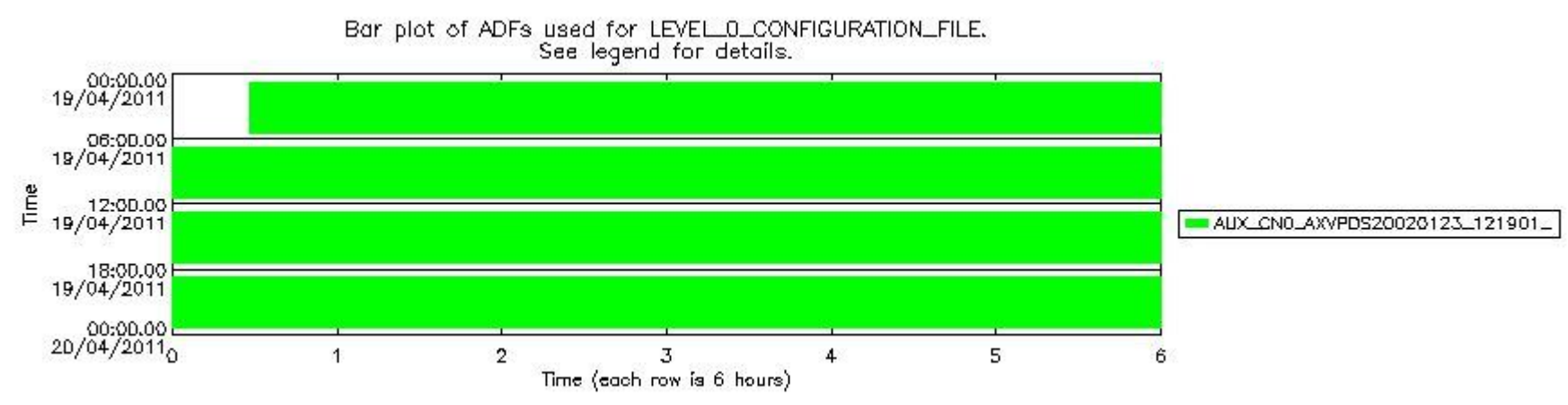
sciamachy_daily_report_level0_KSPT_L0_4504_N_20110419_7.PNG
