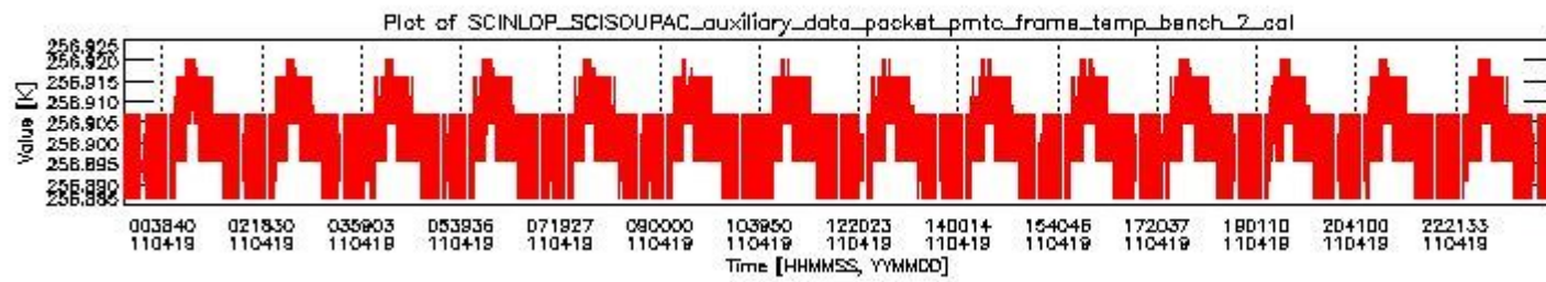
sciamachy_daily_report_level0_KSPT_L0_4504_N_20110419_1.PNG
