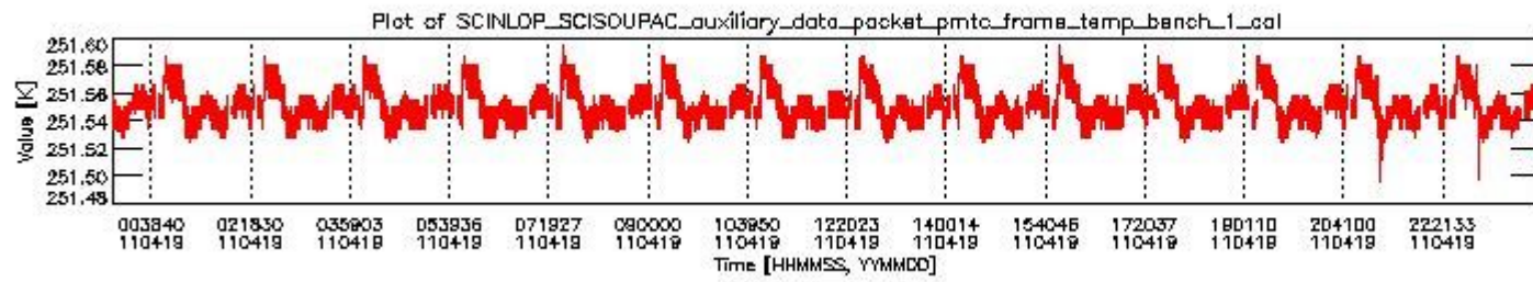
sciamachy_daily_report_level0_KSPT_L0_4504_N_20110419_0.PNG
