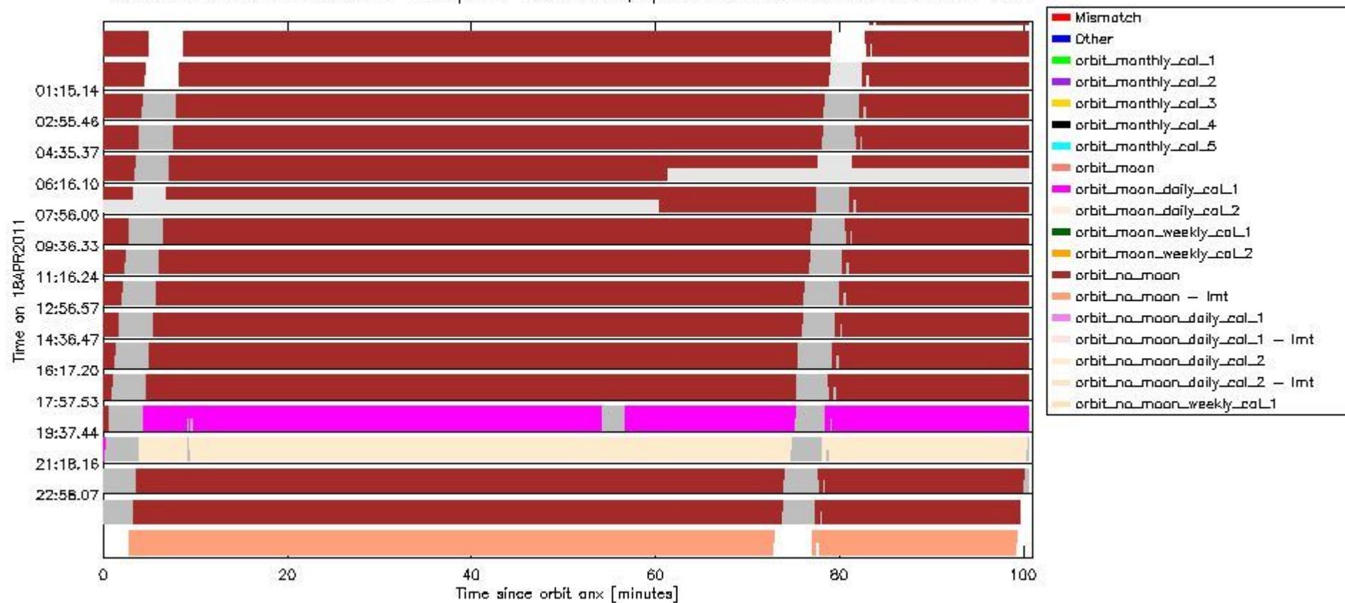
sciamachy_daily_report_level0_KSPT_L0_4504_N_20110418_6.PNG
