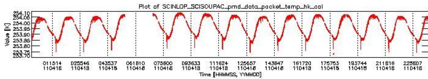
sciamachy_daily_report_level0_KSPT_L0_4504_N_20110418_3.PNG
