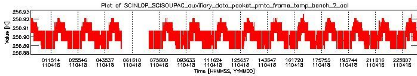
sciamachy_daily_report_level0_KSPT_L0_4504_N_20110418_1.PNG
