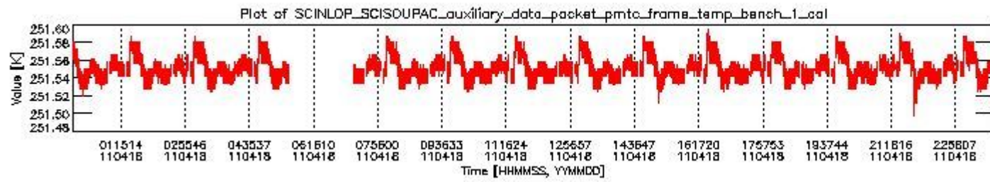
sciamachy_daily_report_level0_KSPT_L0_4504_N_20110418_0.PNG
