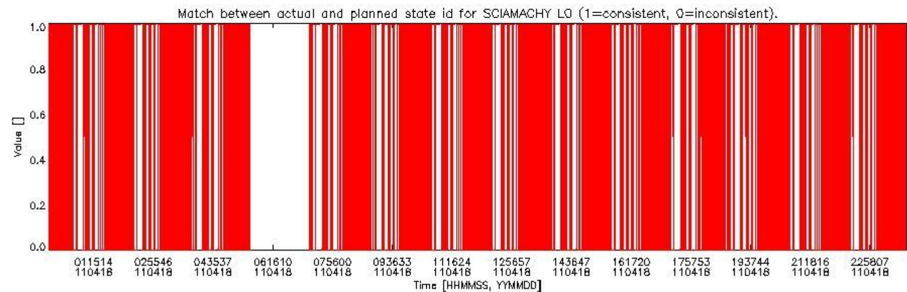
sciamachy_daily_report_level0_KSPT_L0_4504_N_20110418_5.PNG
