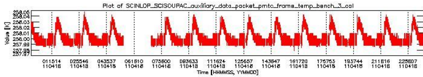
sciamachy_daily_report_level0_KSPT_L0_4504_N_20110418_2.PNG
