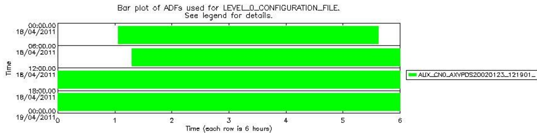
sciamachy_daily_report_level0_KSPT_L0_4504_N_20110418_7.PNG
