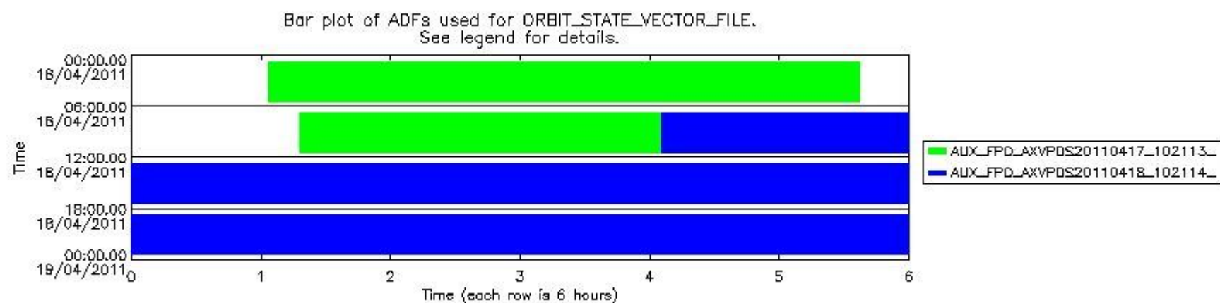
sciamachy_daily_report_level0_KSPT_L0_4504_N_20110418_8.PNG
