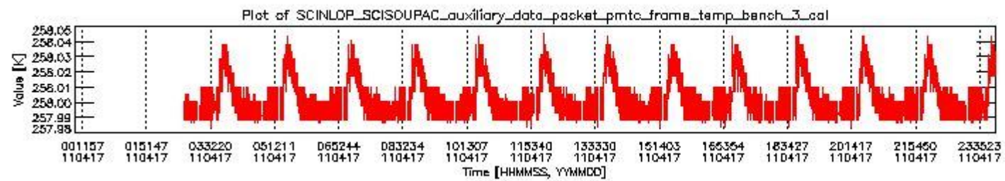
sciamachy_daily_report_level0_KSPT_L0_4504_N_20110417_2.PNG
