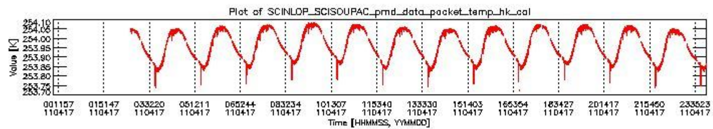
sciamachy_daily_report_level0_KSPT_L0_4504_N_20110417_3.PNG
