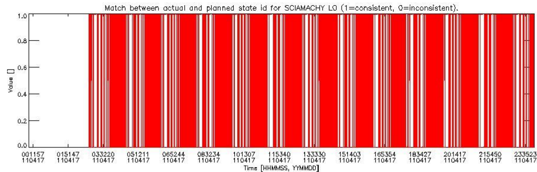
sciamachy_daily_report_level0_KSPT_L0_4504_N_20110417_5.PNG
