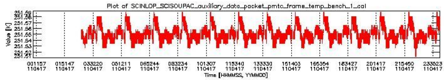
sciamachy_daily_report_level0_KSPT_L0_4504_N_20110417_0.PNG
