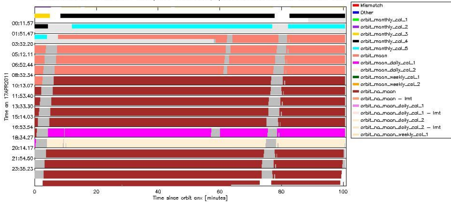
sciamachy_daily_report_level0_KSPT_L0_4504_N_20110417_6.PNG
