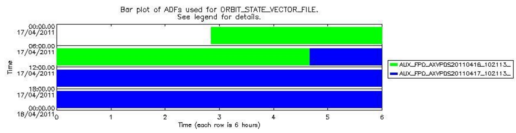
sciamachy_daily_report_level0_KSPT_L0_4504_N_20110417_8.PNG
