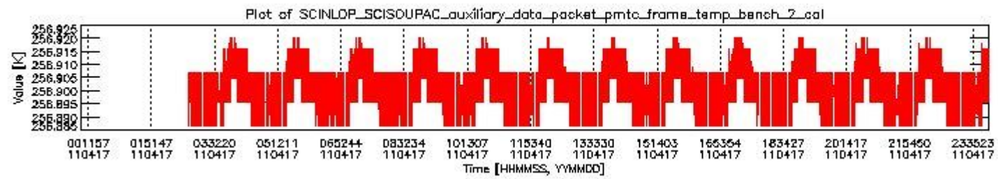
sciamachy_daily_report_level0_KSPT_L0_4504_N_20110417_1.PNG
