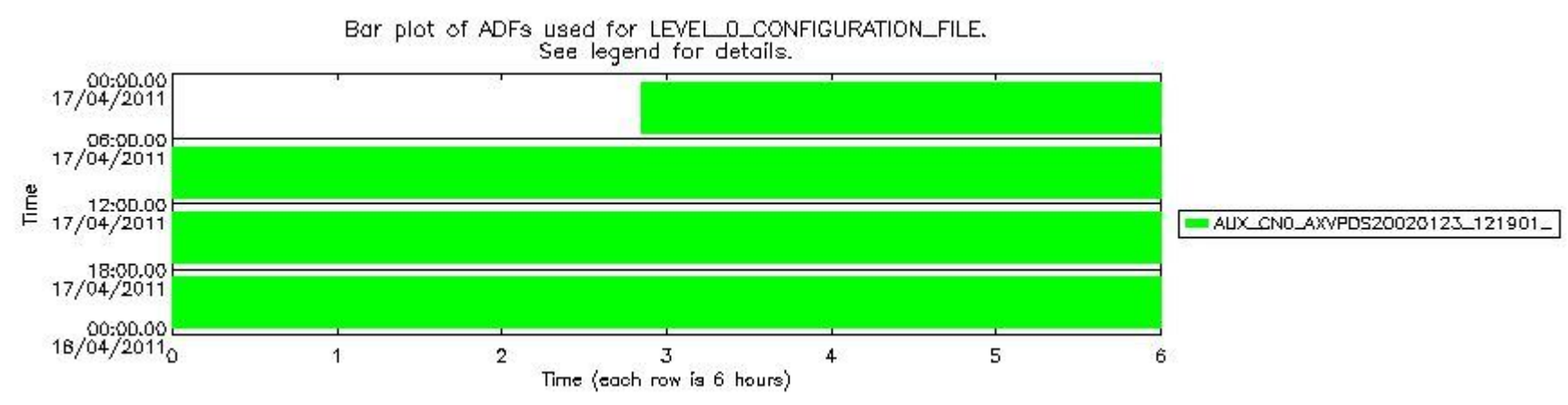
sciamachy_daily_report_level0_KSPT_L0_4504_N_20110417_7.PNG
