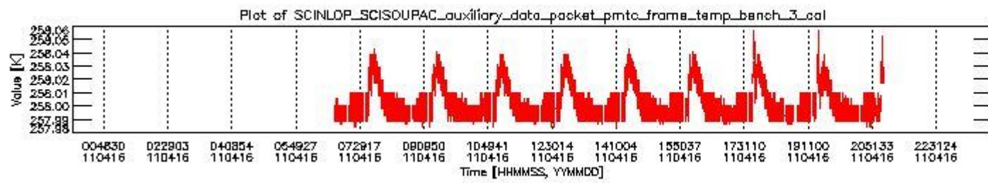
sciamachy_daily_report_level0_KSPT_L0_4504_N_20110416_2.PNG
