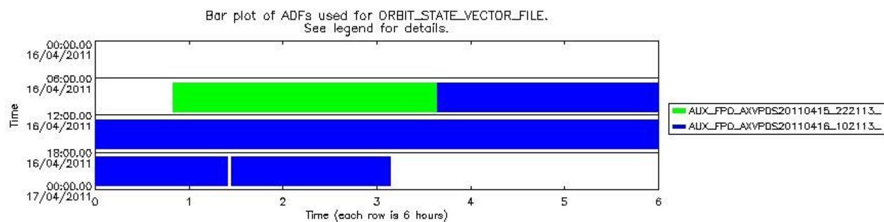
sciamachy_daily_report_level0_KSPT_L0_4504_N_20110416_8.PNG
