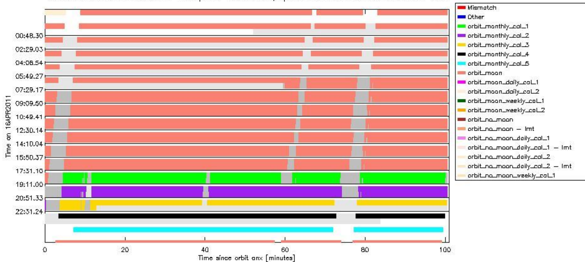
sciamachy_daily_report_level0_KSPT_L0_4504_N_20110416_6.PNG
