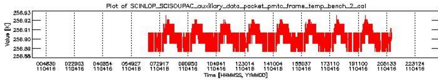
sciamachy_daily_report_level0_KSPT_L0_4504_N_20110416_1.PNG
