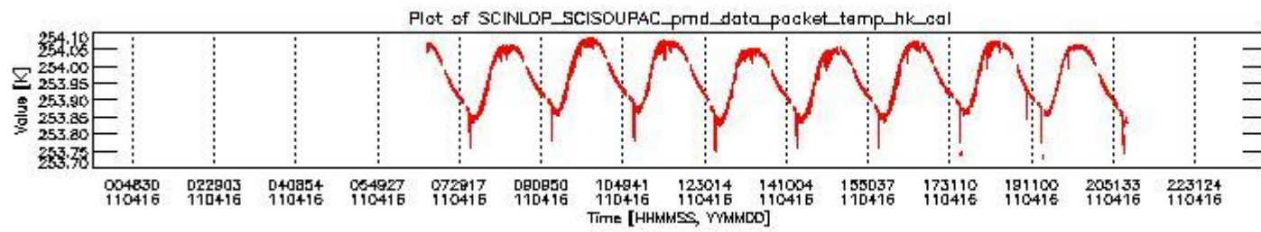
sciamachy_daily_report_level0_KSPT_L0_4504_N_20110416_3.PNG
