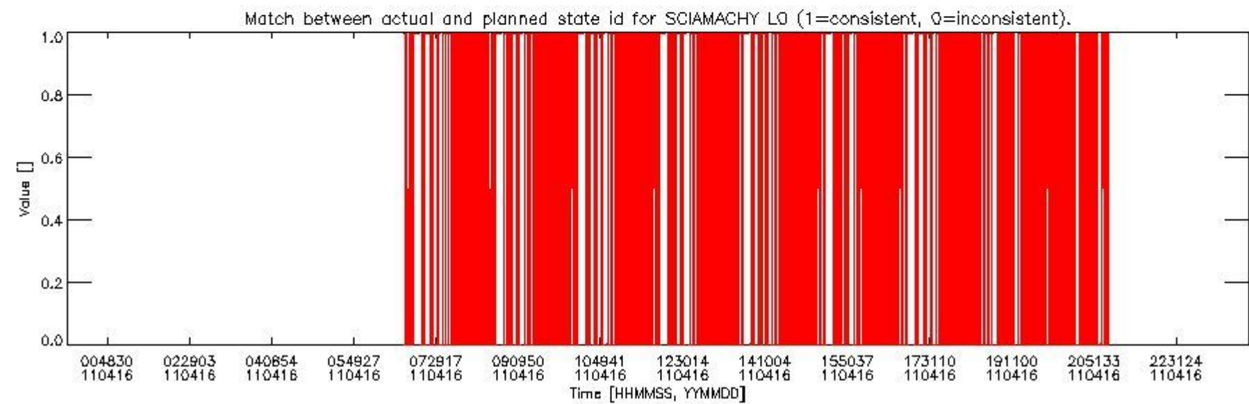
sciamachy_daily_report_level0_KSPT_L0_4504_N_20110416_5.PNG
