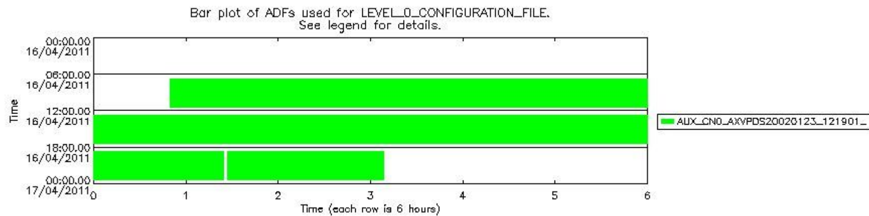
sciamachy_daily_report_level0_KSPT_L0_4504_N_20110416_7.PNG
