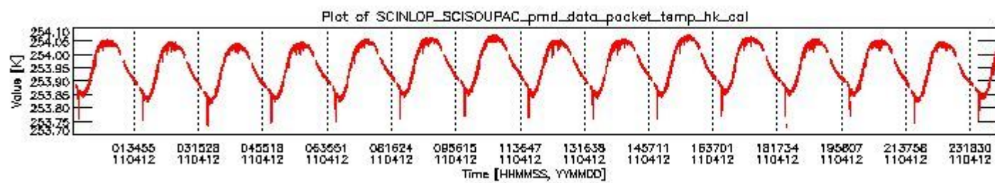
sciamachy_daily_report_level0_KSPT_L0_4504_N_20110412_3.PNG
