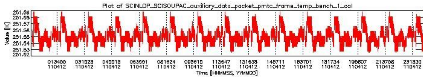
sciamachy_daily_report_level0_KSPT_L0_4504_N_20110412_0.PNG
