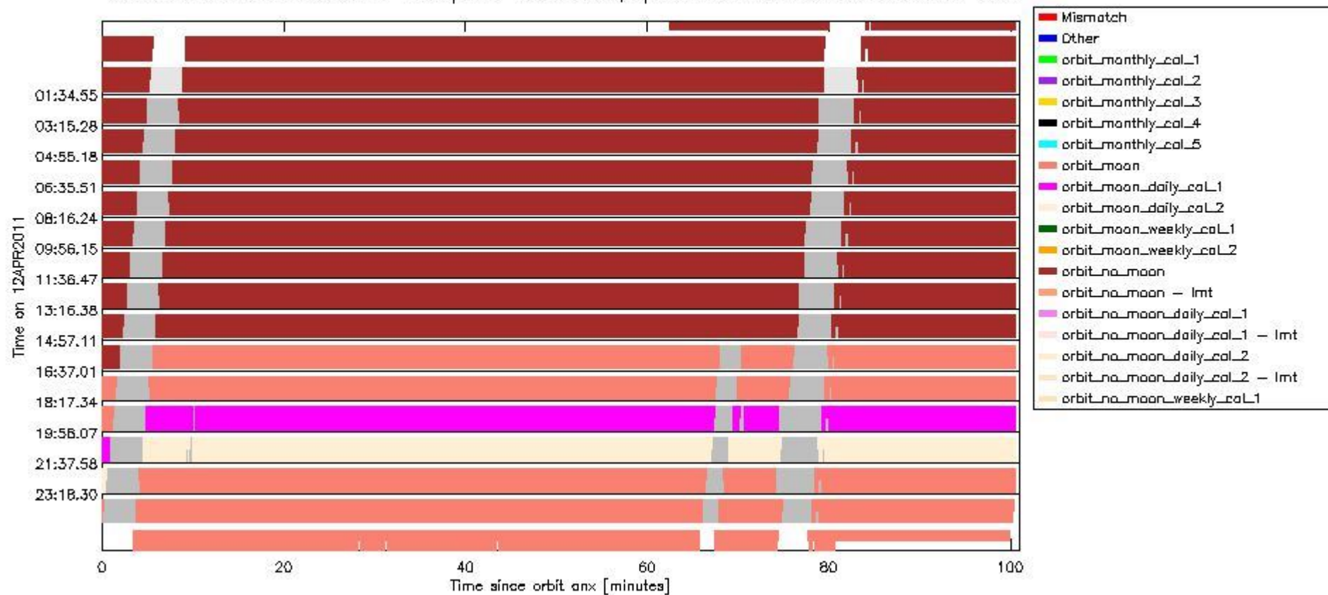
sciamachy_daily_report_level0_KSPT_L0_4504_N_20110412_6.PNG
