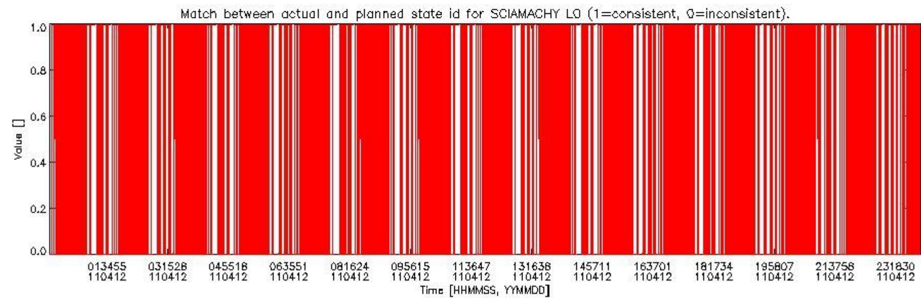
sciamachy_daily_report_level0_KSPT_L0_4504_N_20110412_5.PNG
