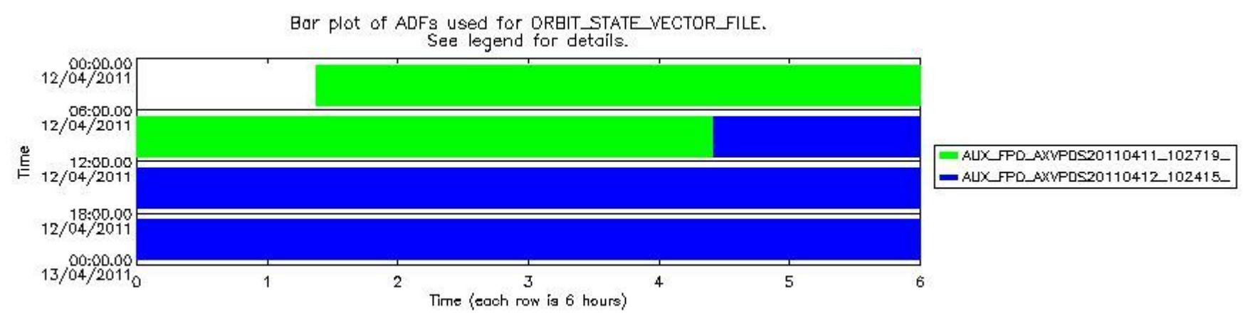
sciamachy_daily_report_level0_KSPT_L0_4504_N_20110412_8.PNG
