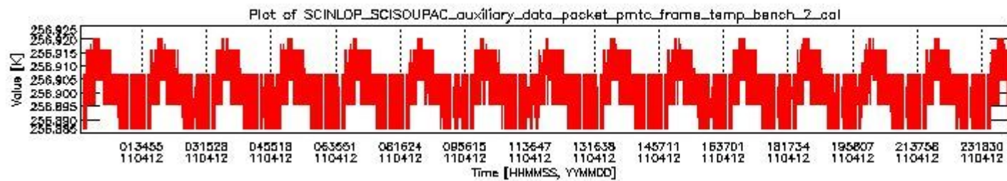
sciamachy_daily_report_level0_KSPT_L0_4504_N_20110412_1.PNG
