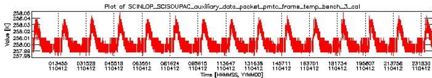
sciamachy_daily_report_level0_KSPT_L0_4504_N_20110412_2.PNG
