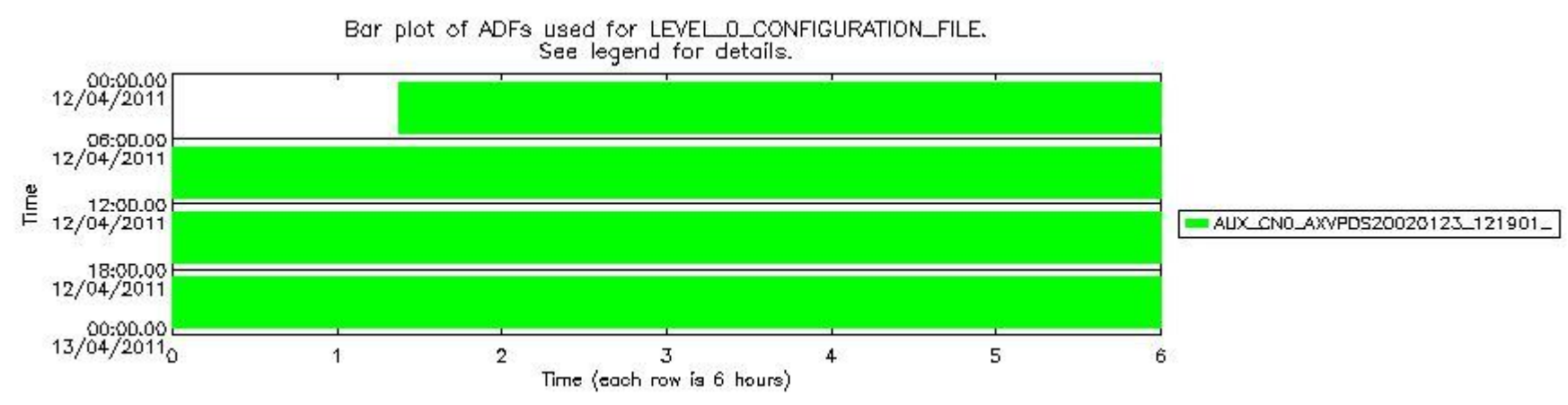
sciamachy_daily_report_level0_KSPT_L0_4504_N_20110412_7.PNG
