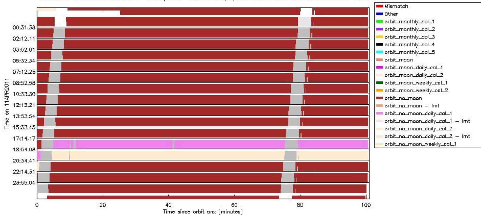
sciamachy_daily_report_level0_KSPT_L0_4504_N_20110411_6.PNG
