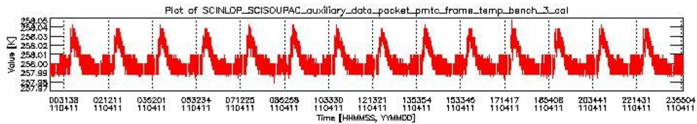
sciamachy_daily_report_level0_KSPT_L0_4504_N_20110411_2.PNG
