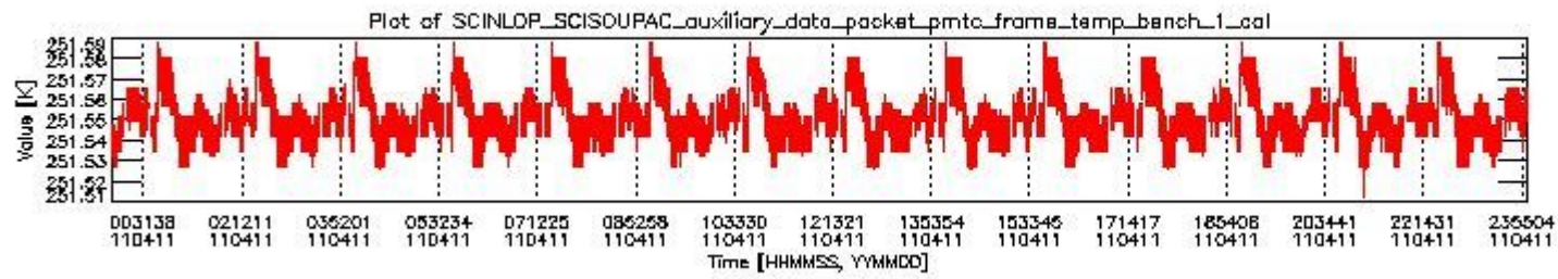
sciamachy_daily_report_level0_KSPT_L0_4504_N_20110411_0.PNG
