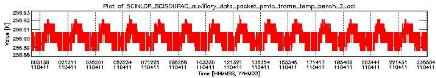
sciamachy_daily_report_level0_KSPT_L0_4504_N_20110411_1.PNG
