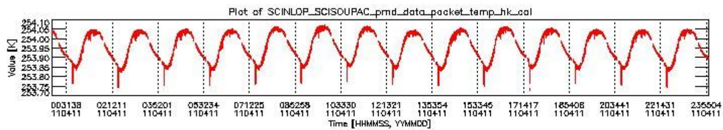
sciamachy_daily_report_level0_KSPT_L0_4504_N_20110411_3.PNG
