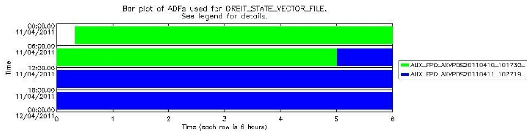
sciamachy_daily_report_level0_KSPT_L0_4504_N_20110411_8.PNG
