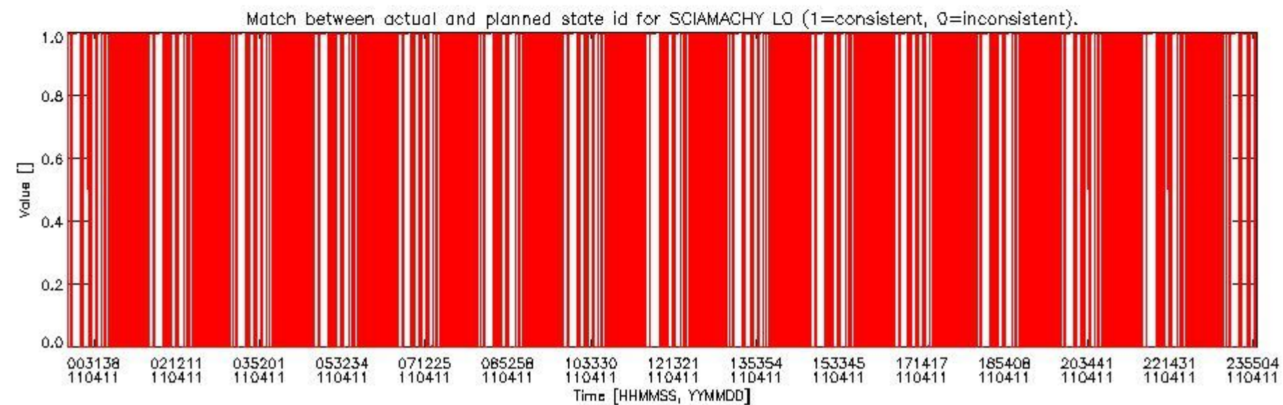
sciamachy_daily_report_level0_KSPT_L0_4504_N_20110411_5.PNG
