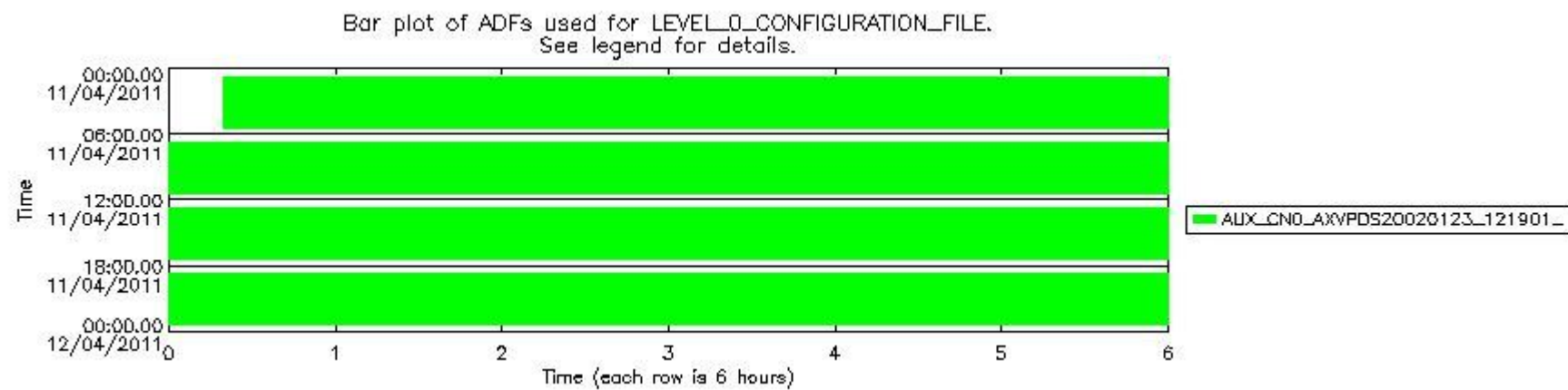
sciamachy_daily_report_level0_KSPT_L0_4504_N_20110411_7.PNG
