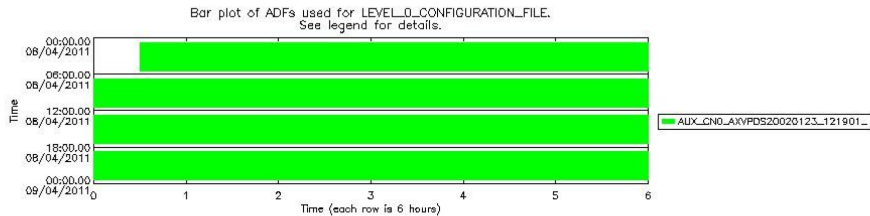
sciamachy_daily_report_level0_KSPT_L0_4504_N_20110408_7.PNG
