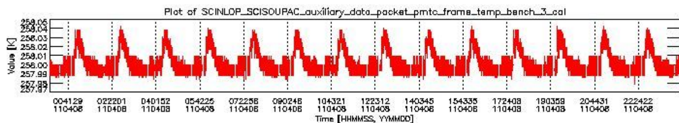
sciamachy_daily_report_level0_KSPT_L0_4504_N_20110408_2.PNG
