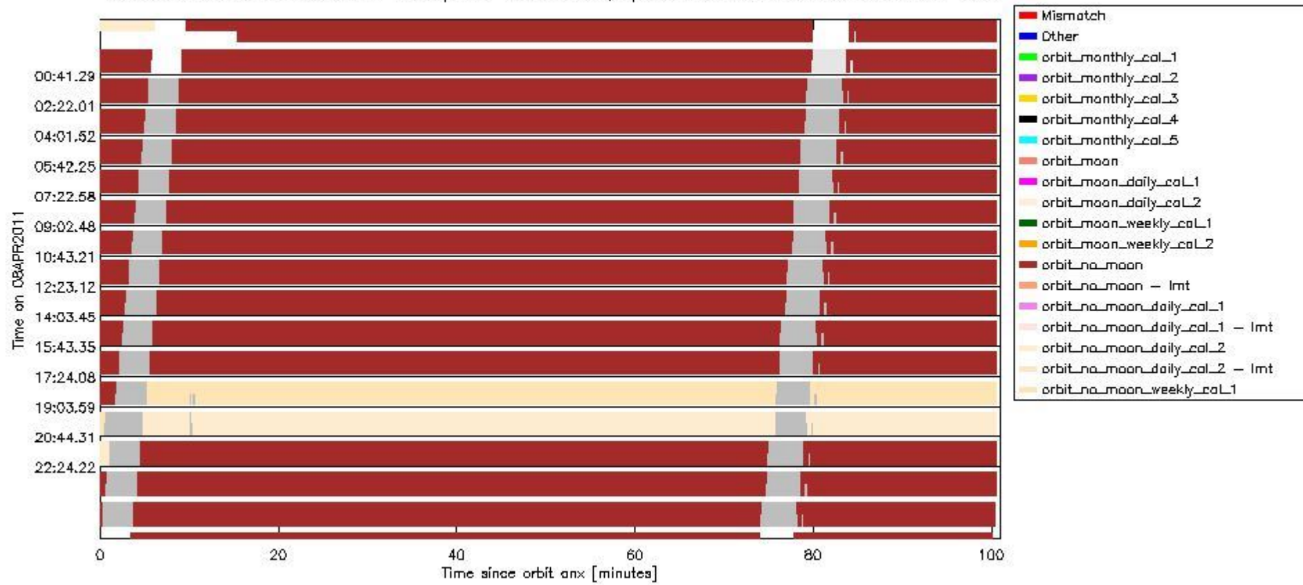
sciamachy_daily_report_level0_KSPT_L0_4504_N_20110408_6.PNG
