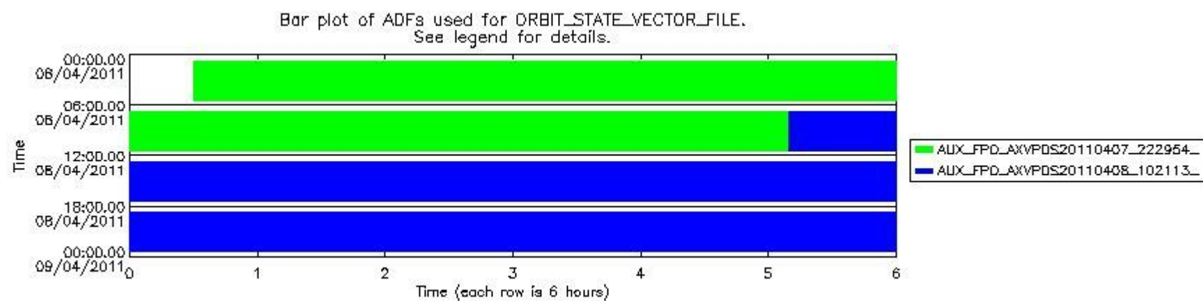
sciamachy_daily_report_level0_KSPT_L0_4504_N_20110408_8.PNG
