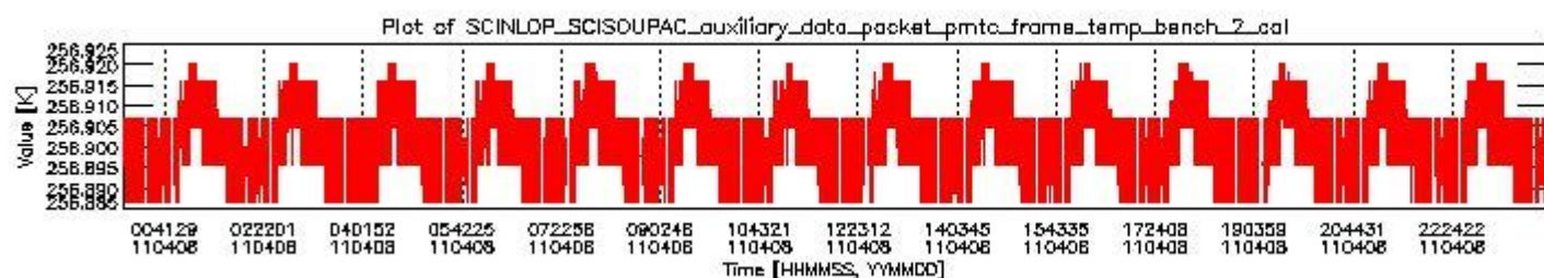
sciamachy_daily_report_level0_KSPT_L0_4504_N_20110408_1.PNG
