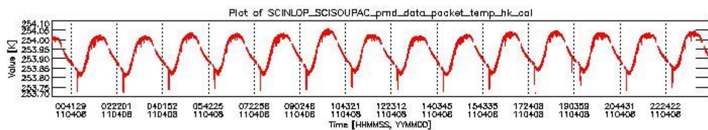
sciamachy_daily_report_level0_KSPT_L0_4504_N_20110408_3.PNG
