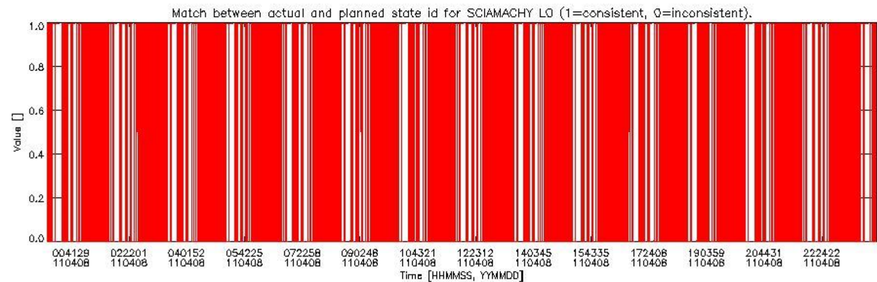
sciamachy_daily_report_level0_KSPT_L0_4504_N_20110408_5.PNG
