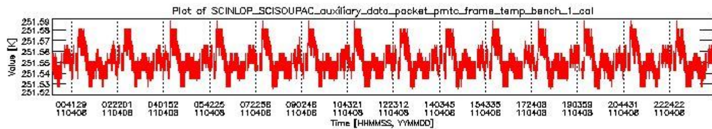
sciamachy_daily_report_level0_KSPT_L0_4504_N_20110408_0.PNG
