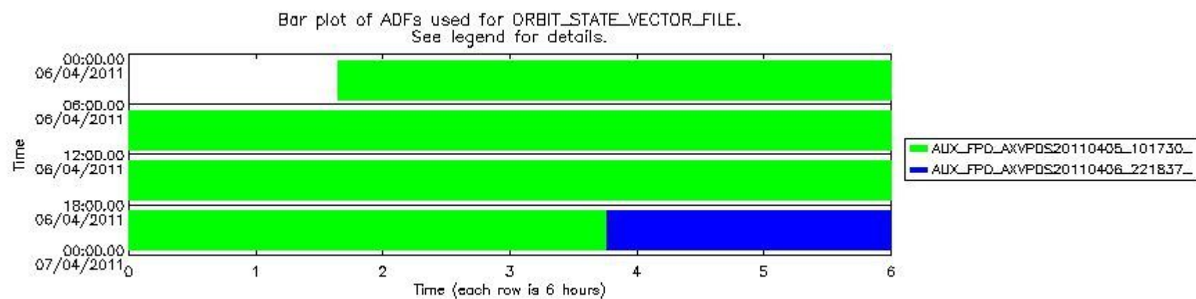
sciamachy_daily_report_level0_KSPT_L0_4504_N_20110406_8.PNG
