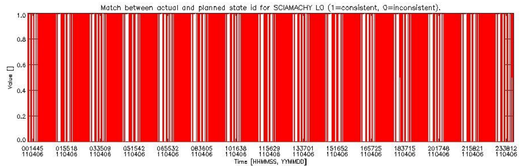
sciamachy_daily_report_level0_KSPT_L0_4504_N_20110406_5.PNG
