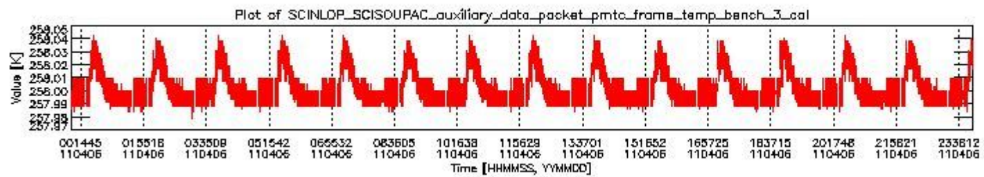
sciamachy_daily_report_level0_KSPT_L0_4504_N_20110406_2.PNG
