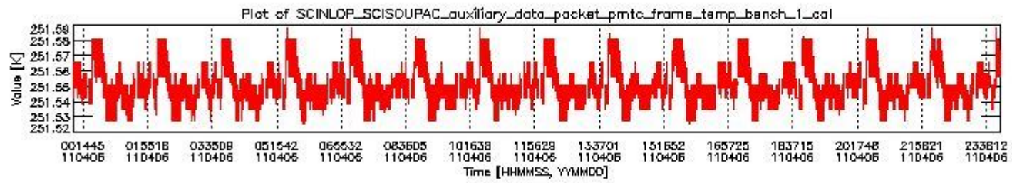
sciamachy_daily_report_level0_KSPT_L0_4504_N_20110406_0.PNG
