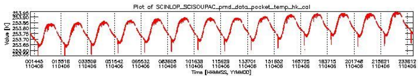
sciamachy_daily_report_level0_KSPT_L0_4504_N_20110406_3.PNG
