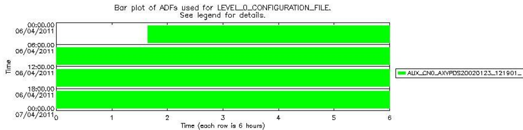
sciamachy_daily_report_level0_KSPT_L0_4504_N_20110406_7.PNG
