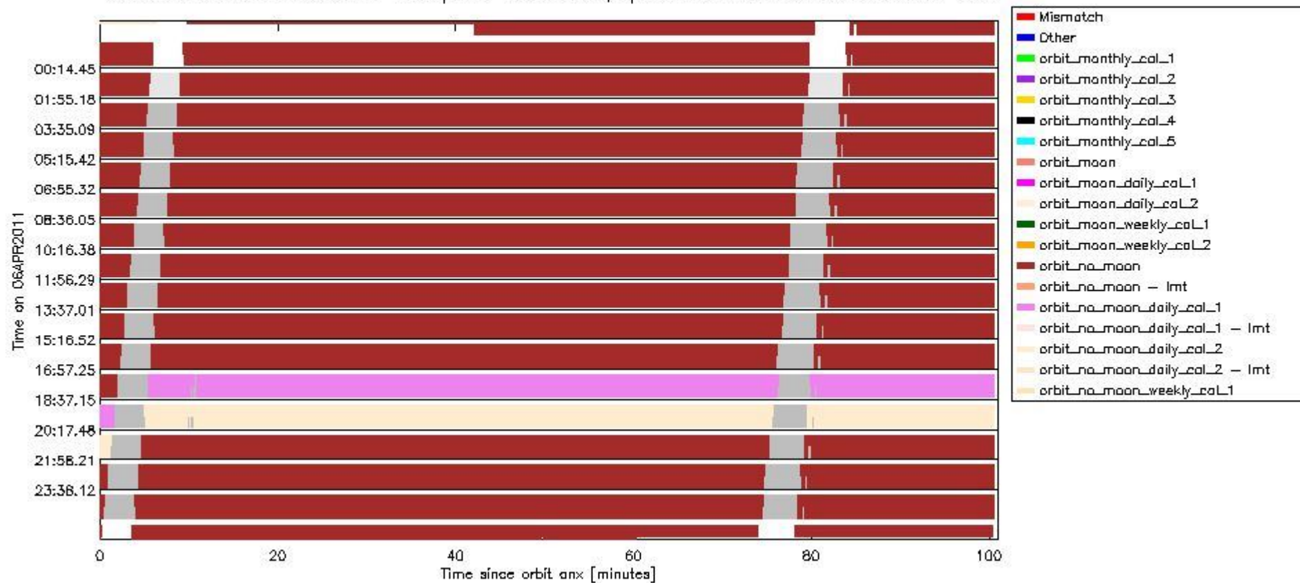
sciamachy_daily_report_level0_KSPT_L0_4504_N_20110406_6.PNG
