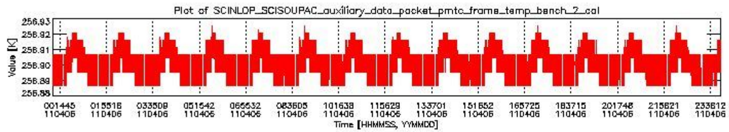
sciamachy_daily_report_level0_KSPT_L0_4504_N_20110406_1.PNG
