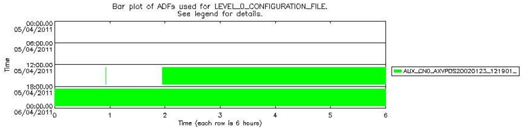
sciamachy_daily_report_level0_KSPT_L0_4504_N_20110405_7.PNG
