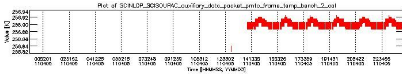
sciamachy_daily_report_level0_KSPT_L0_4504_N_20110405_1.PNG
