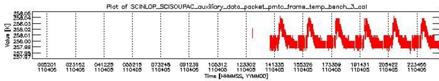
sciamachy_daily_report_level0_KSPT_L0_4504_N_20110405_2.PNG
