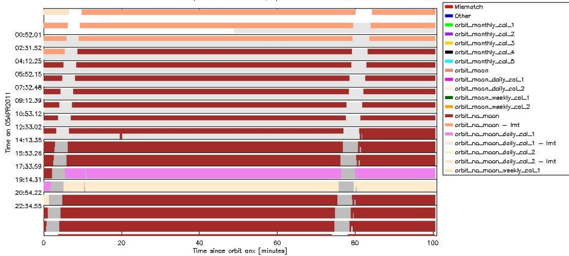
sciamachy_daily_report_level0_KSPT_L0_4504_N_20110405_6.PNG
