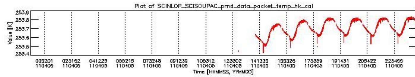
sciamachy_daily_report_level0_KSPT_L0_4504_N_20110405_3.PNG
