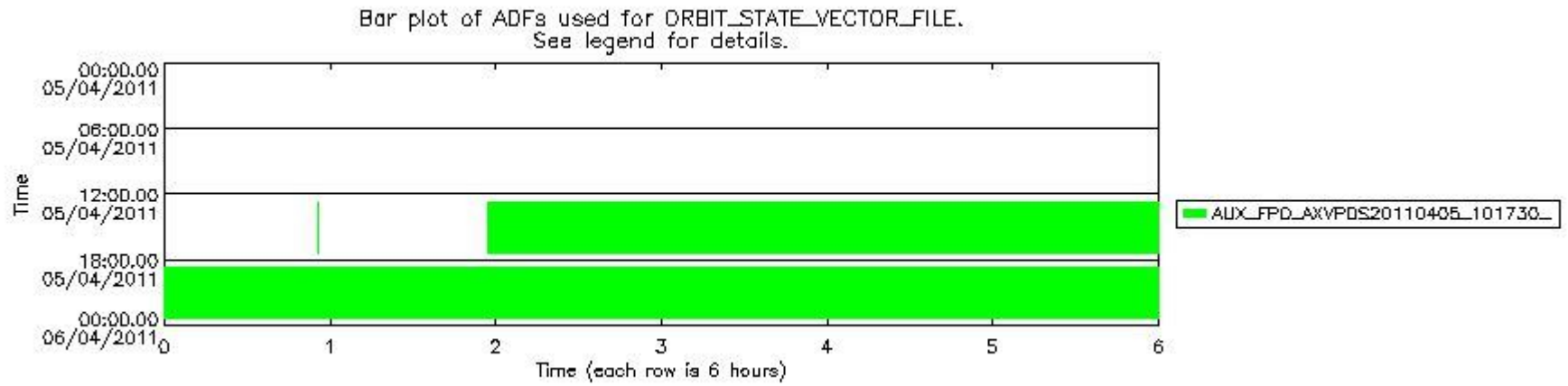
sciamachy_daily_report_level0_KSPT_L0_4504_N_20110405_8.PNG
