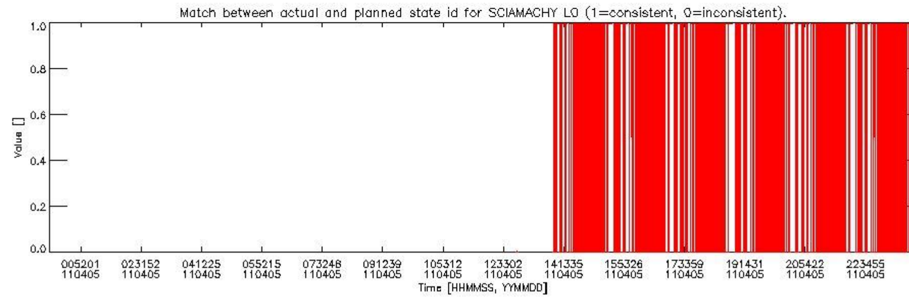
sciamachy_daily_report_level0_KSPT_L0_4504_N_20110405_5.PNG
