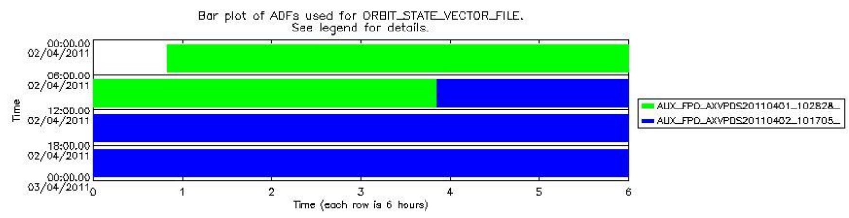
sciamachy_daily_report_level0_KSPT_L0_4504_N_20110402_8.PNG
