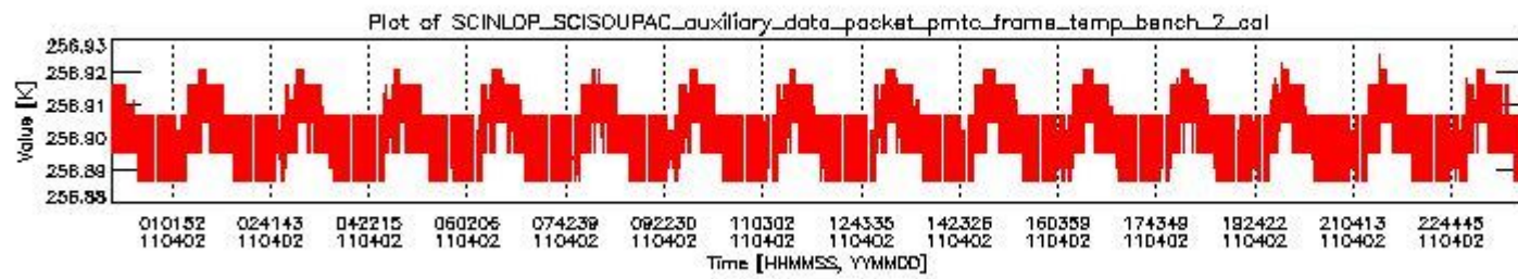
sciamachy_daily_report_level0_KSPT_L0_4504_N_20110402_1.PNG
