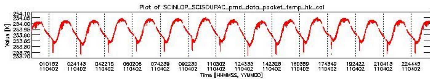
sciamachy_daily_report_level0_KSPT_L0_4504_N_20110402_3.PNG
