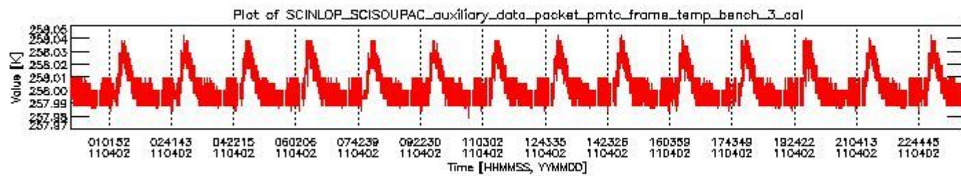
sciamachy_daily_report_level0_KSPT_L0_4504_N_20110402_2.PNG
