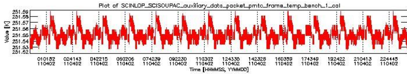
sciamachy_daily_report_level0_KSPT_L0_4504_N_20110402_0.PNG
