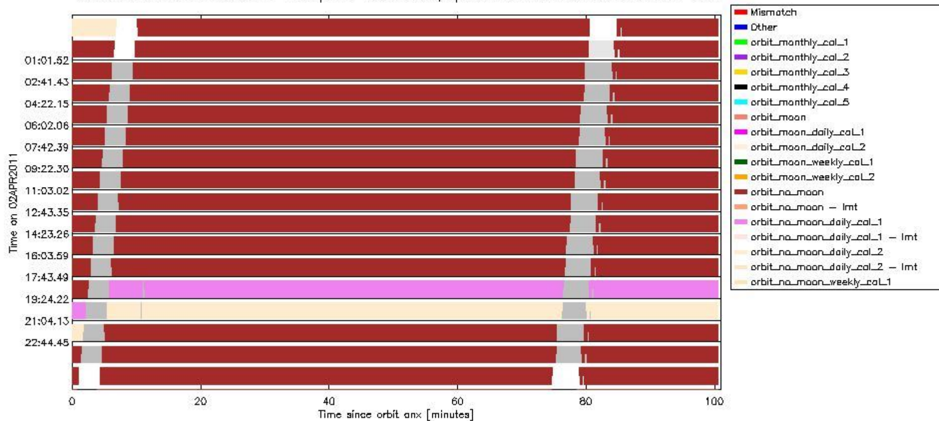
sciamachy_daily_report_level0_KSPT_L0_4504_N_20110402_6.PNG
