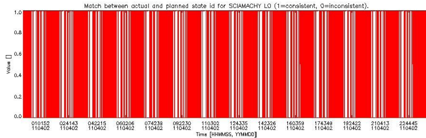
sciamachy_daily_report_level0_KSPT_L0_4504_N_20110402_5.PNG
