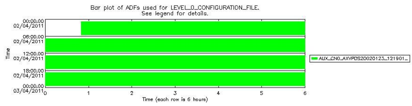
sciamachy_daily_report_level0_KSPT_L0_4504_N_20110402_7.PNG
