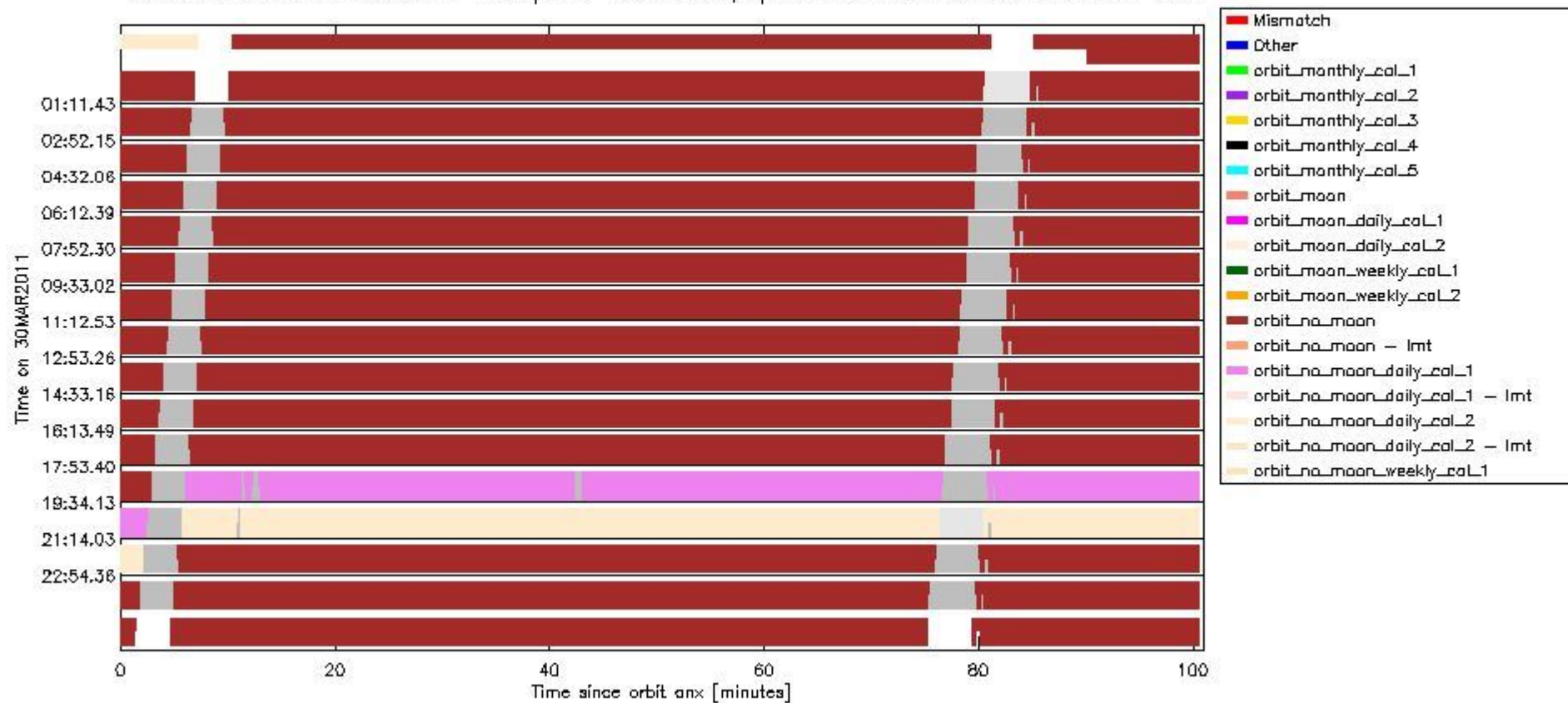
sciamachy_daily_report_level0_KSPT_L0_4504_N_20110330_6.PNG
