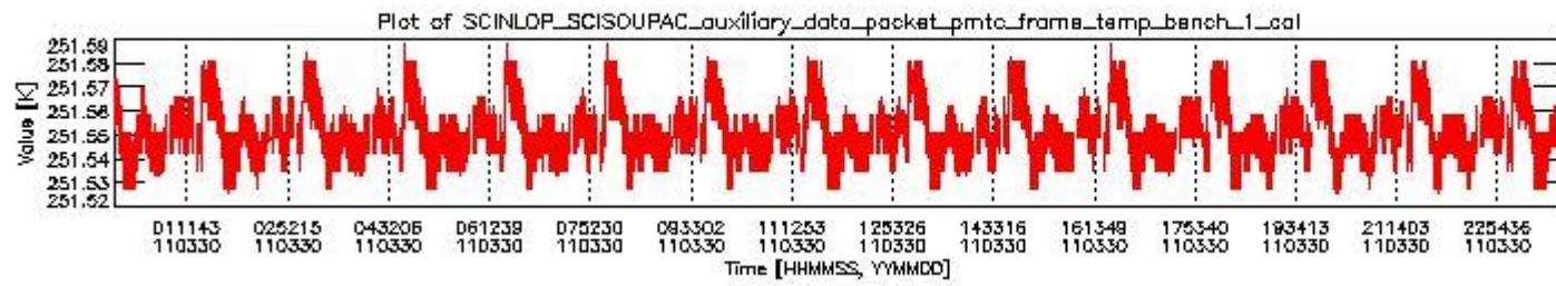
sciamachy_daily_report_level0_KSPT_L0_4504_N_20110330_0.PNG
