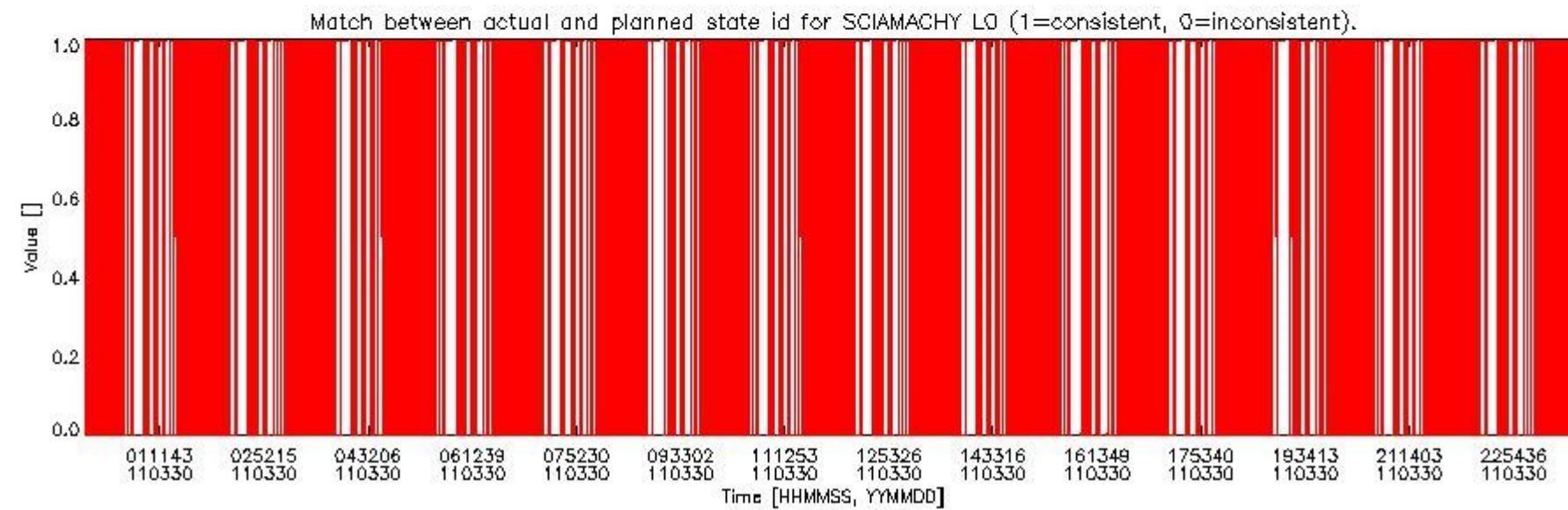
sciamachy_daily_report_level0_KSPT_L0_4504_N_20110330_5.PNG
