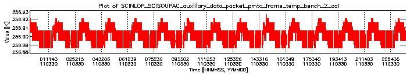
sciamachy_daily_report_level0_KSPT_L0_4504_N_20110330_1.PNG
