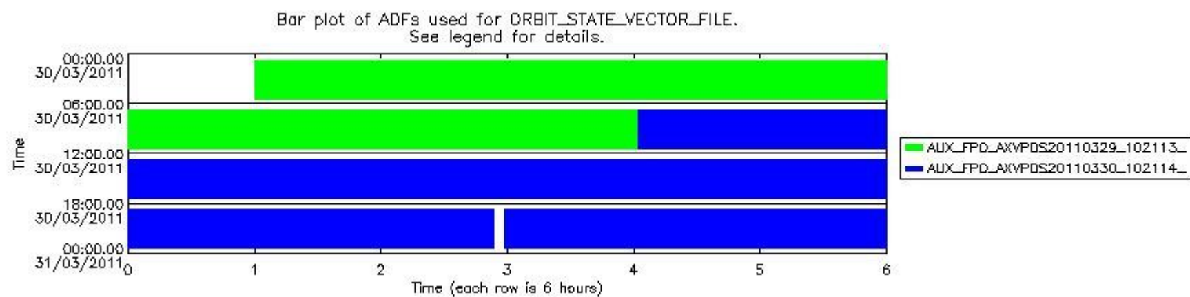
sciamachy_daily_report_level0_KSPT_L0_4504_N_20110330_8.PNG
