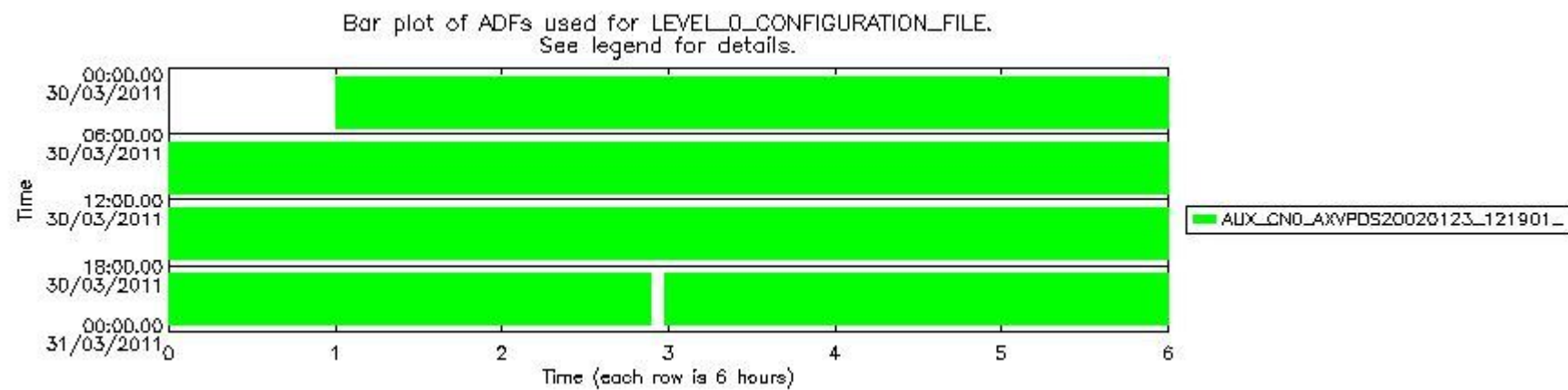
sciamachy_daily_report_level0_KSPT_L0_4504_N_20110330_7.PNG
