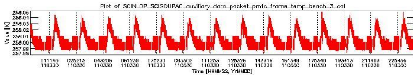
sciamachy_daily_report_level0_KSPT_L0_4504_N_20110330_2.PNG
