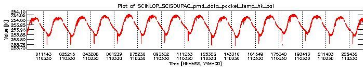
sciamachy_daily_report_level0_KSPT_L0_4504_N_20110330_3.PNG
