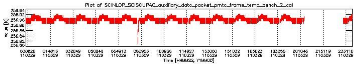
sciamachy_daily_report_level0_KSPT_L0_4504_N_20110329_1.PNG
