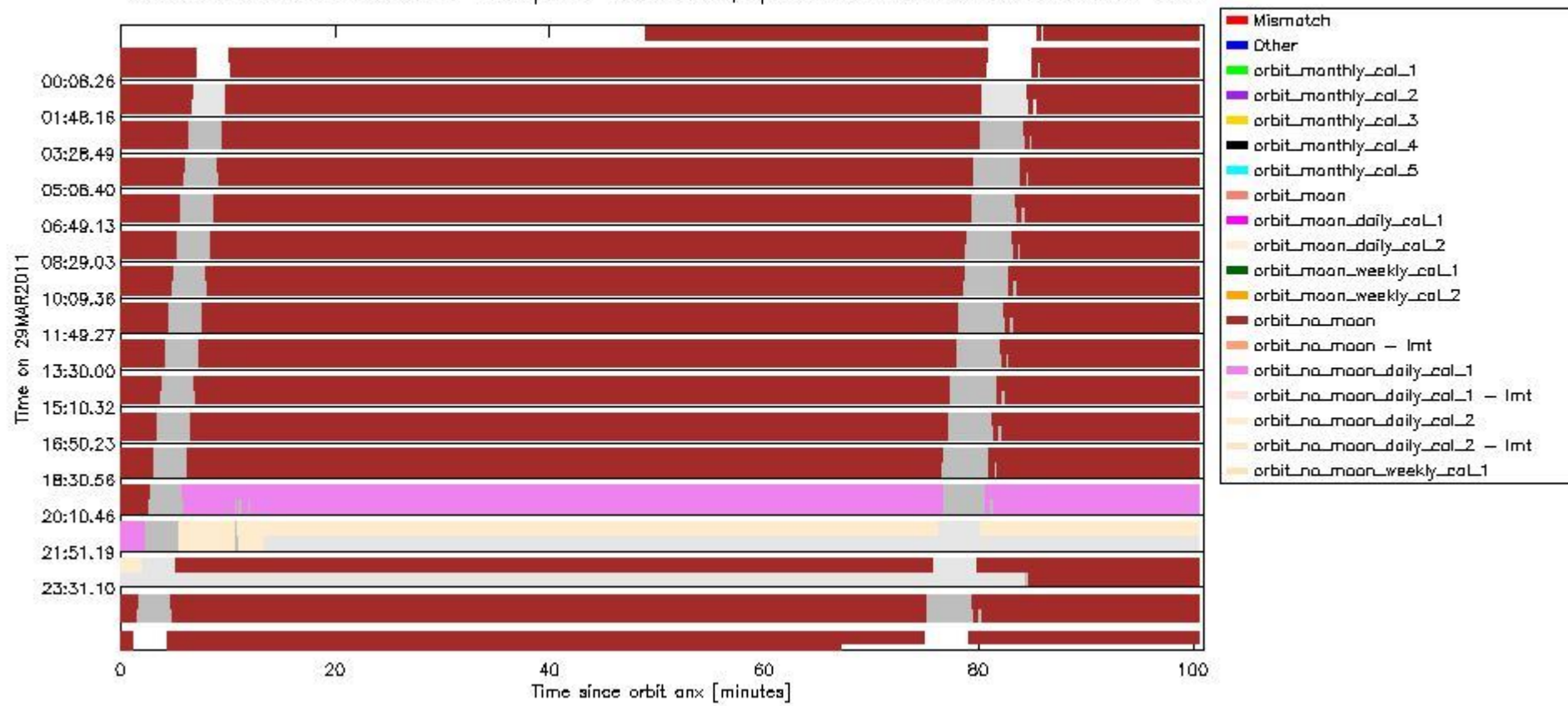
sciamachy_daily_report_level0_KSPT_L0_4504_N_20110329_6.PNG
