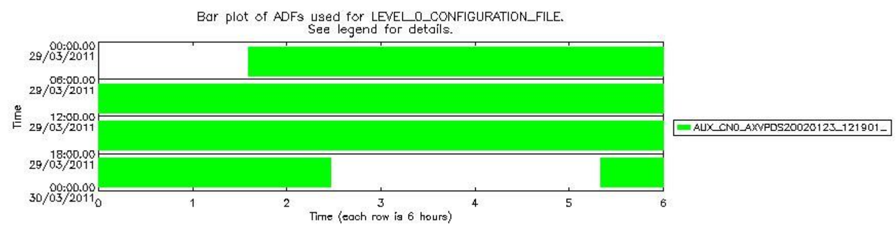
sciamachy_daily_report_level0_KSPT_L0_4504_N_20110329_7.PNG
