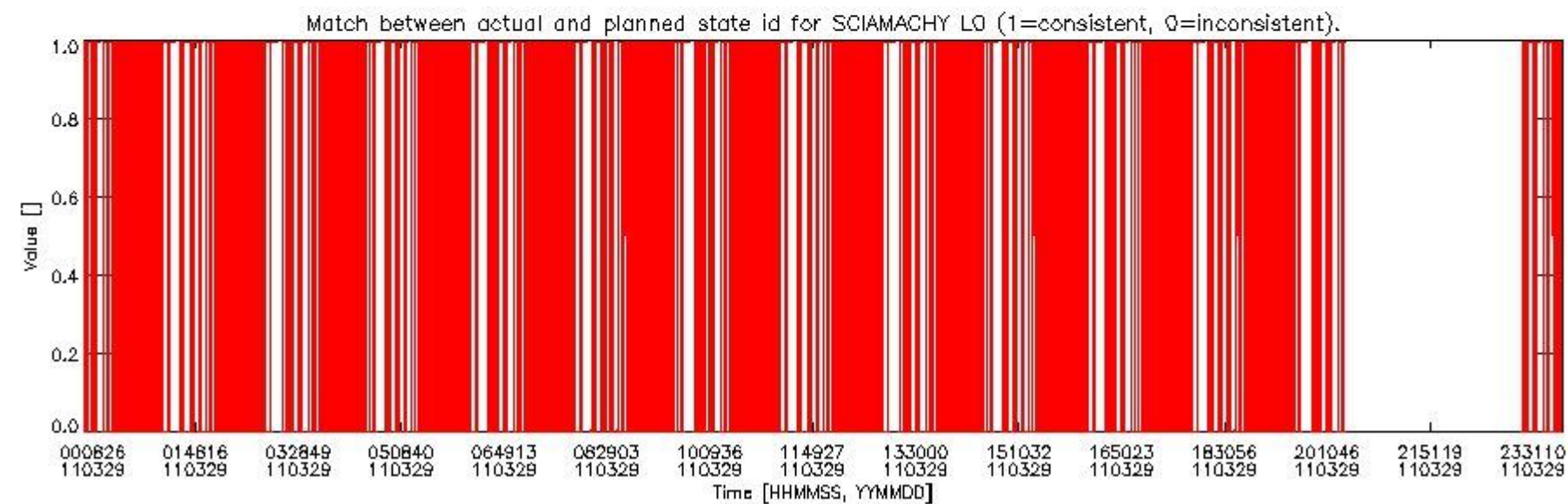
sciamachy_daily_report_level0_KSPT_L0_4504_N_20110329_5.PNG
