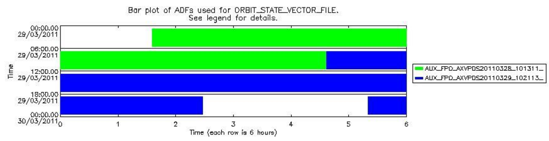
sciamachy_daily_report_level0_KSPT_L0_4504_N_20110329_8.PNG
