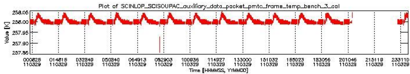
sciamachy_daily_report_level0_KSPT_L0_4504_N_20110329_2.PNG
