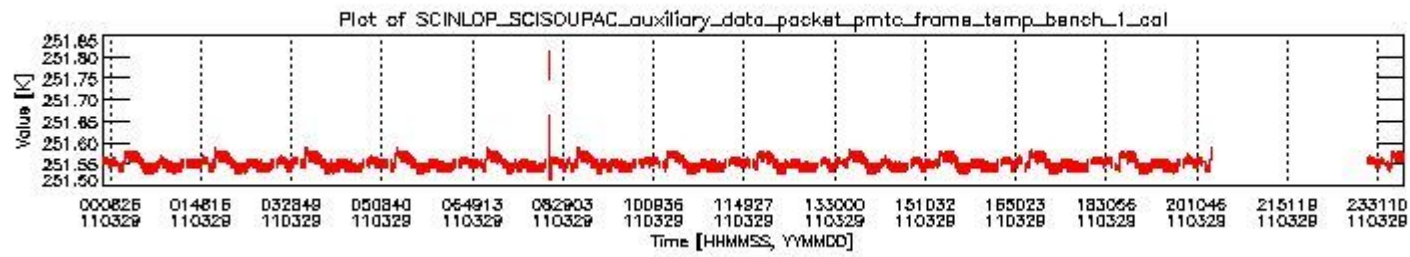
sciamachy_daily_report_level0_KSPT_L0_4504_N_20110329_0.PNG
