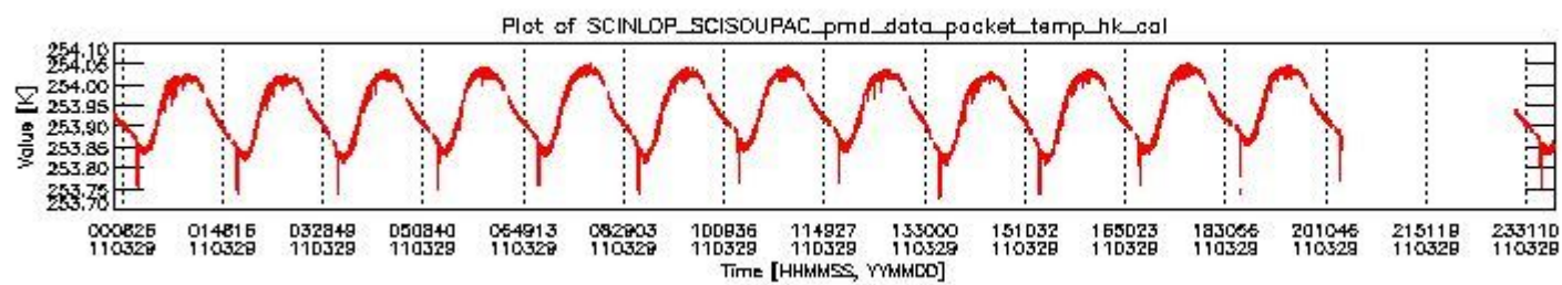
sciamachy_daily_report_level0_KSPT_L0_4504_N_20110329_3.PNG
