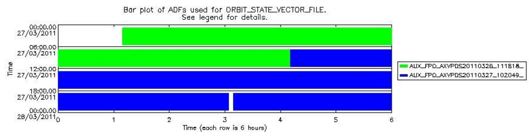
sciamachy_daily_report_level0_KSPT_L0_4504_N_20110327_8.PNG
