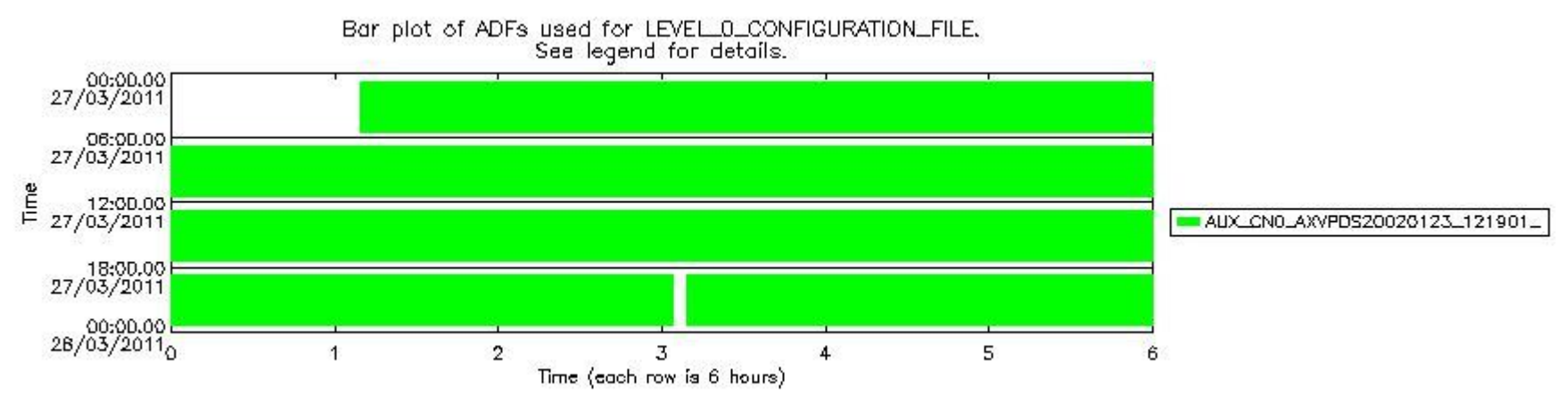
sciamachy_daily_report_level0_KSPT_L0_4504_N_20110327_7.PNG
