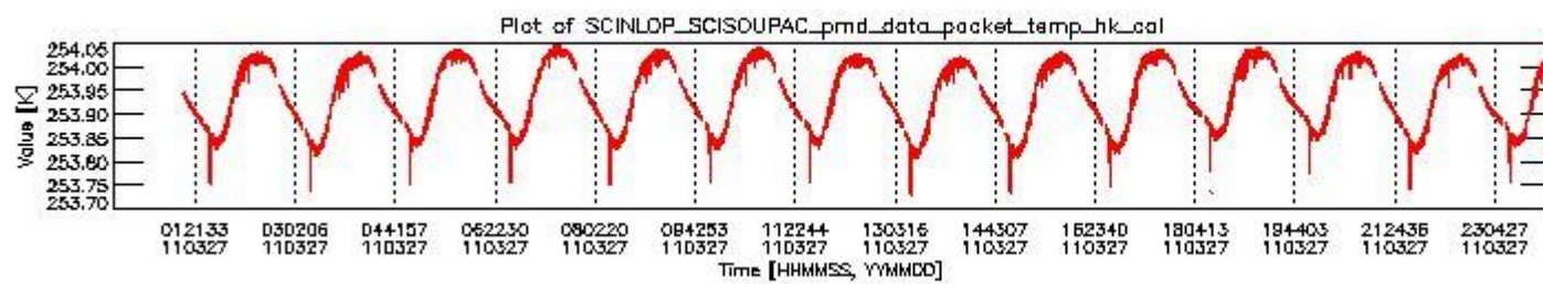
sciamachy_daily_report_level0_KSPT_L0_4504_N_20110327_3.PNG
