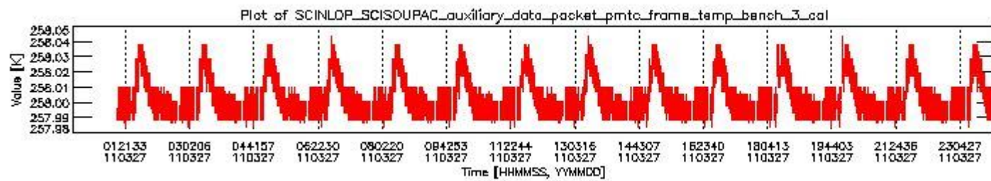
sciamachy_daily_report_level0_KSPT_L0_4504_N_20110327_2.PNG
