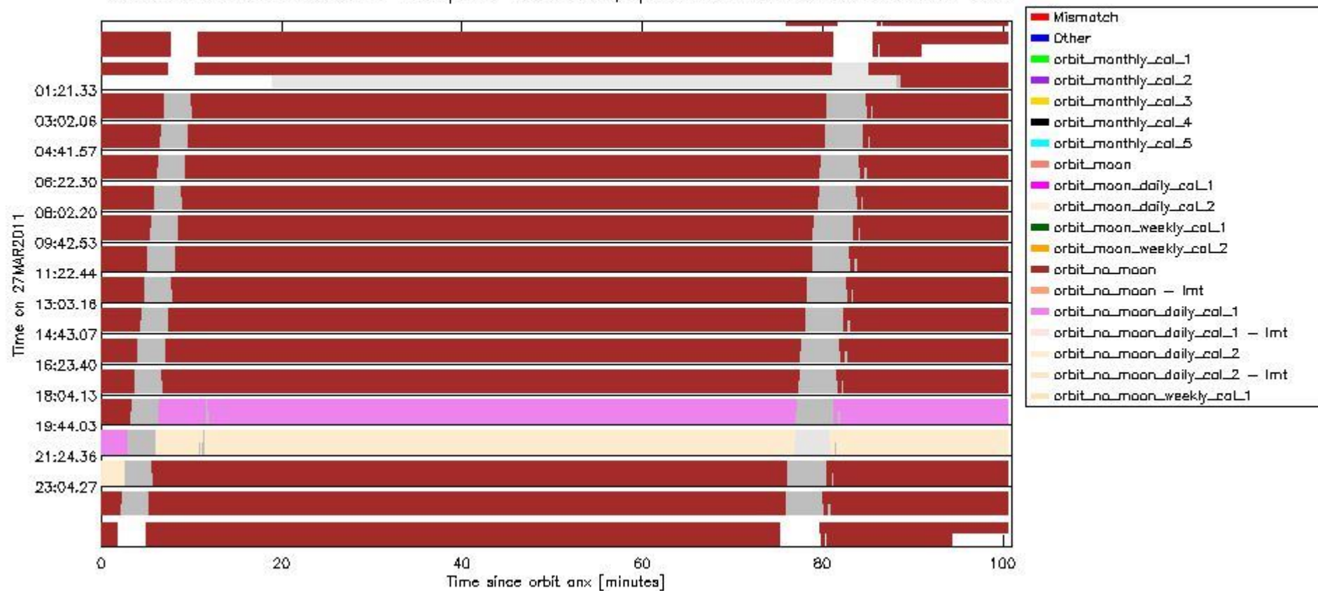
sciamachy_daily_report_level0_KSPT_L0_4504_N_20110327_6.PNG
