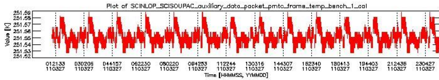
sciamachy_daily_report_level0_KSPT_L0_4504_N_20110327_0.PNG
