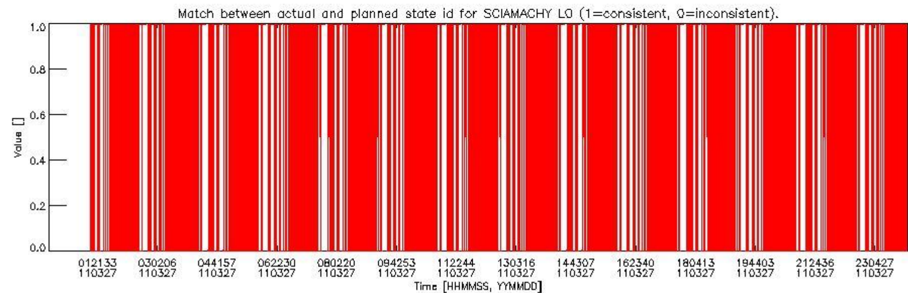
sciamachy_daily_report_level0_KSPT_L0_4504_N_20110327_5.PNG
