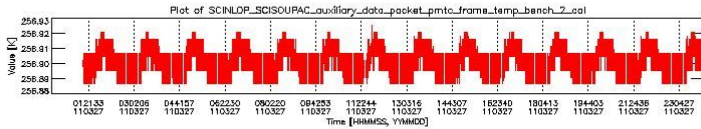
sciamachy_daily_report_level0_KSPT_L0_4504_N_20110327_1.PNG
