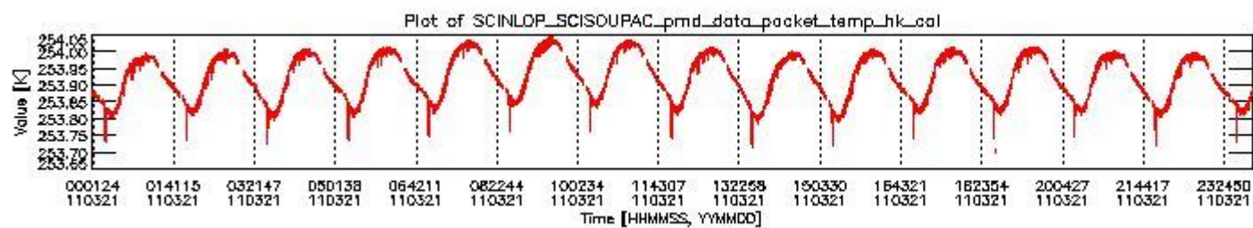
sciamachy_daily_report_level0_KSPT_L0_4504_N_20110321_3.PNG
