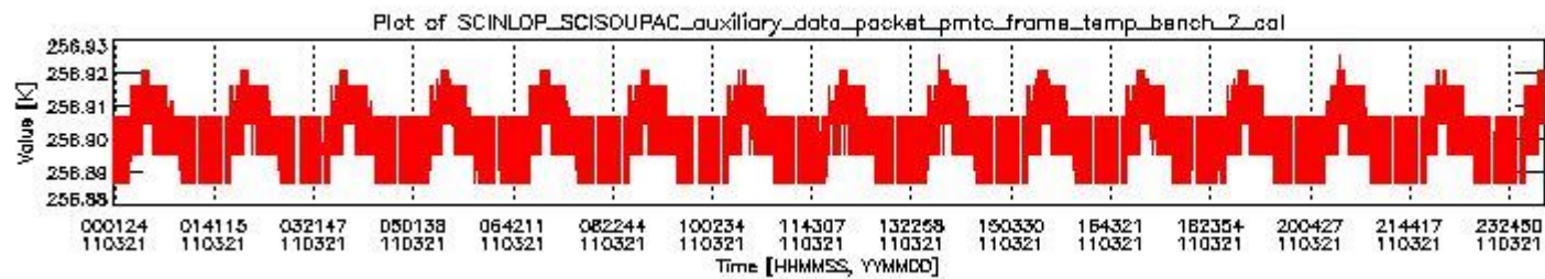
sciamachy_daily_report_level0_KSPT_L0_4504_N_20110321_1.PNG
