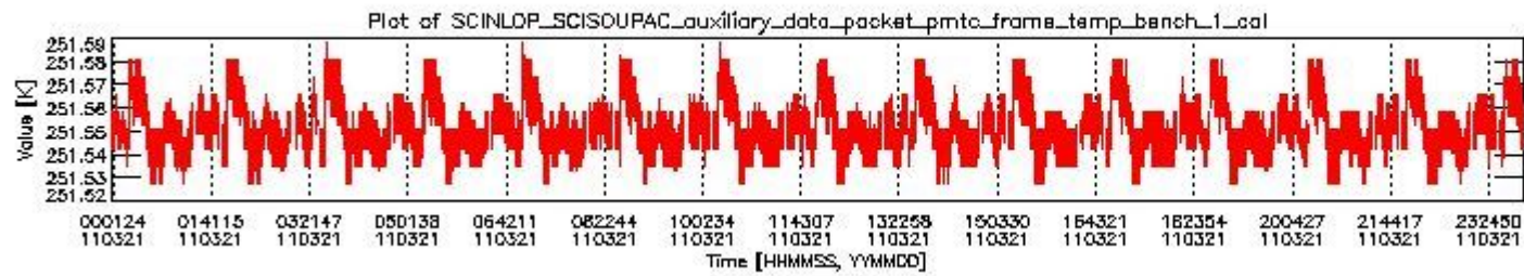
sciamachy_daily_report_level0_KSPT_L0_4504_N_20110321_0.PNG
