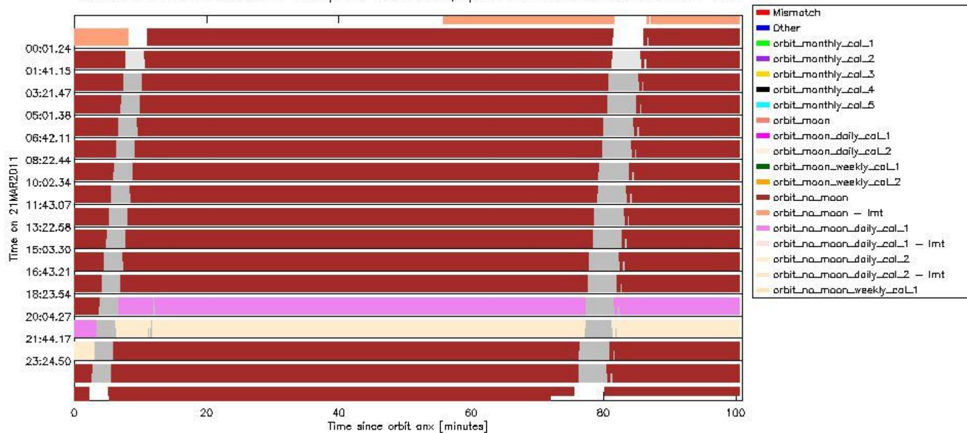
sciamachy_daily_report_level0_KSPT_L0_4504_N_20110321_6.PNG
