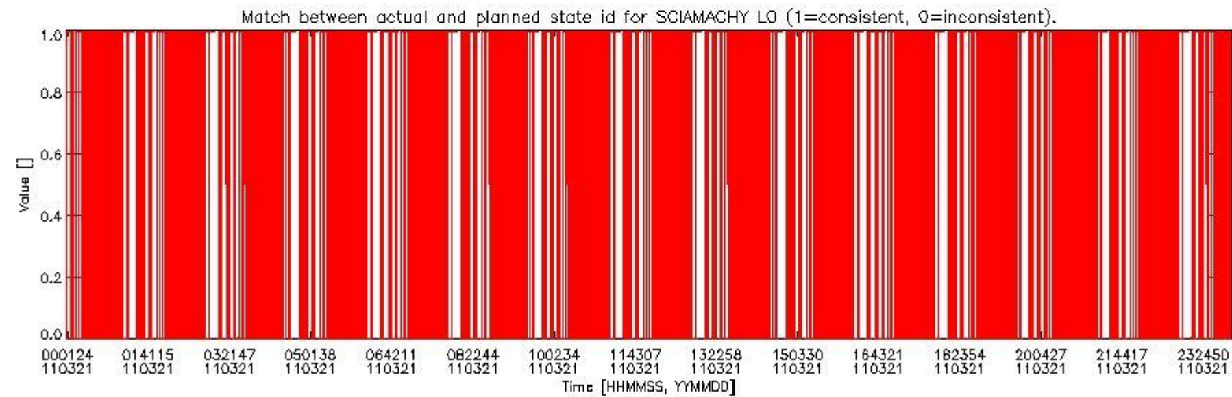
sciamachy_daily_report_level0_KSPT_L0_4504_N_20110321_5.PNG
