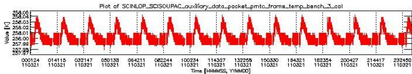
sciamachy_daily_report_level0_KSPT_L0_4504_N_20110321_2.PNG
