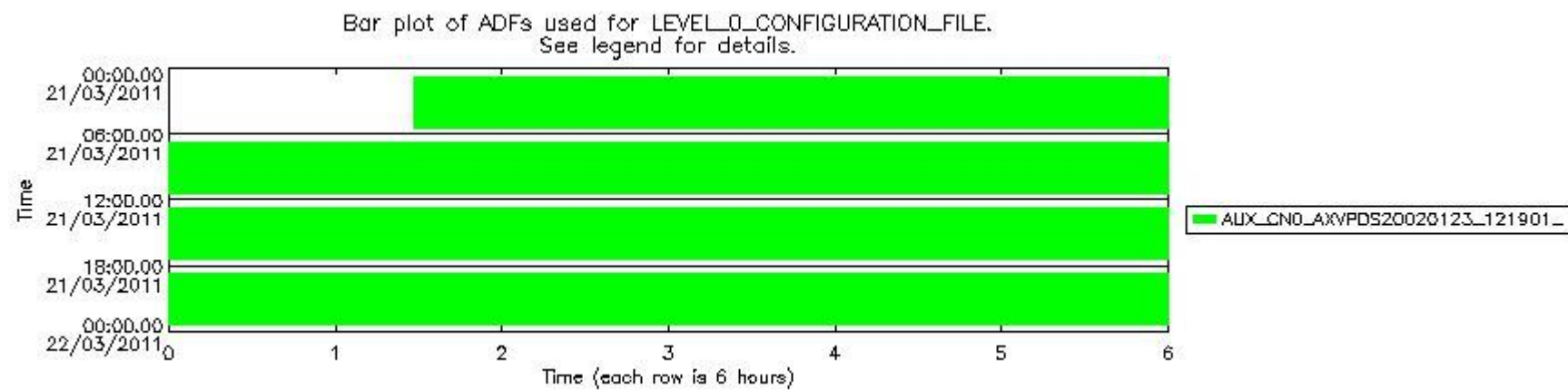
sciamachy_daily_report_level0_KSPT_L0_4504_N_20110321_7.PNG
