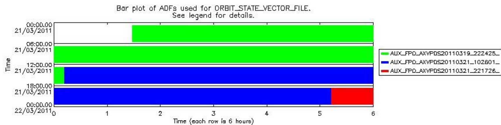
sciamachy_daily_report_level0_KSPT_L0_4504_N_20110321_8.PNG
