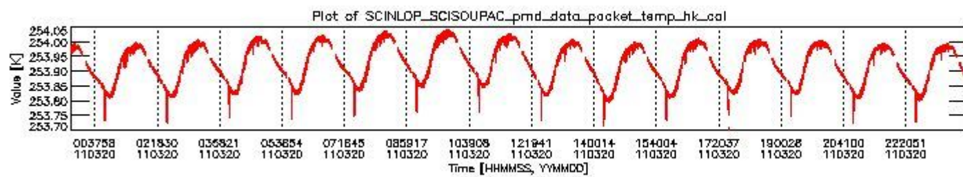
sciamachy_daily_report_level0_KSPT_L0_4504_N_20110320_3.PNG
