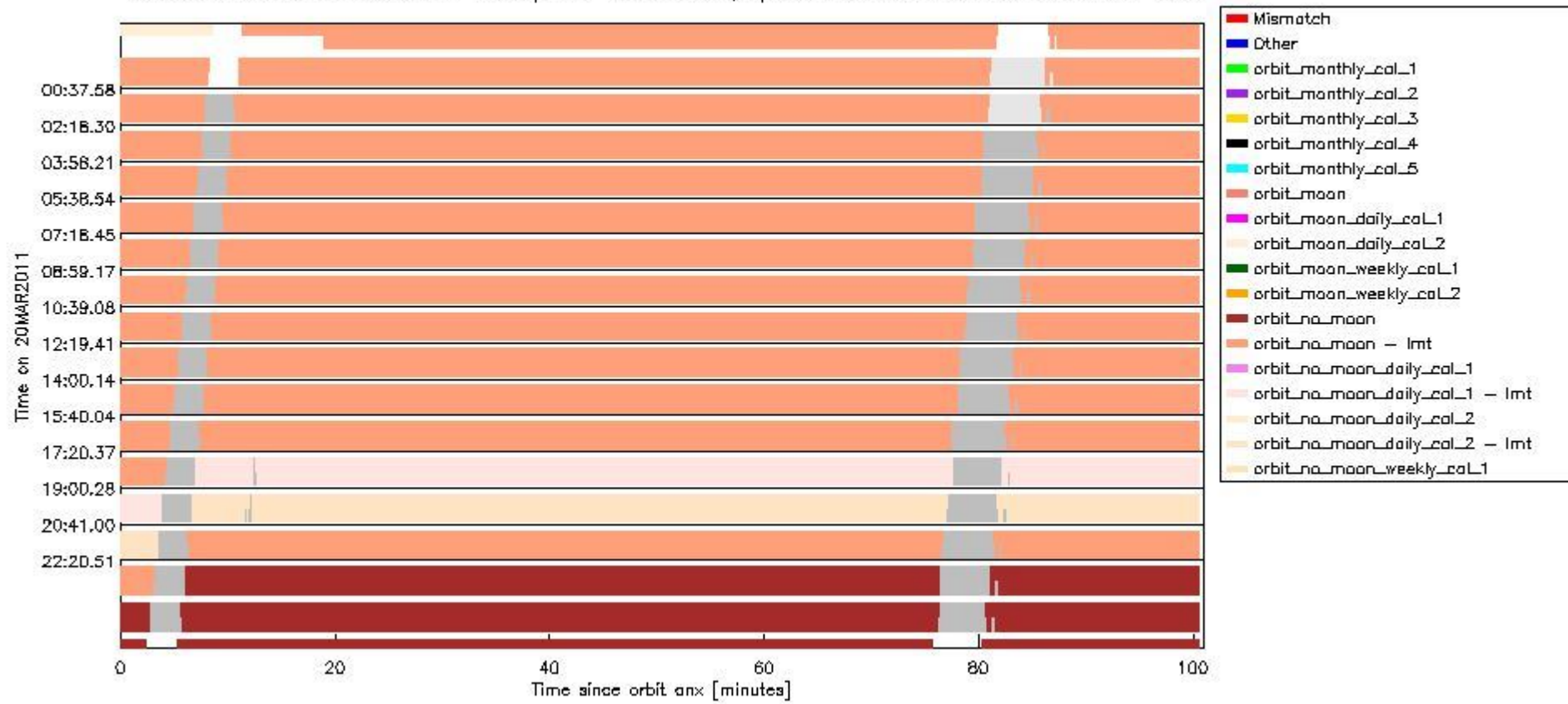
sciamachy_daily_report_level0_KSPT_L0_4504_N_20110320_6.PNG
