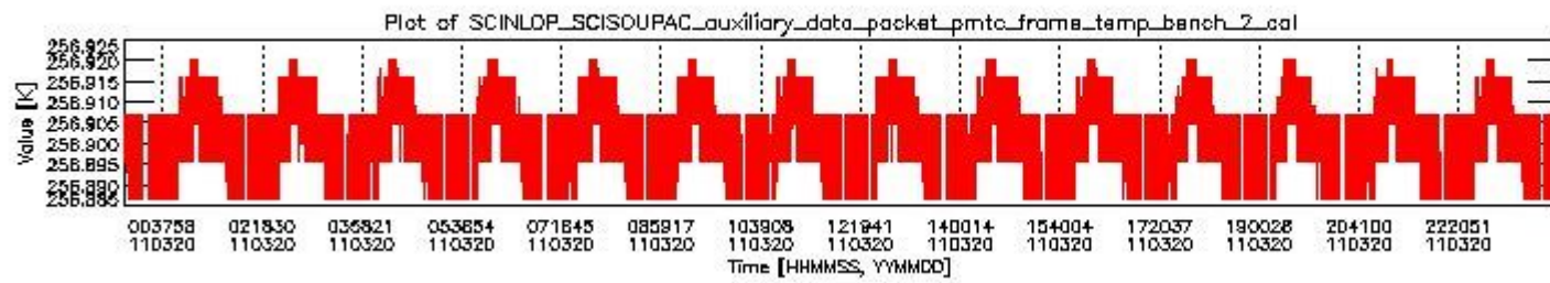
sciamachy_daily_report_level0_KSPT_L0_4504_N_20110320_1.PNG
