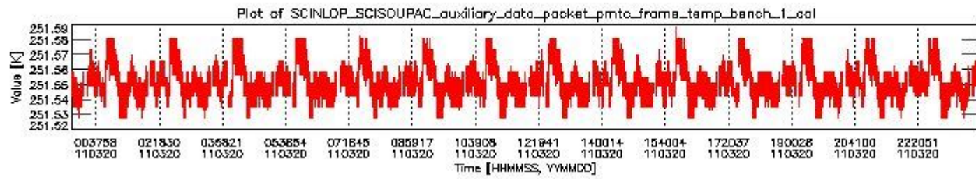
sciamachy_daily_report_level0_KSPT_L0_4504_N_20110320_0.PNG
