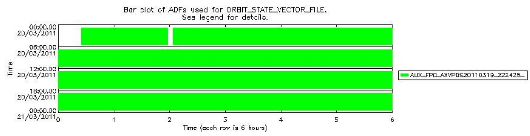
sciamachy_daily_report_level0_KSPT_L0_4504_N_20110320_8.PNG
