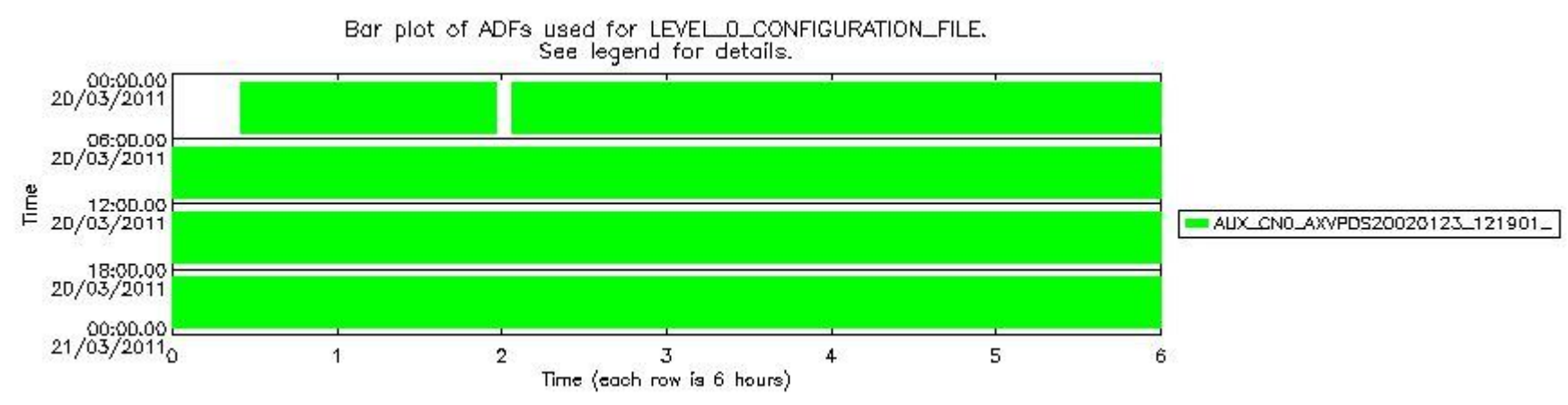
sciamachy_daily_report_level0_KSPT_L0_4504_N_20110320_7.PNG
