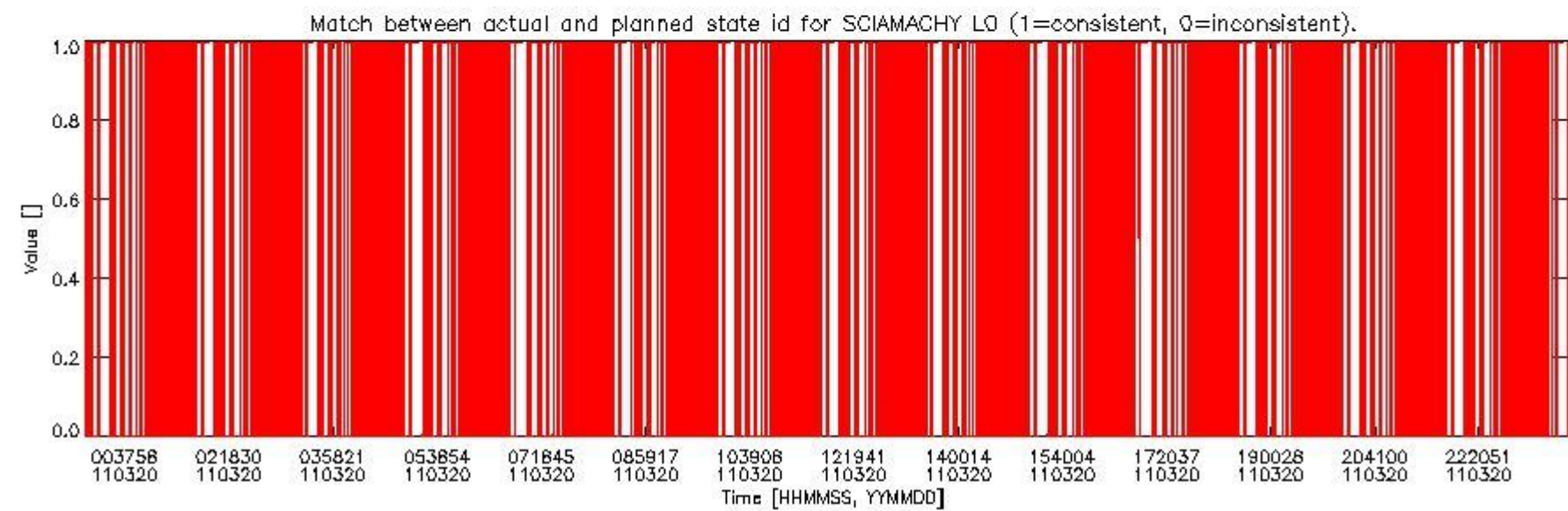
sciamachy_daily_report_level0_KSPT_L0_4504_N_20110320_5.PNG
