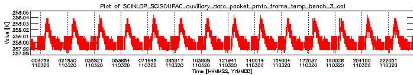
sciamachy_daily_report_level0_KSPT_L0_4504_N_20110320_2.PNG
