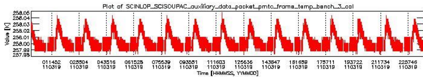
sciamachy_daily_report_level0_KSPT_L0_4504_N_20110319_2.PNG
