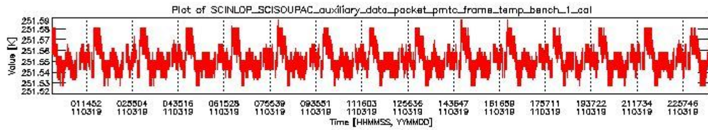
sciamachy_daily_report_level0_KSPT_L0_4504_N_20110319_0.PNG
