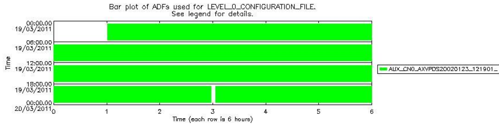
sciamachy_daily_report_level0_KSPT_L0_4504_N_20110319_7.PNG
