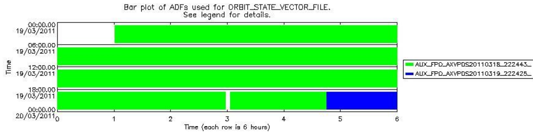
sciamachy_daily_report_level0_KSPT_L0_4504_N_20110319_8.PNG
