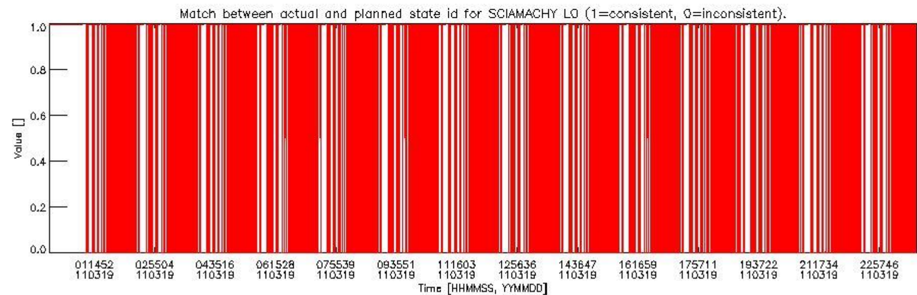
sciamachy_daily_report_level0_KSPT_L0_4504_N_20110319_5.PNG
