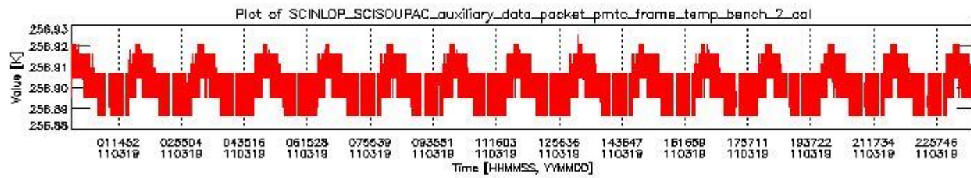
sciamachy_daily_report_level0_KSPT_L0_4504_N_20110319_1.PNG
