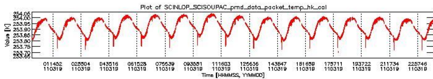
sciamachy_daily_report_level0_KSPT_L0_4504_N_20110319_3.PNG
