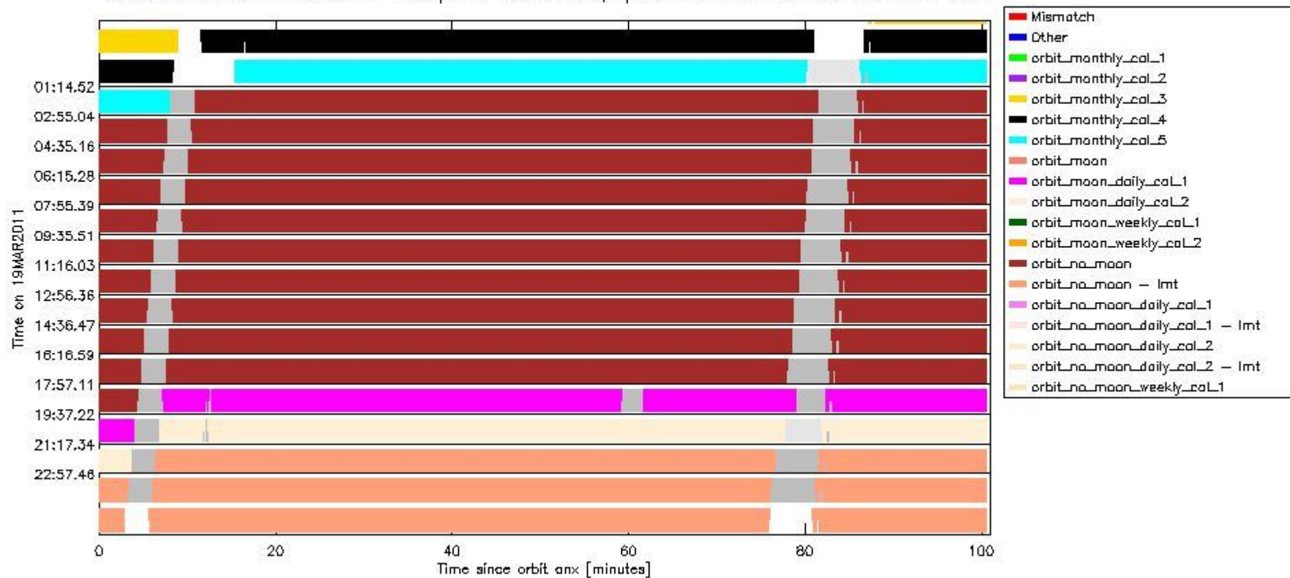
sciamachy_daily_report_level0_KSPT_L0_4504_N_20110319_6.PNG
