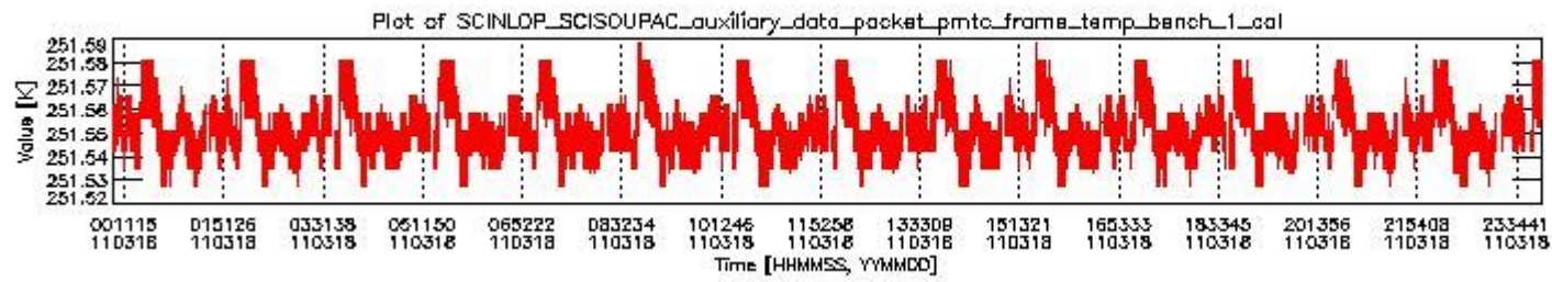
sciamachy_daily_report_level0_KSPT_L0_4504_N_20110318_0.PNG
