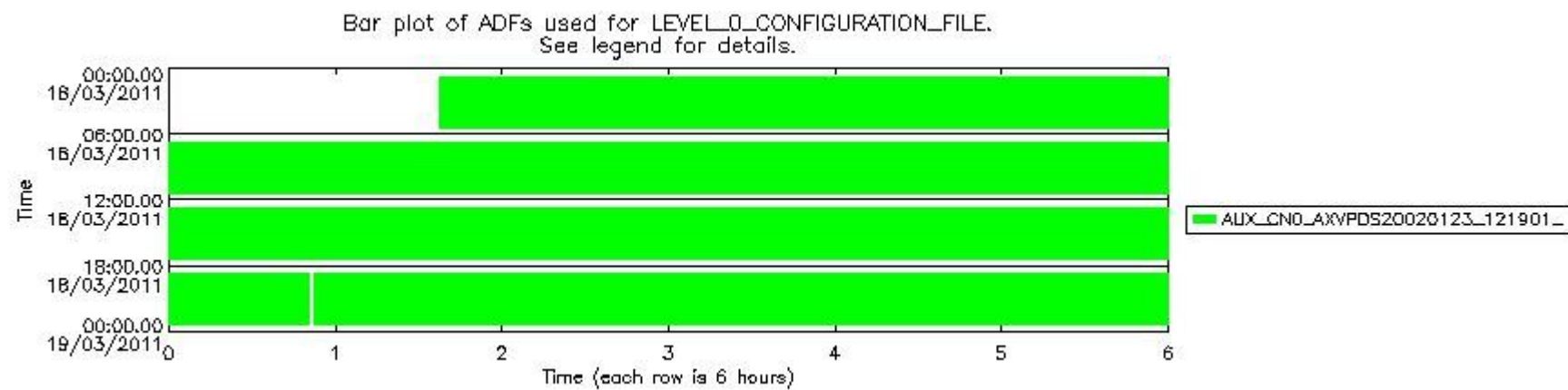
sciamachy_daily_report_level0_KSPT_L0_4504_N_20110318_7.PNG
