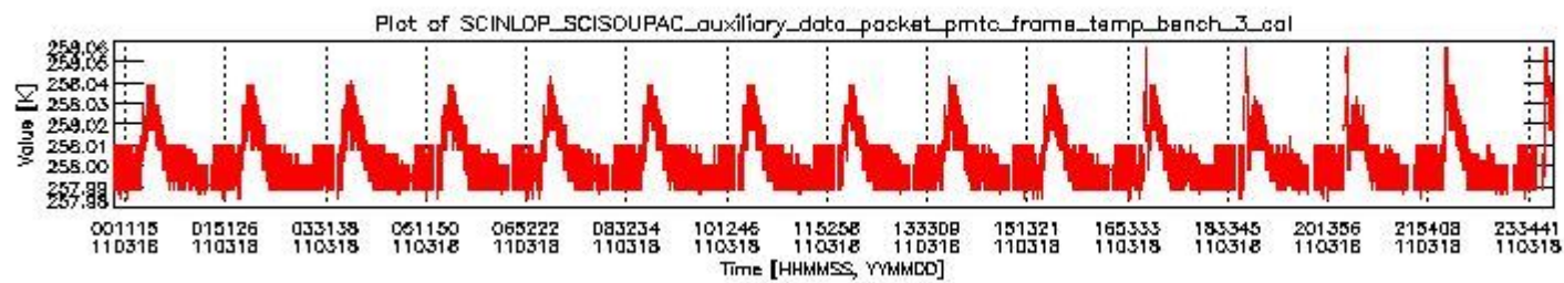
sciamachy_daily_report_level0_KSPT_L0_4504_N_20110318_2.PNG
