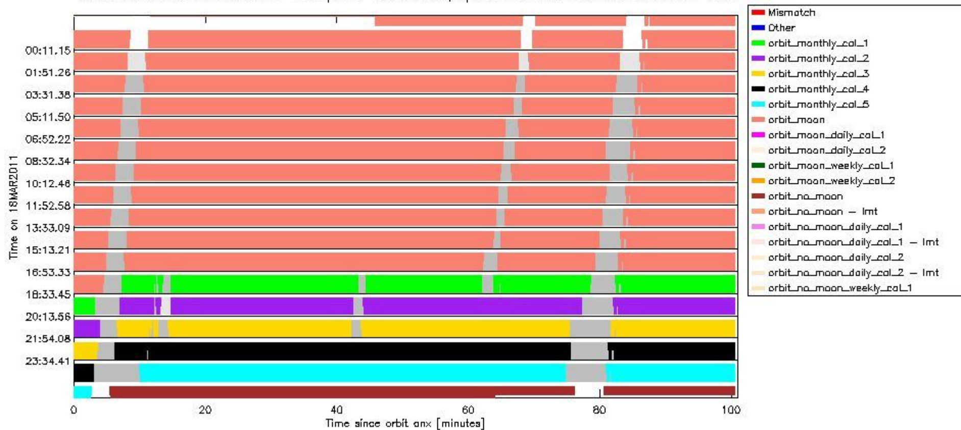
sciamachy_daily_report_level0_KSPT_L0_4504_N_20110318_6.PNG
