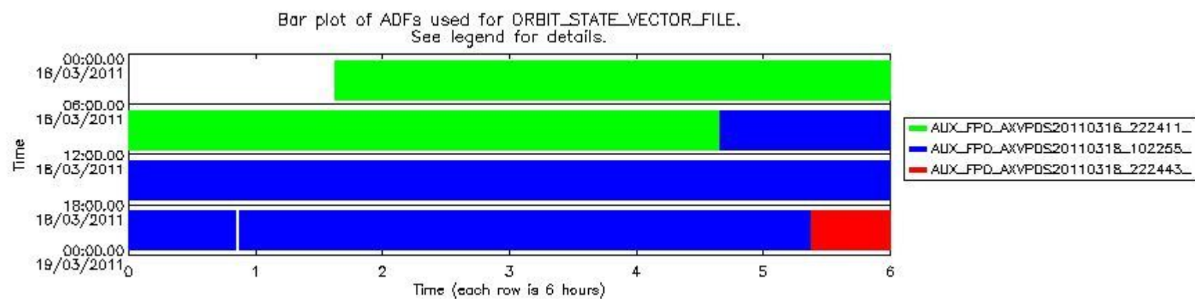
sciamachy_daily_report_level0_KSPT_L0_4504_N_20110318_8.PNG
