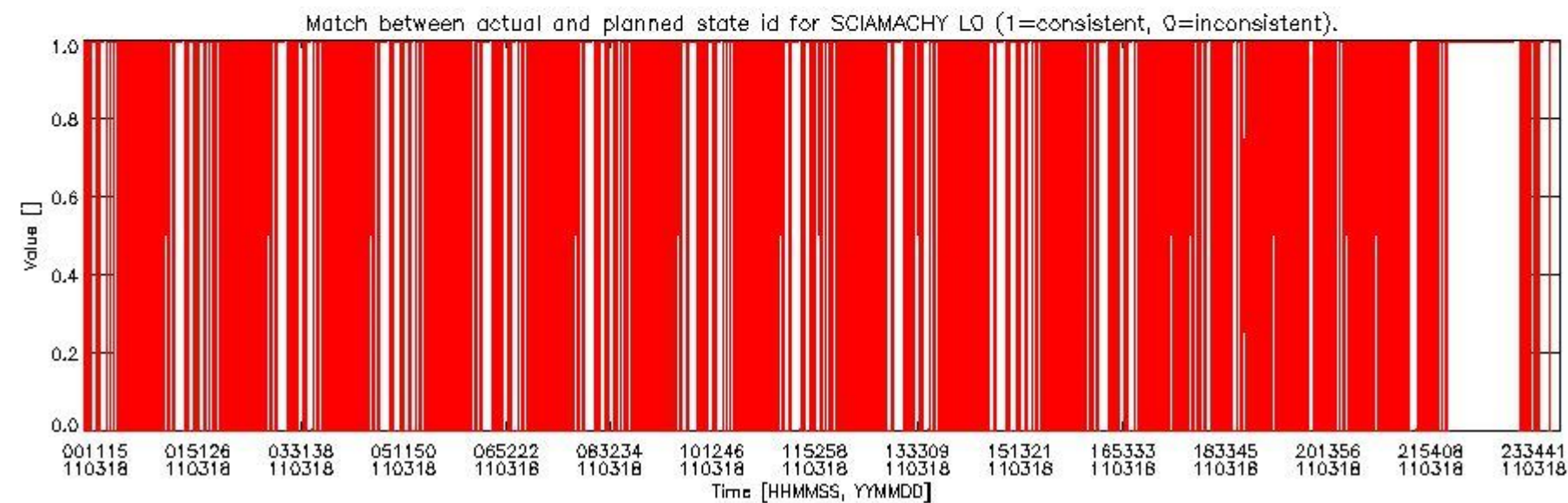
sciamachy_daily_report_level0_KSPT_L0_4504_N_20110318_5.PNG
