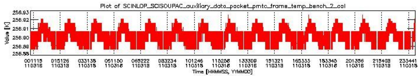
sciamachy_daily_report_level0_KSPT_L0_4504_N_20110318_1.PNG
