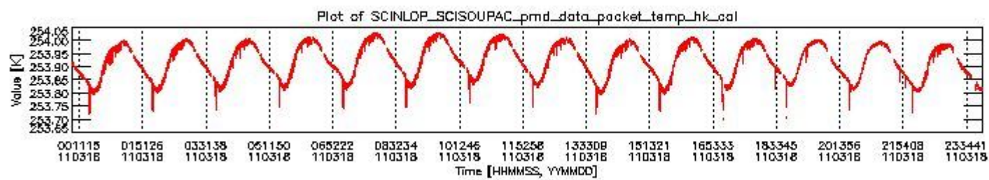
sciamachy_daily_report_level0_KSPT_L0_4504_N_20110318_3.PNG
