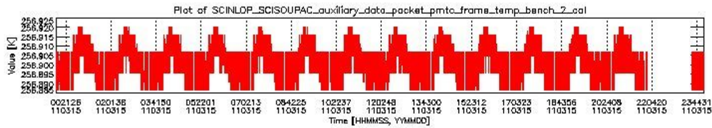
sciamachy_daily_report_level0_KSPT_L0_4504_N_20110315_1.PNG
