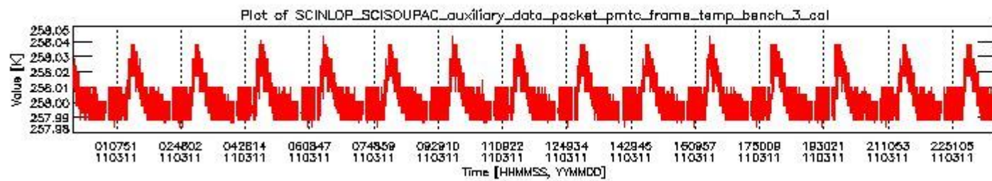
sciamachy_daily_report_level0_KSPT_L0_4504_N_20110311_2.PNG
