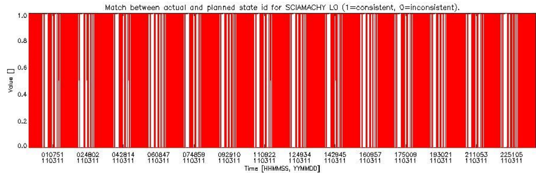
sciamachy_daily_report_level0_KSPT_L0_4504_N_20110311_5.PNG
