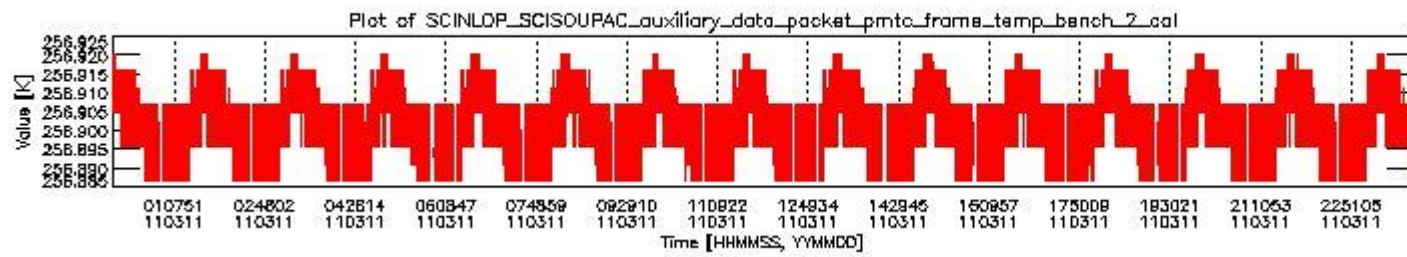
sciamachy_daily_report_level0_KSPT_L0_4504_N_20110311_1.PNG
