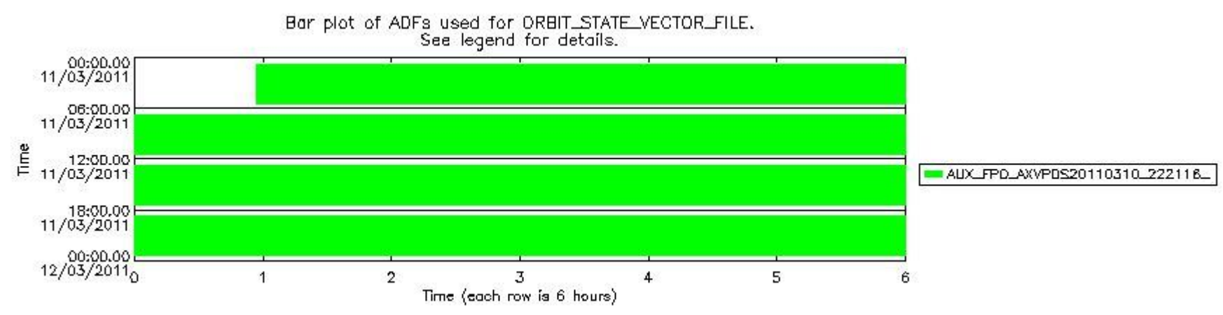
sciamachy_daily_report_level0_KSPT_L0_4504_N_20110311_8.PNG
