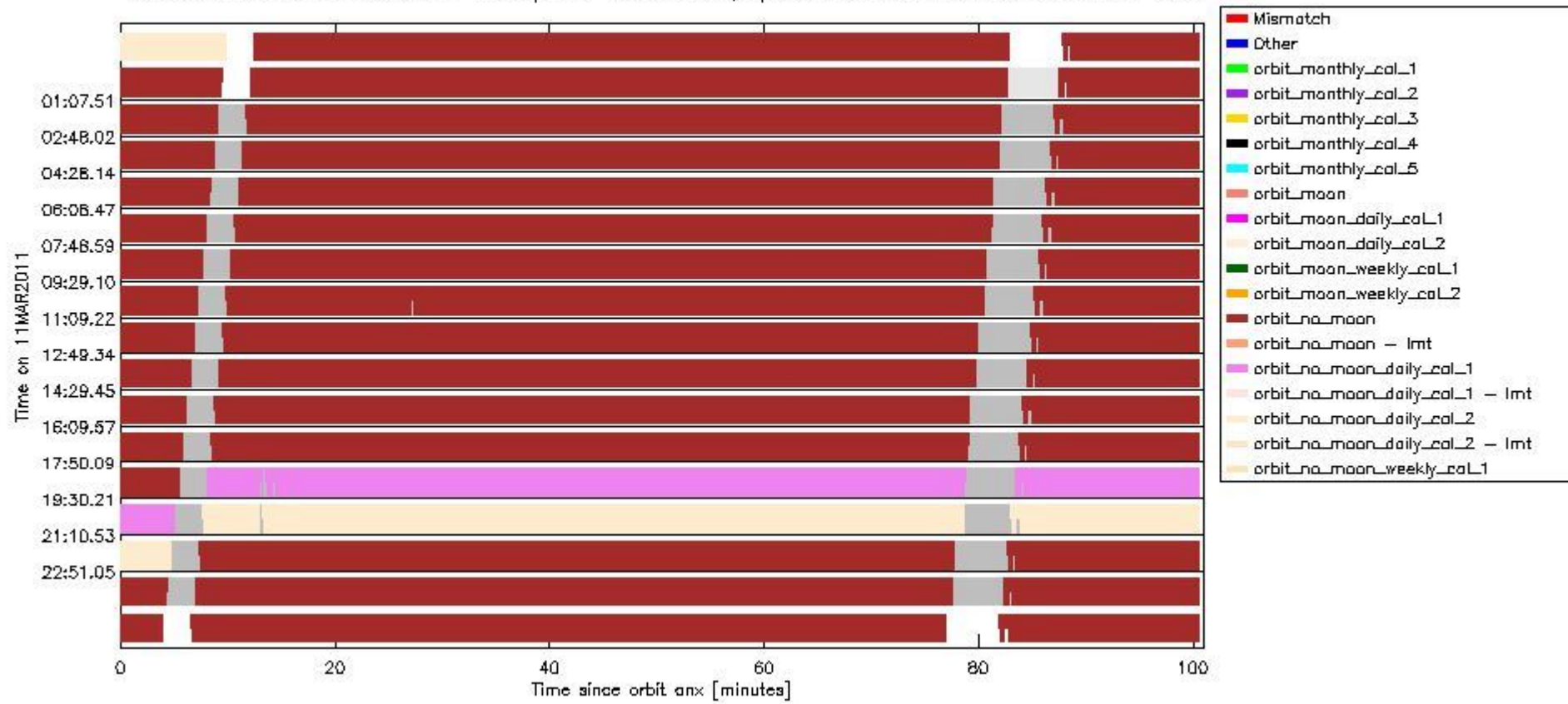
sciamachy_daily_report_level0_KSPT_L0_4504_N_20110311_6.PNG
