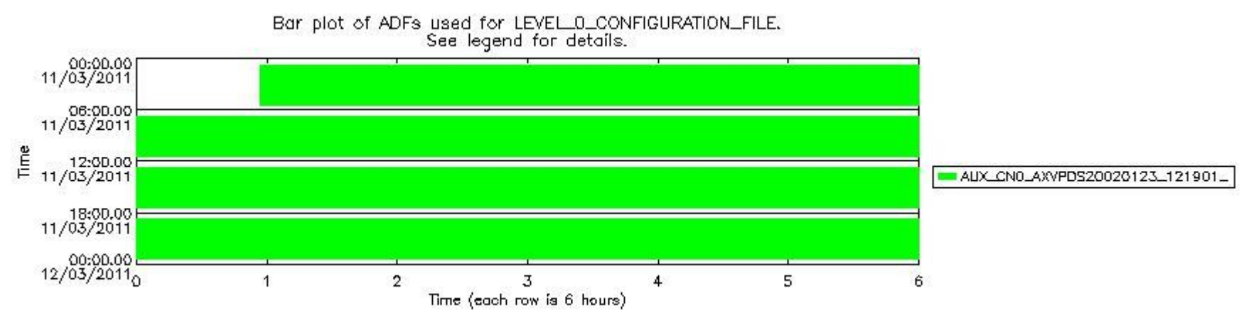
sciamachy_daily_report_level0_KSPT_L0_4504_N_20110311_7.PNG
