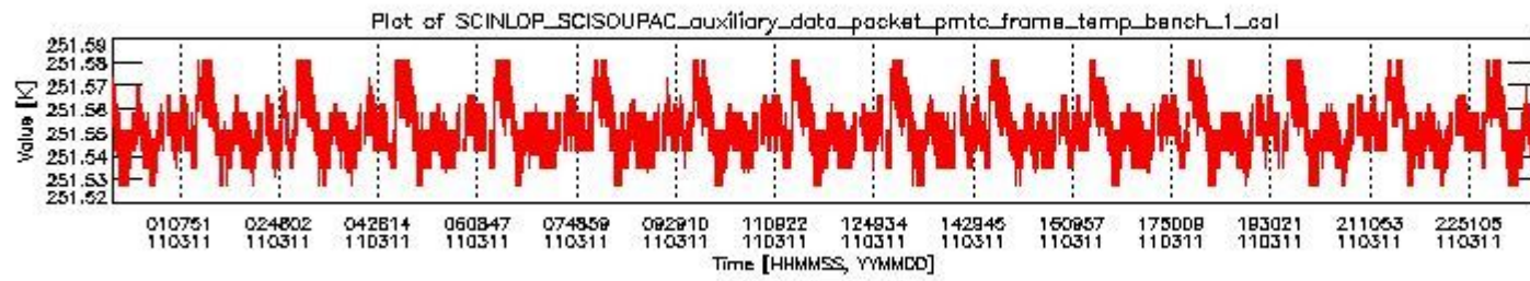
sciamachy_daily_report_level0_KSPT_L0_4504_N_20110311_0.PNG
