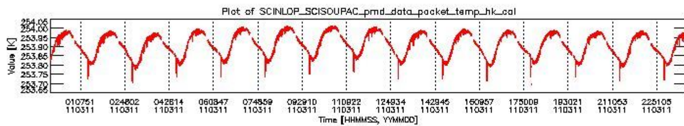
sciamachy_daily_report_level0_KSPT_L0_4504_N_20110311_3.PNG
