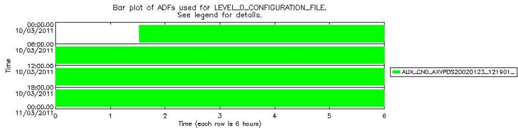
sciamachy_daily_report_level0_KSPT_L0_4504_N_20110310_7.PNG
