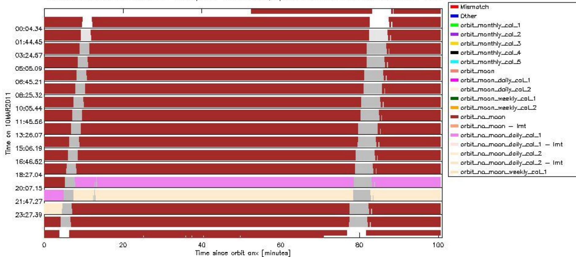
sciamachy_daily_report_level0_KSPT_L0_4504_N_20110310_6.PNG
