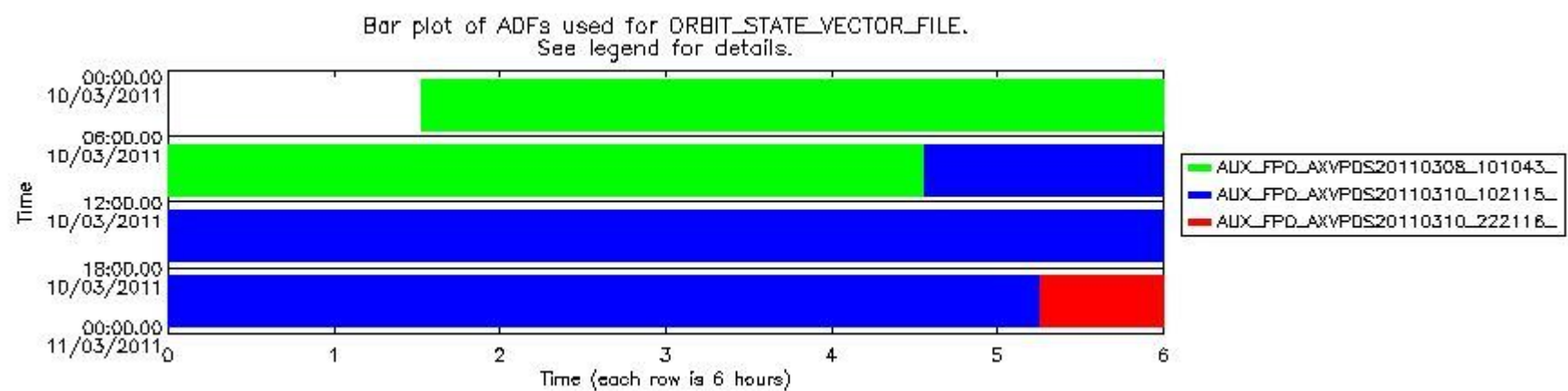
sciamachy_daily_report_level0_KSPT_L0_4504_N_20110310_8.PNG
