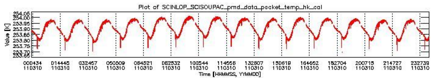
sciamachy_daily_report_level0_KSPT_L0_4504_N_20110310_3.PNG
