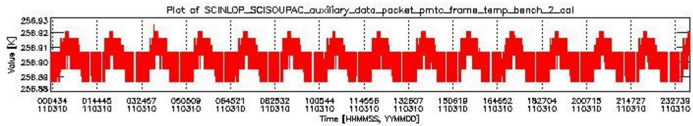
sciamachy_daily_report_level0_KSPT_L0_4504_N_20110310_1.PNG
