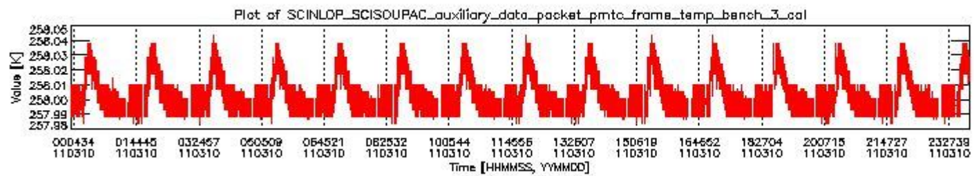
sciamachy_daily_report_level0_KSPT_L0_4504_N_20110310_2.PNG
