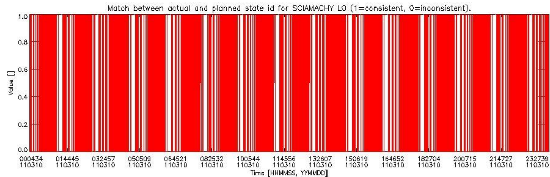
sciamachy_daily_report_level0_KSPT_L0_4504_N_20110310_5.PNG
