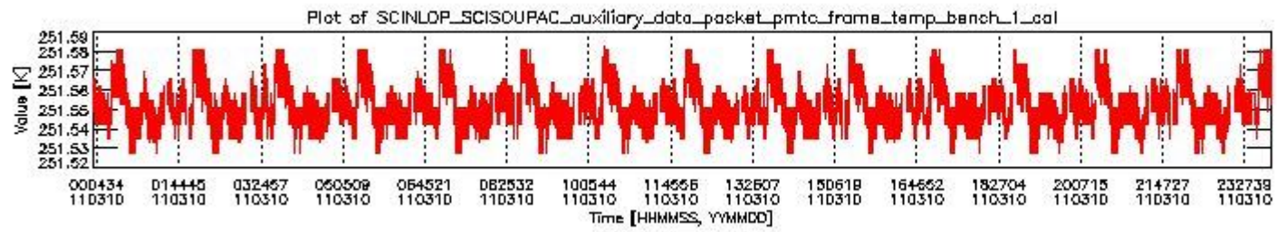
sciamachy_daily_report_level0_KSPT_L0_4504_N_20110310_0.PNG
