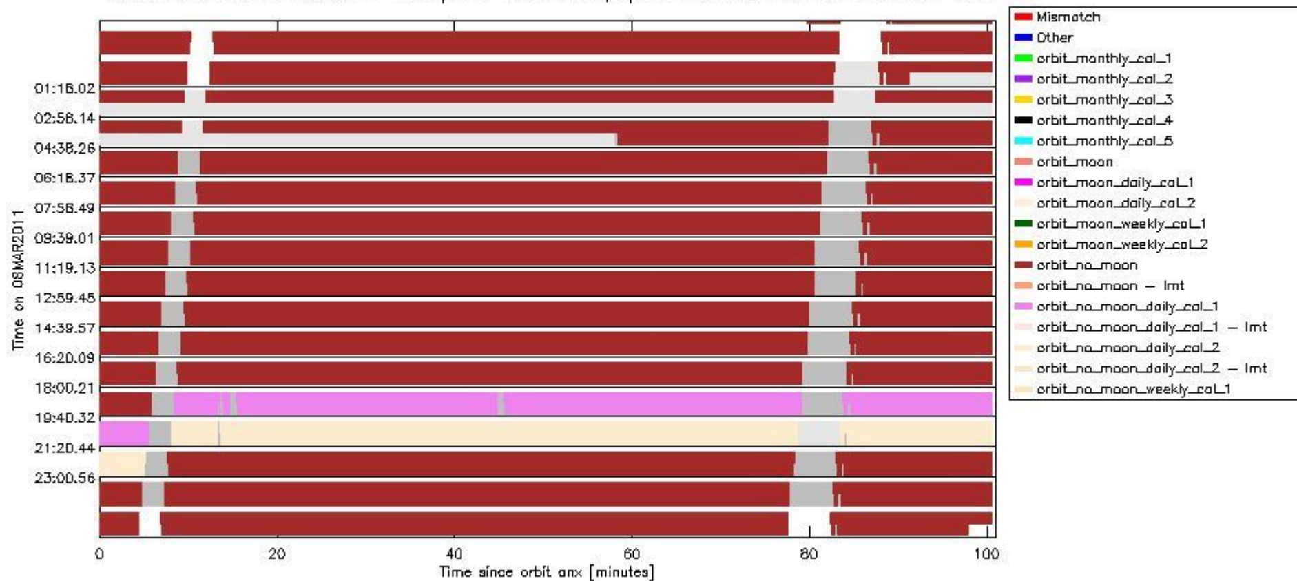
sciamachy_daily_report_level0_KSPT_L0_4504_N_20110308_6.PNG
