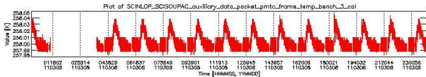
sciamachy_daily_report_level0_KSPT_L0_4504_N_20110308_2.PNG
