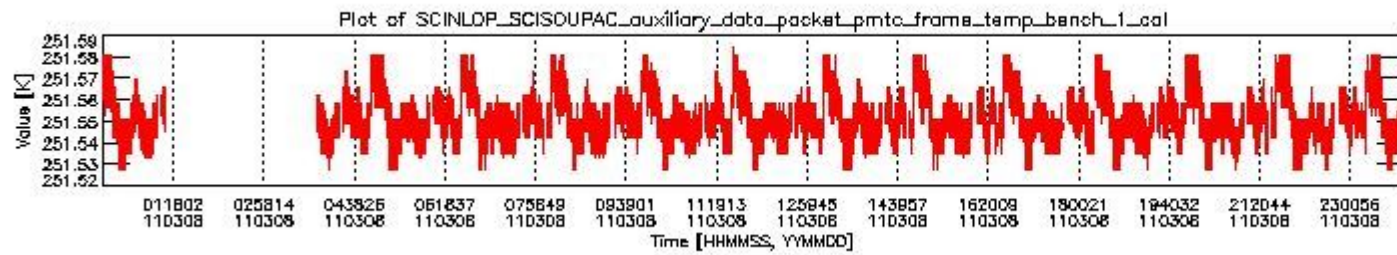
sciamachy_daily_report_level0_KSPT_L0_4504_N_20110308_0.PNG
