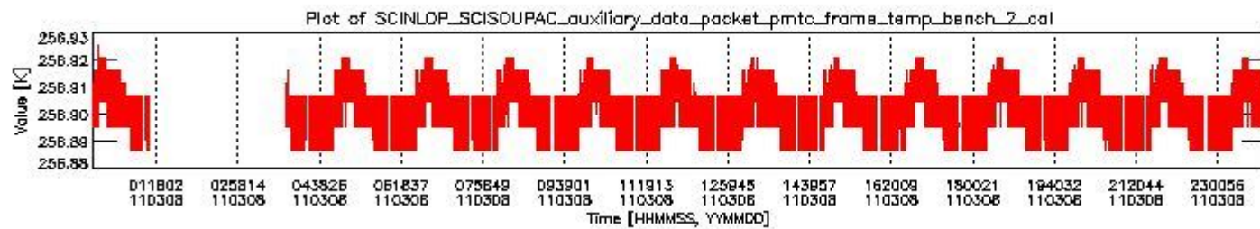
sciamachy_daily_report_level0_KSPT_L0_4504_N_20110308_1.PNG
