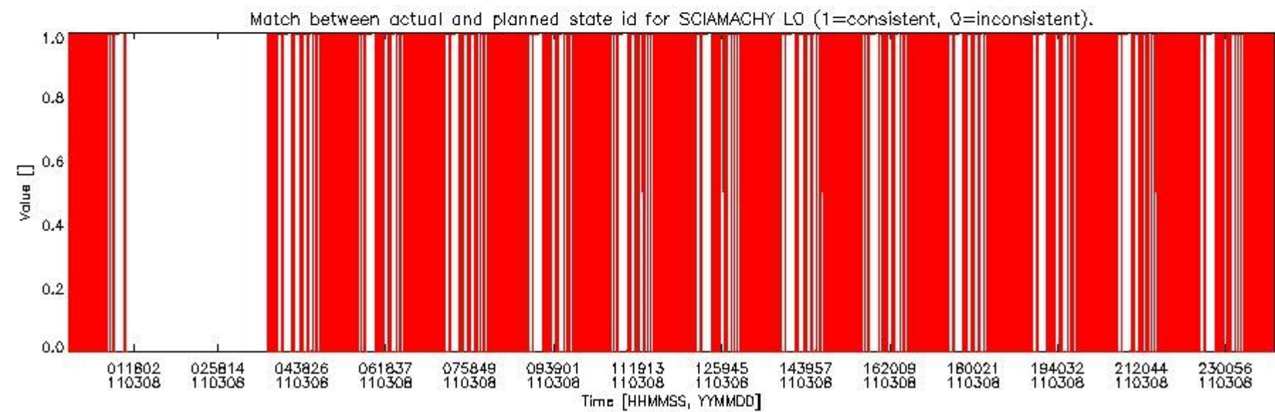
sciamachy_daily_report_level0_KSPT_L0_4504_N_20110308_5.PNG
