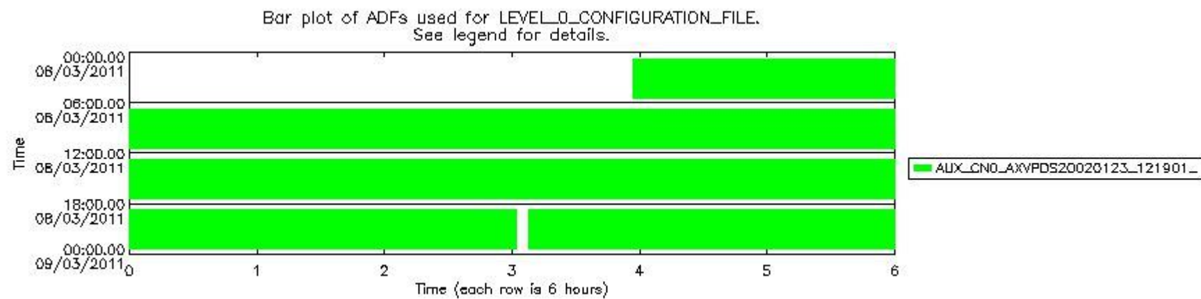
sciamachy_daily_report_level0_KSPT_L0_4504_N_20110308_7.PNG
