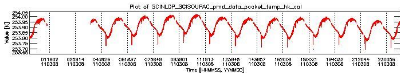
sciamachy_daily_report_level0_KSPT_L0_4504_N_20110308_3.PNG
