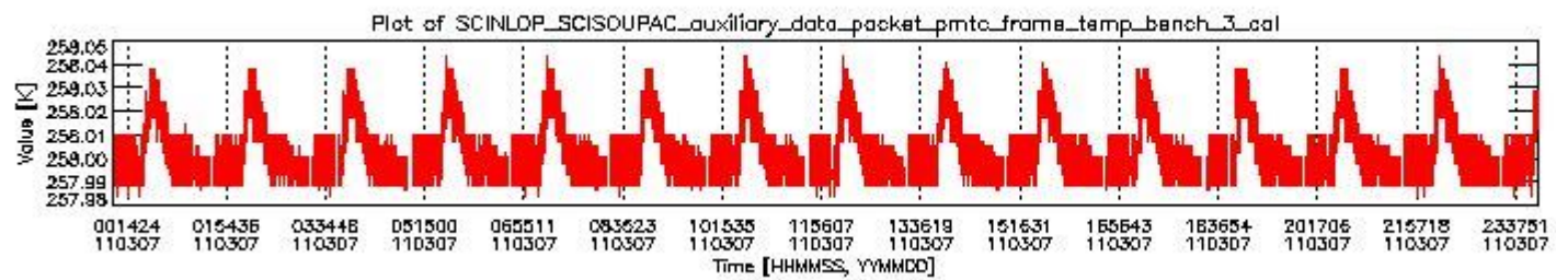
sciamachy_daily_report_level0_KSPT_L0_4504_N_20110307_2.PNG
