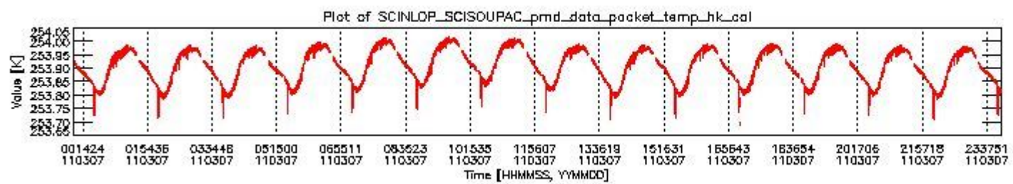
sciamachy_daily_report_level0_KSPT_L0_4504_N_20110307_3.PNG
