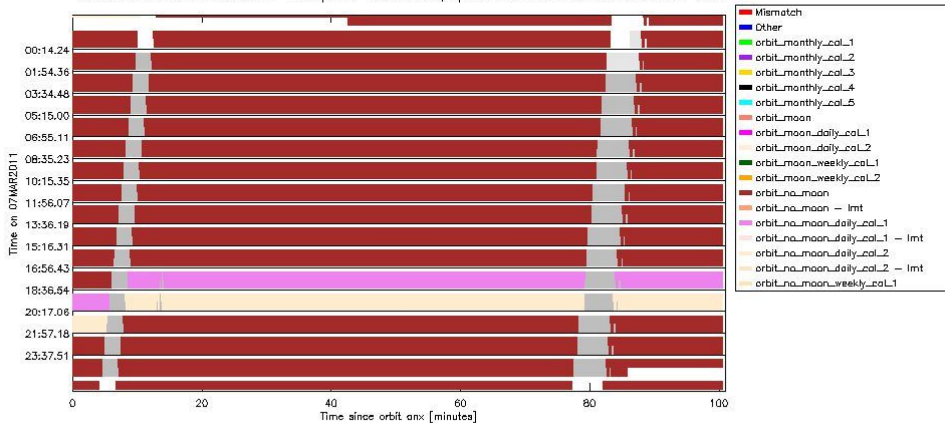
sciamachy_daily_report_level0_KSPT_L0_4504_N_20110307_6.PNG
