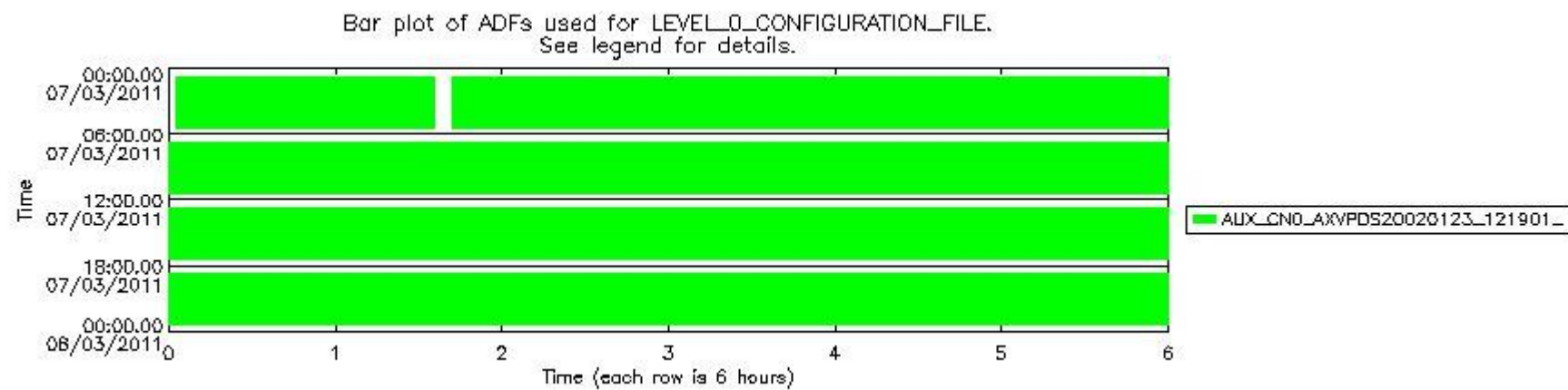
sciamachy_daily_report_level0_KSPT_L0_4504_N_20110307_7.PNG
