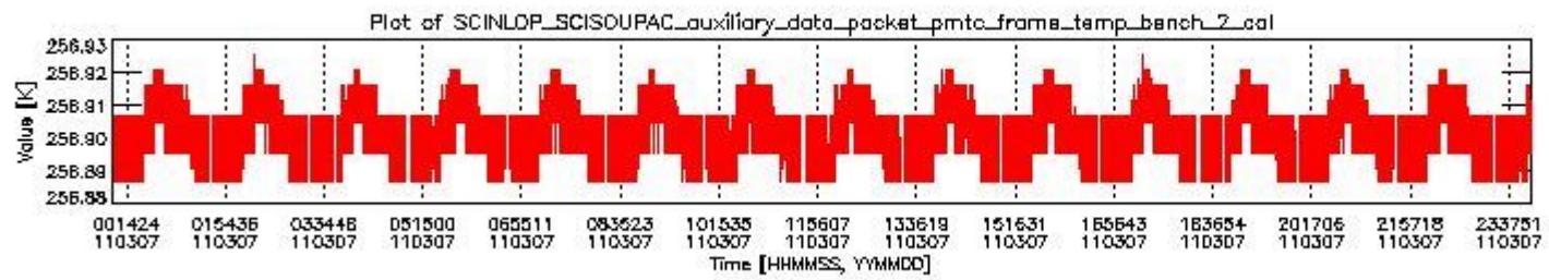
sciamachy_daily_report_level0_KSPT_L0_4504_N_20110307_1.PNG
