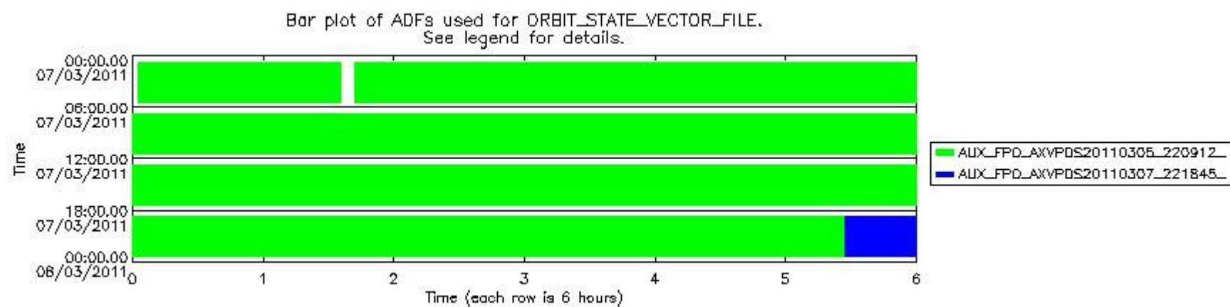
sciamachy_daily_report_level0_KSPT_L0_4504_N_20110307_8.PNG
