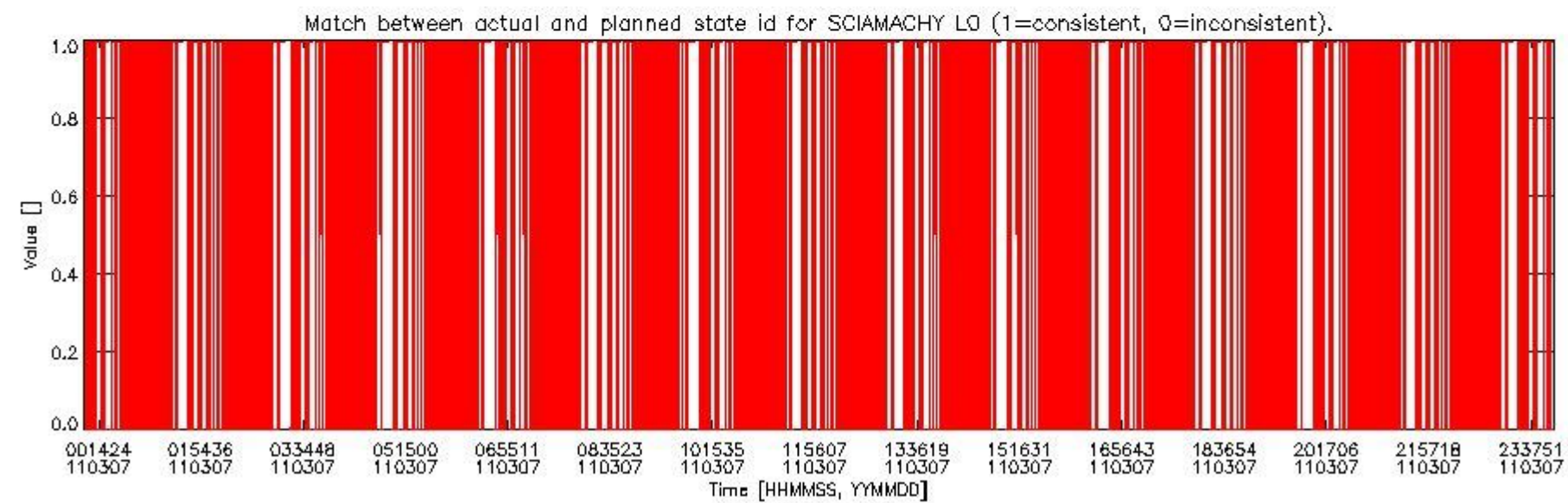
sciamachy_daily_report_level0_KSPT_L0_4504_N_20110307_5.PNG
