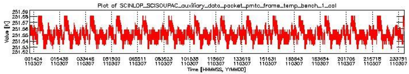
sciamachy_daily_report_level0_KSPT_L0_4504_N_20110307_0.PNG
