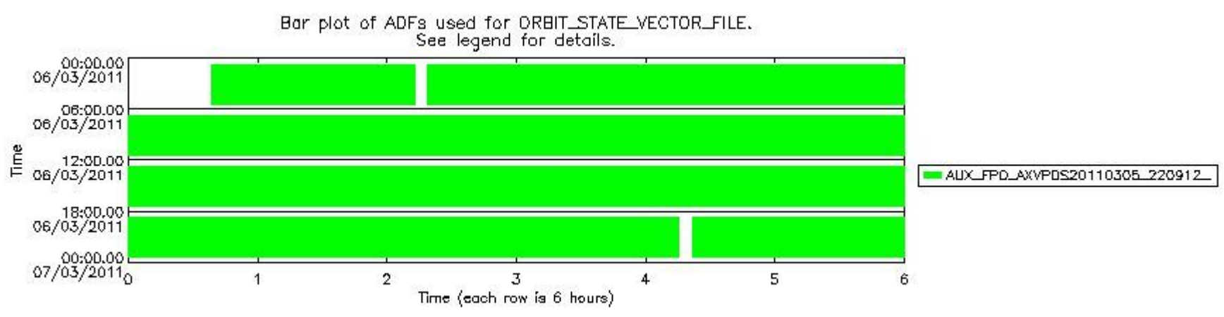
sciamachy_daily_report_level0_KSPT_L0_4504_N_20110306_8.PNG
