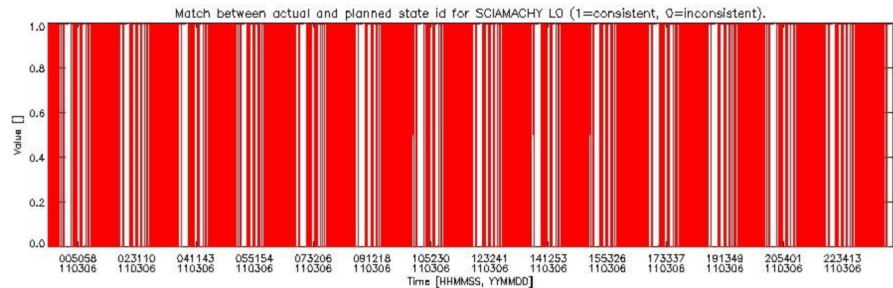
sciamachy_daily_report_level0_KSPT_L0_4504_N_20110306_5.PNG
