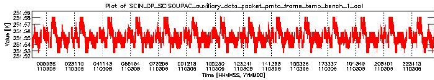
sciamachy_daily_report_level0_KSPT_L0_4504_N_20110306_0.PNG
