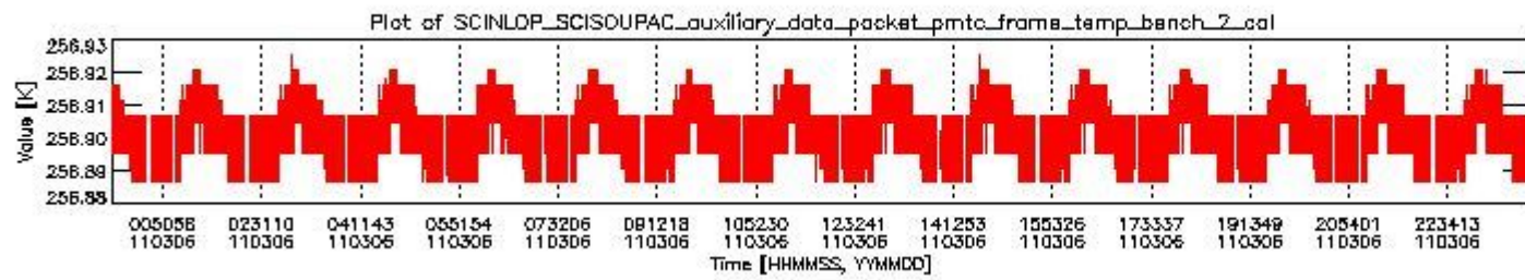
sciamachy_daily_report_level0_KSPT_L0_4504_N_20110306_1.PNG
