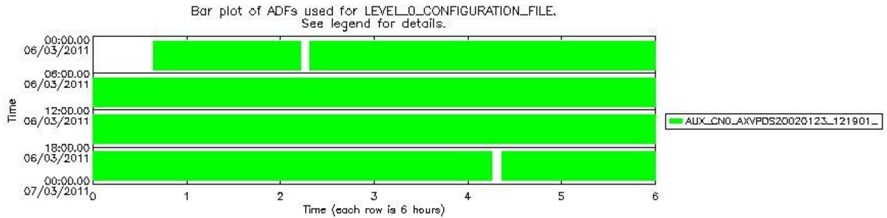
sciamachy_daily_report_level0_KSPT_L0_4504_N_20110306_7.PNG
