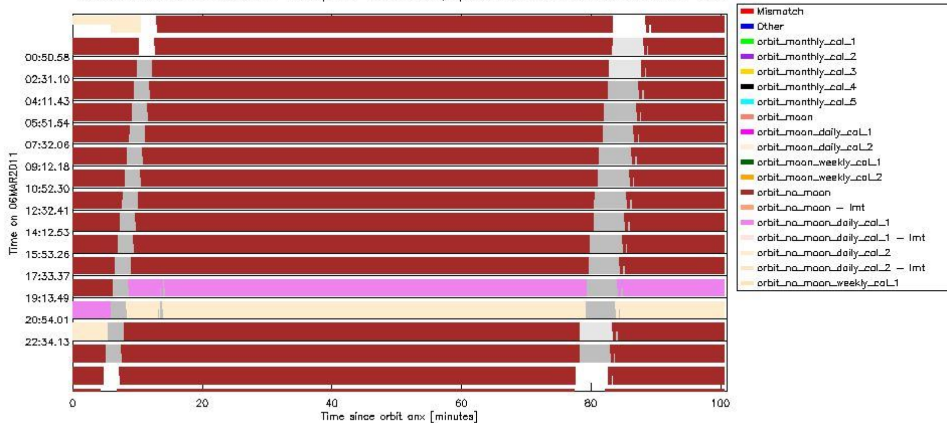
sciamachy_daily_report_level0_KSPT_L0_4504_N_20110306_6.PNG
