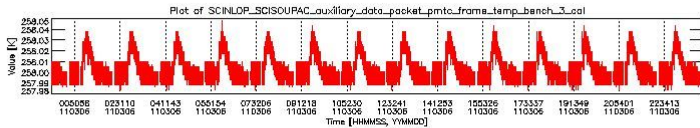
sciamachy_daily_report_level0_KSPT_L0_4504_N_20110306_2.PNG
