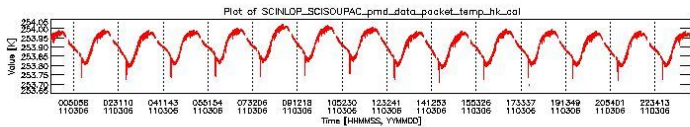
sciamachy_daily_report_level0_KSPT_L0_4504_N_20110306_3.PNG
