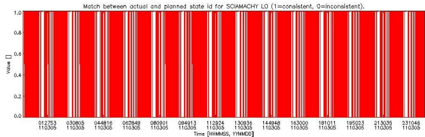
sciamachy_daily_report_level0_KSPT_L0_4504_N_20110305_5.PNG
