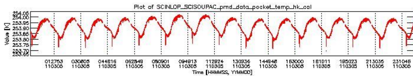
sciamachy_daily_report_level0_KSPT_L0_4504_N_20110305_3.PNG
