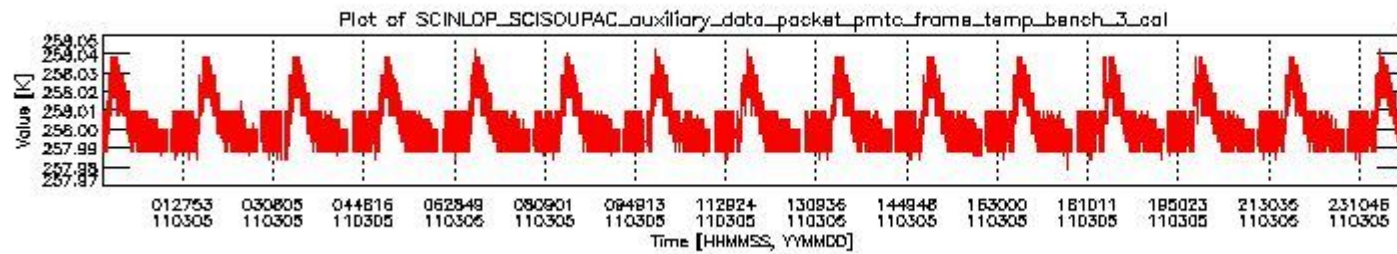
sciamachy_daily_report_level0_KSPT_L0_4504_N_20110305_2.PNG
