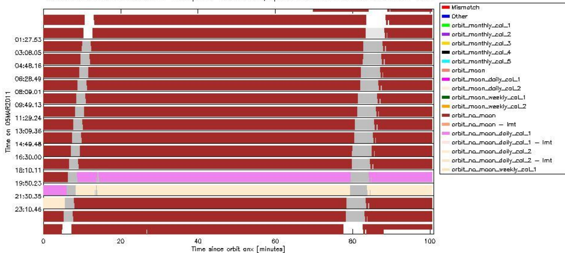
sciamachy_daily_report_level0_KSPT_L0_4504_N_20110305_6.PNG
