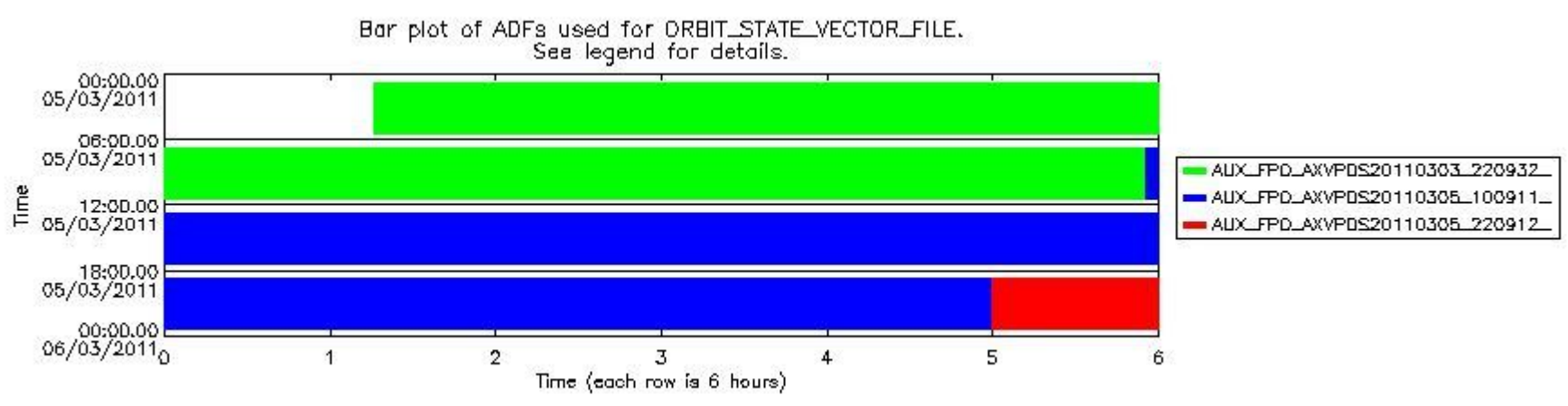
sciamachy_daily_report_level0_KSPT_L0_4504_N_20110305_8.PNG
