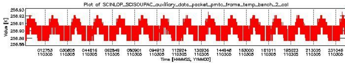
sciamachy_daily_report_level0_KSPT_L0_4504_N_20110305_1.PNG
