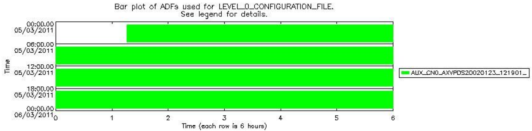
sciamachy_daily_report_level0_KSPT_L0_4504_N_20110305_7.PNG
