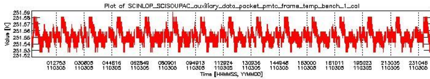
sciamachy_daily_report_level0_KSPT_L0_4504_N_20110305_0.PNG
