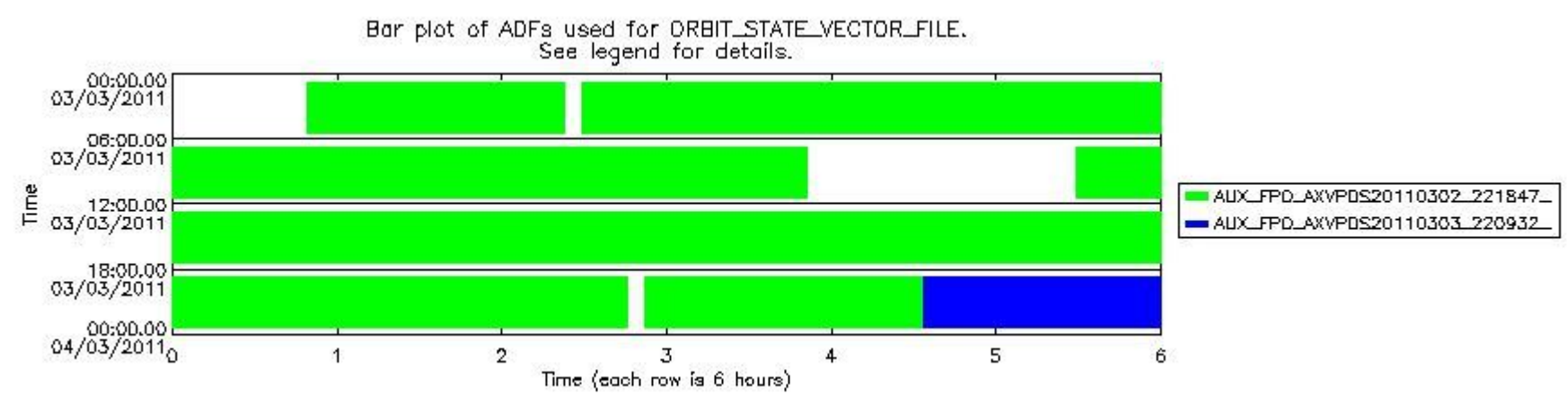
sciamachy_daily_report_level0_KSPT_L0_4504_N_20110303_8.PNG
