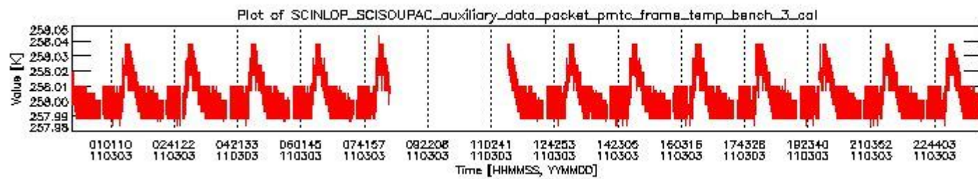
sciamachy_daily_report_level0_KSPT_L0_4504_N_20110303_2.PNG
