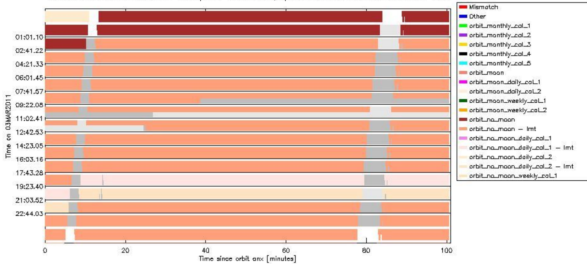
sciamachy_daily_report_level0_KSPT_L0_4504_N_20110303_6.PNG
