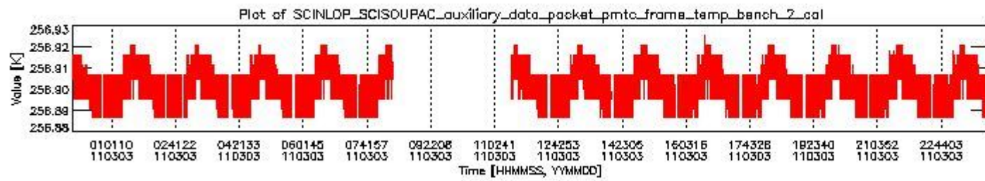
sciamachy_daily_report_level0_KSPT_L0_4504_N_20110303_1.PNG
