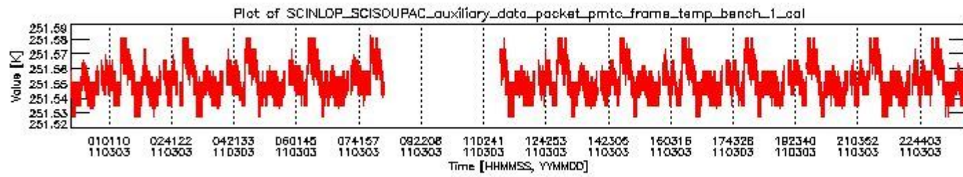
sciamachy_daily_report_level0_KSPT_L0_4504_N_20110303_0.PNG
