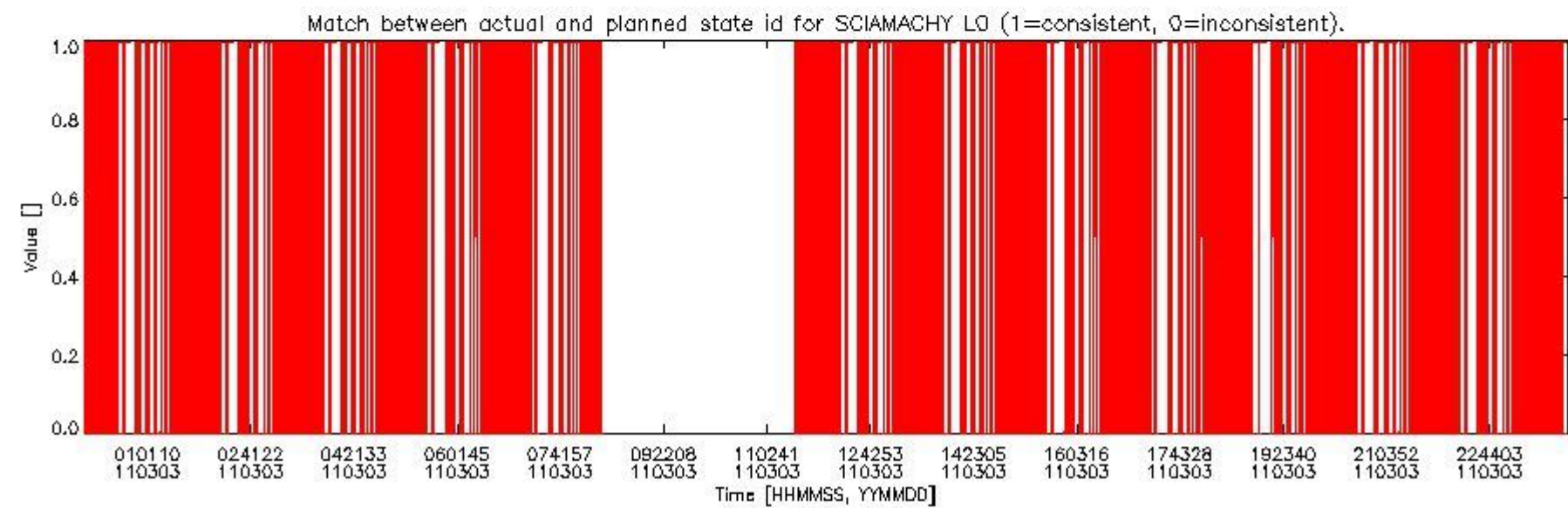
sciamachy_daily_report_level0_KSPT_L0_4504_N_20110303_5.PNG
