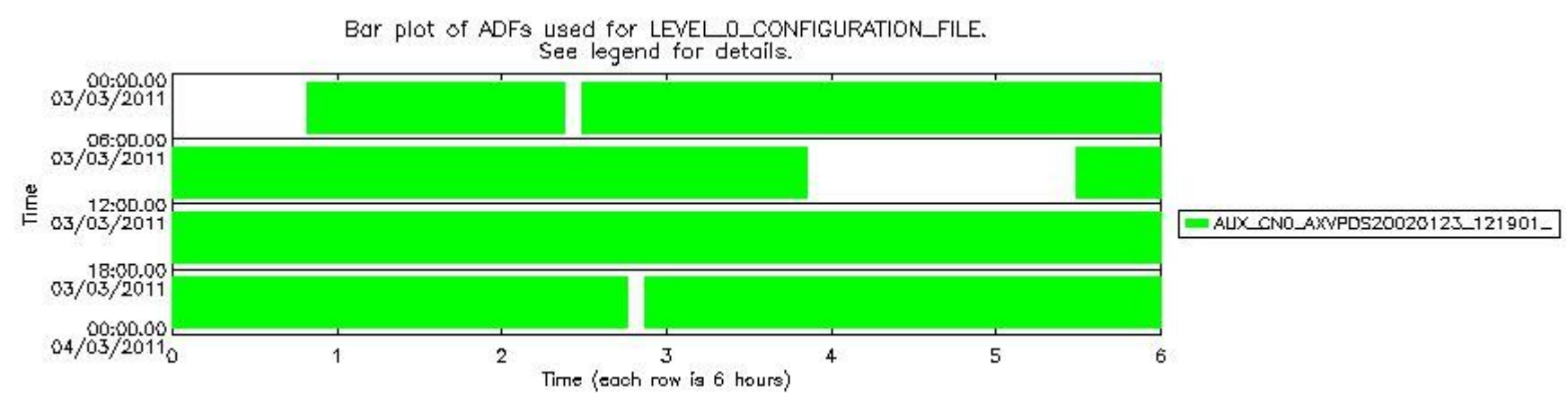
sciamachy_daily_report_level0_KSPT_L0_4504_N_20110303_7.PNG
