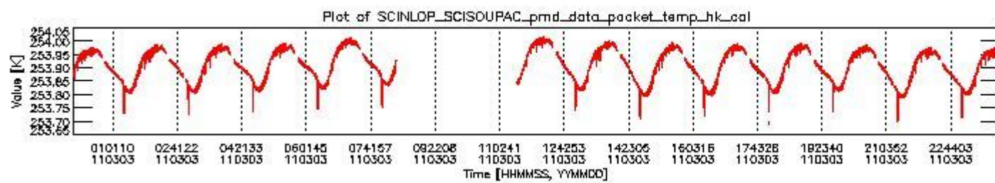
sciamachy_daily_report_level0_KSPT_L0_4504_N_20110303_3.PNG
