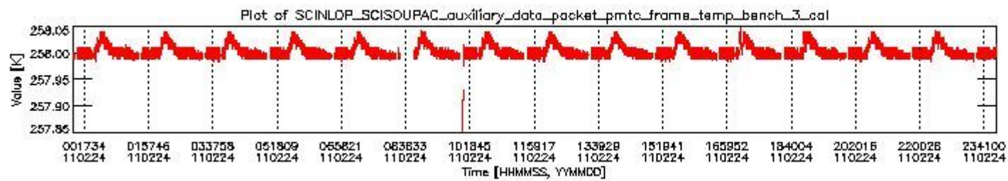
sciamachy_daily_report_level0_KSPT_L0_4504_N_20110224_2.PNG
