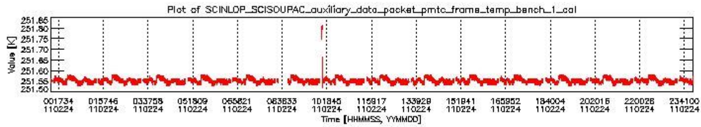
sciamachy_daily_report_level0_KSPT_L0_4504_N_20110224_0.PNG
