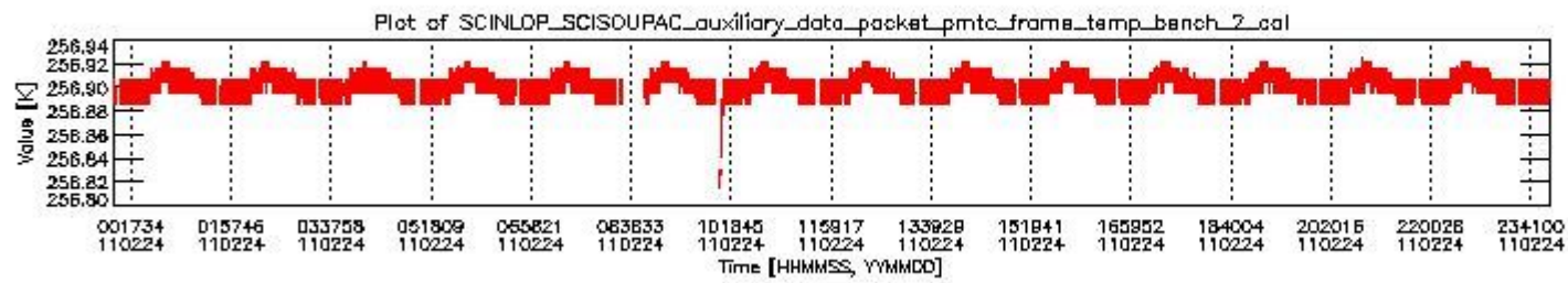
sciamachy_daily_report_level0_KSPT_L0_4504_N_20110224_1.PNG
