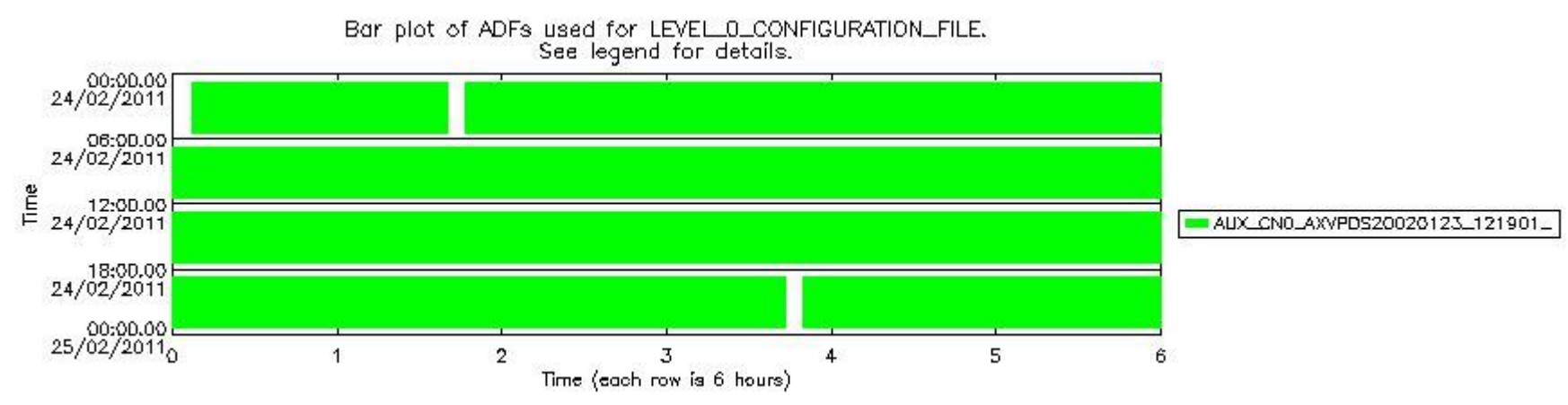
sciamachy_daily_report_level0_KSPT_L0_4504_N_20110224_7.PNG
