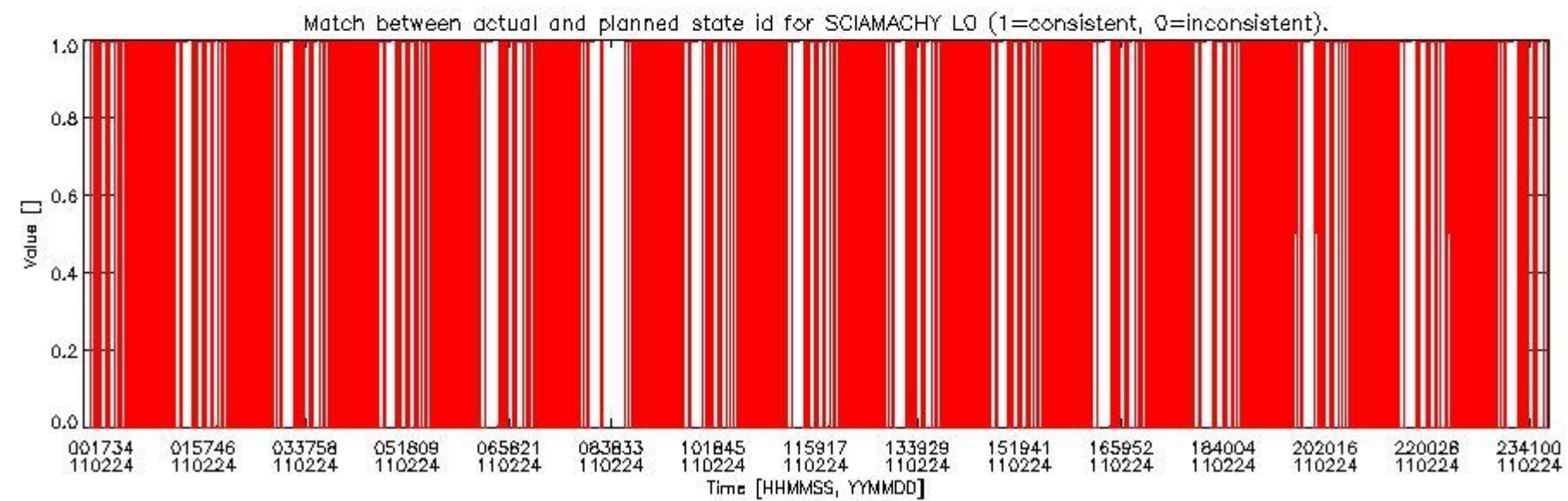
sciamachy_daily_report_level0_KSPT_L0_4504_N_20110224_5.PNG
