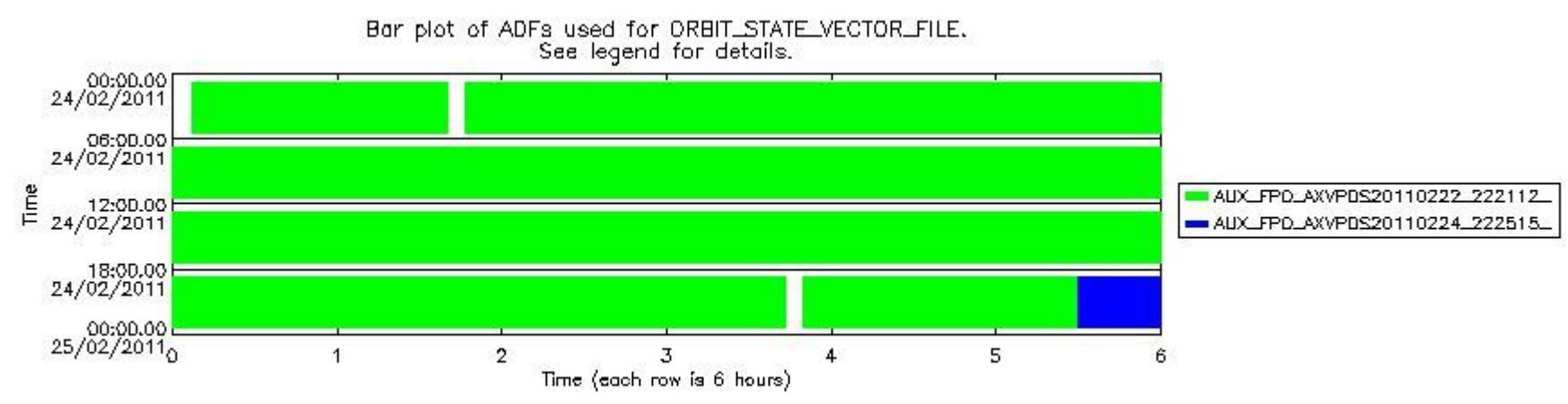
sciamachy_daily_report_level0_KSPT_L0_4504_N_20110224_8.PNG
