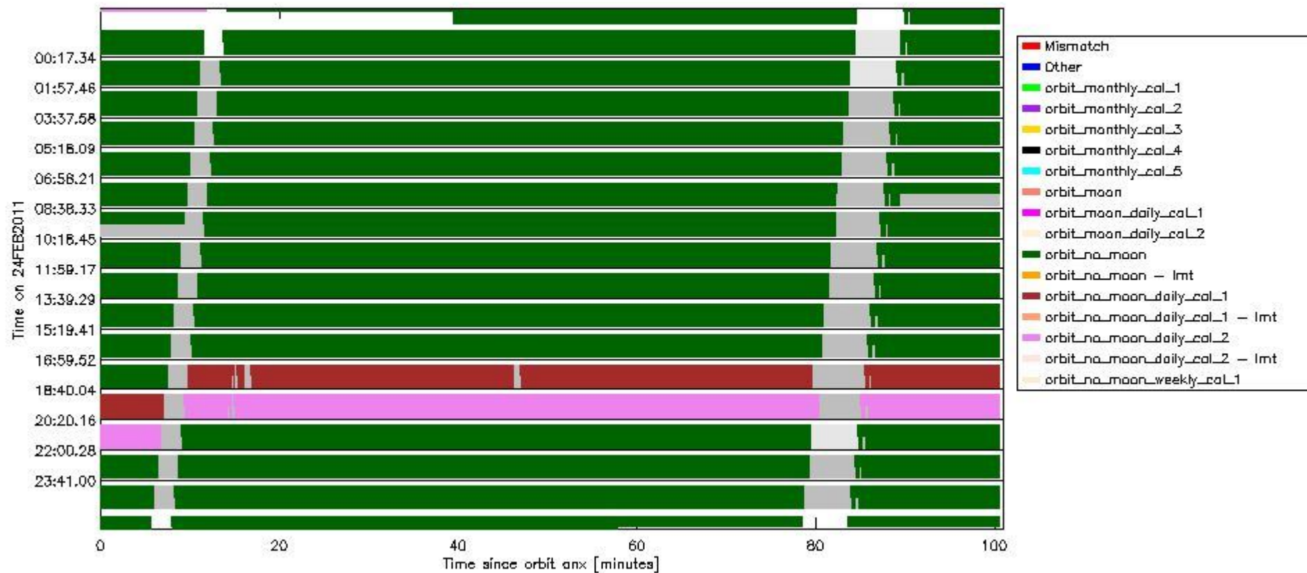
sciamachy_daily_report_level0_KSPT_L0_4504_N_20110224_6.PNG
