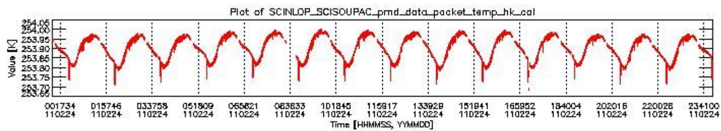
sciamachy_daily_report_level0_KSPT_L0_4504_N_20110224_3.PNG
