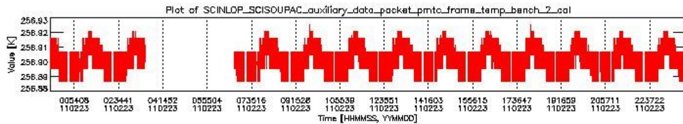
sciamachy_daily_report_level0_KSPT_L0_4504_N_20110223_1.PNG
