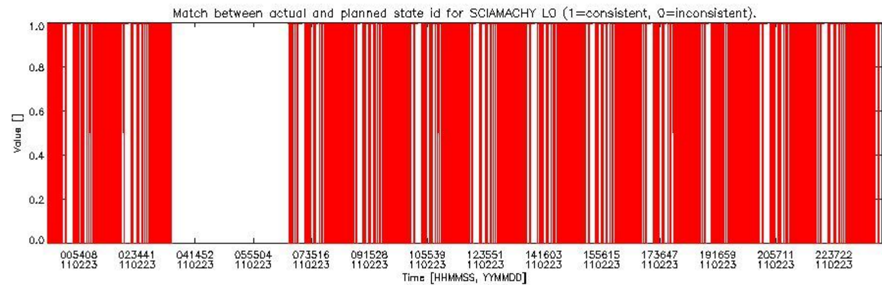
sciamachy_daily_report_level0_KSPT_L0_4504_N_20110223_5.PNG
