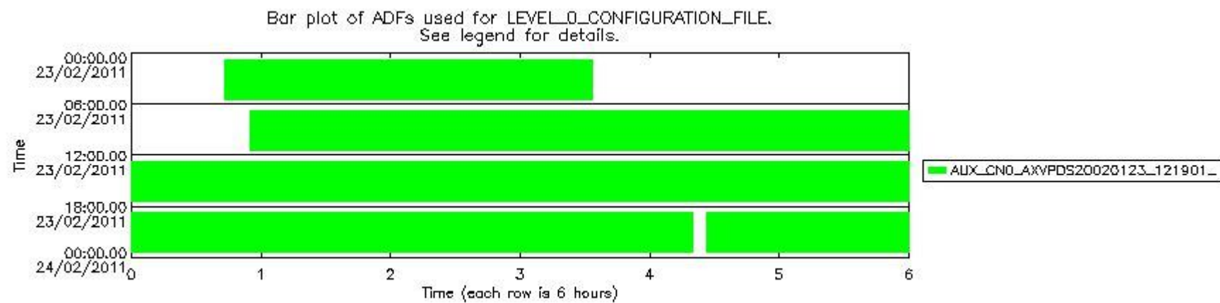
sciamachy_daily_report_level0_KSPT_L0_4504_N_20110223_7.PNG
