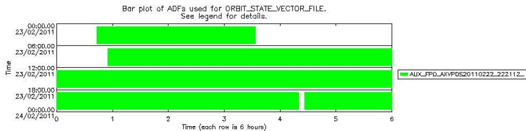
sciamachy_daily_report_level0_KSPT_L0_4504_N_20110223_8.PNG
