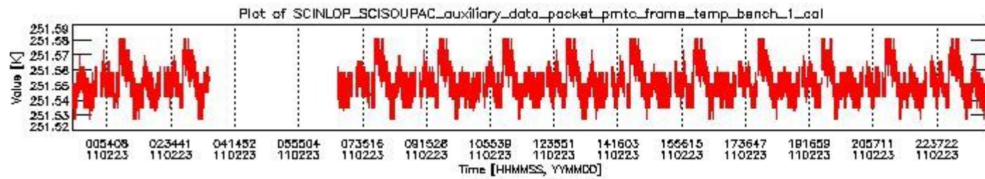
sciamachy_daily_report_level0_KSPT_L0_4504_N_20110223_0.PNG
