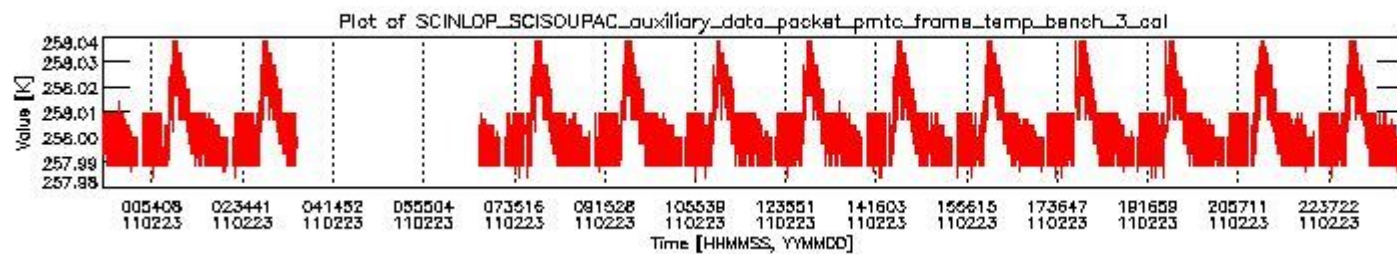
sciamachy_daily_report_level0_KSPT_L0_4504_N_20110223_2.PNG
