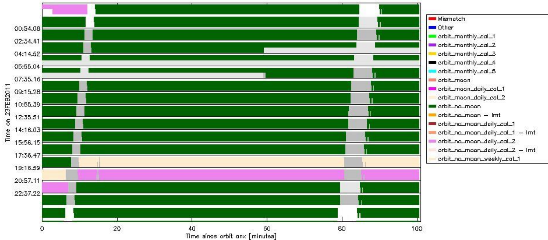
sciamachy_daily_report_level0_KSPT_L0_4504_N_20110223_6.PNG
