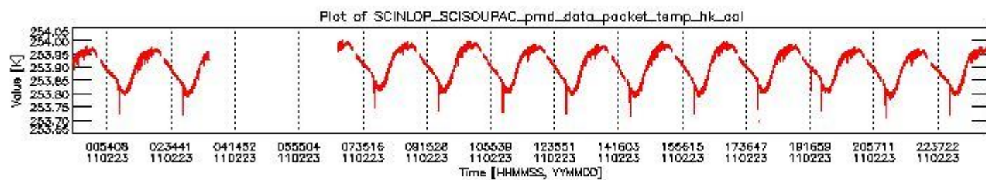
sciamachy_daily_report_level0_KSPT_L0_4504_N_20110223_3.PNG
