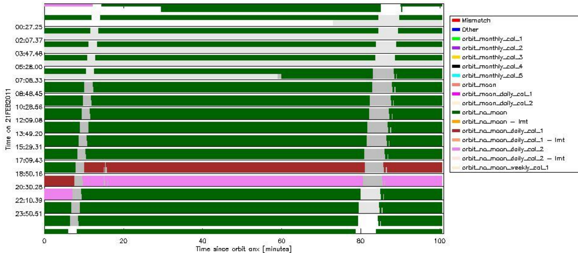
sciamachy_daily_report_level0_KSPT_L0_4504_N_20110221_6.PNG
