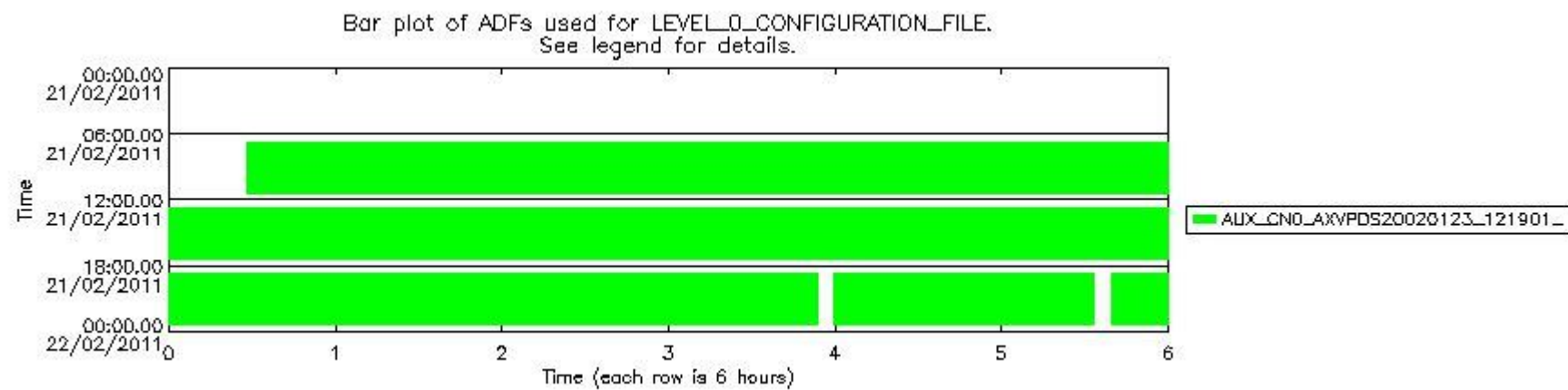
sciamachy_daily_report_level0_KSPT_L0_4504_N_20110221_7.PNG
