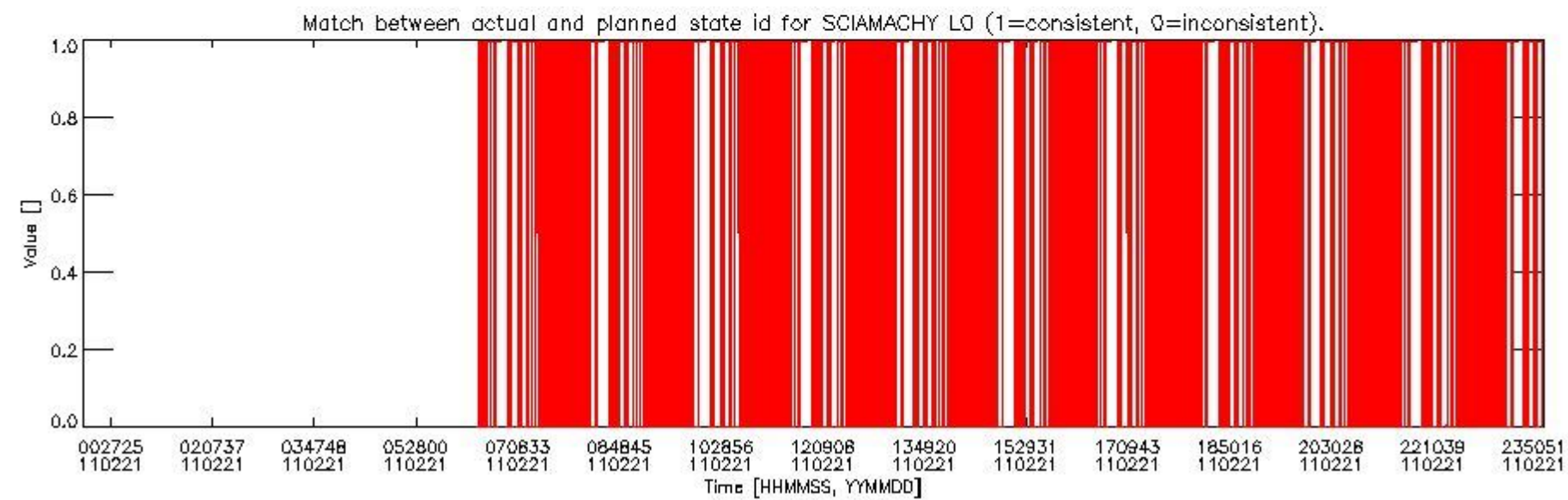
sciamachy_daily_report_level0_KSPT_L0_4504_N_20110221_5.PNG
