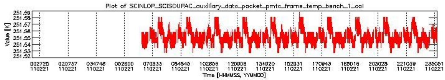
sciamachy_daily_report_level0_KSPT_L0_4504_N_20110221_0.PNG
