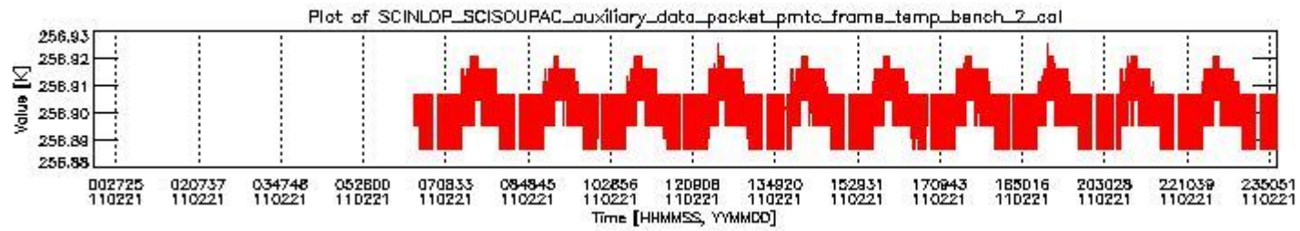
sciamachy_daily_report_level0_KSPT_L0_4504_N_20110221_1.PNG
