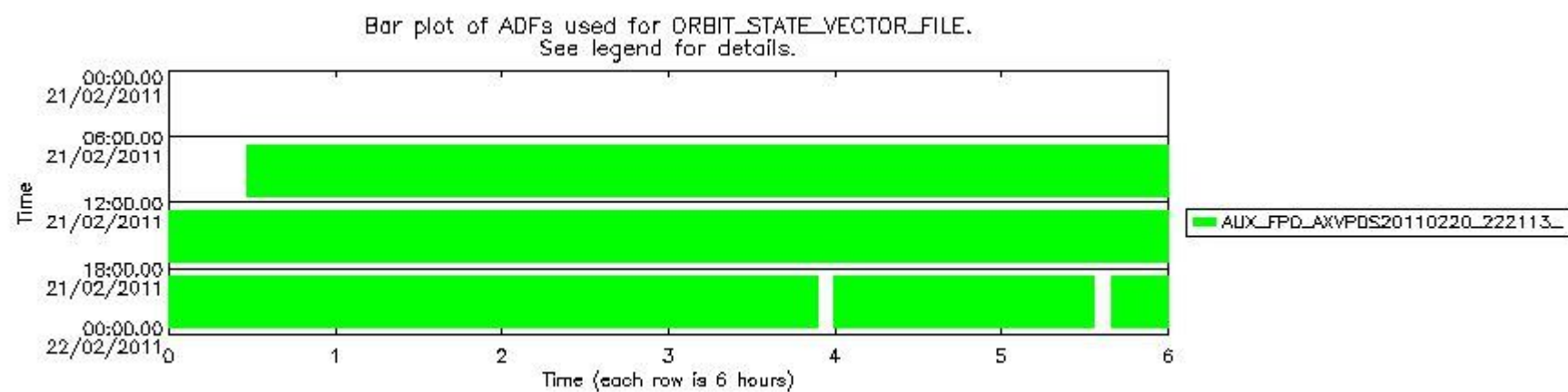
sciamachy_daily_report_level0_KSPT_L0_4504_N_20110221_8.PNG
