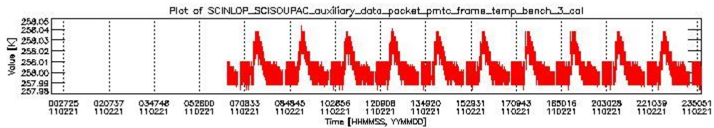
sciamachy_daily_report_level0_KSPT_L0_4504_N_20110221_2.PNG
