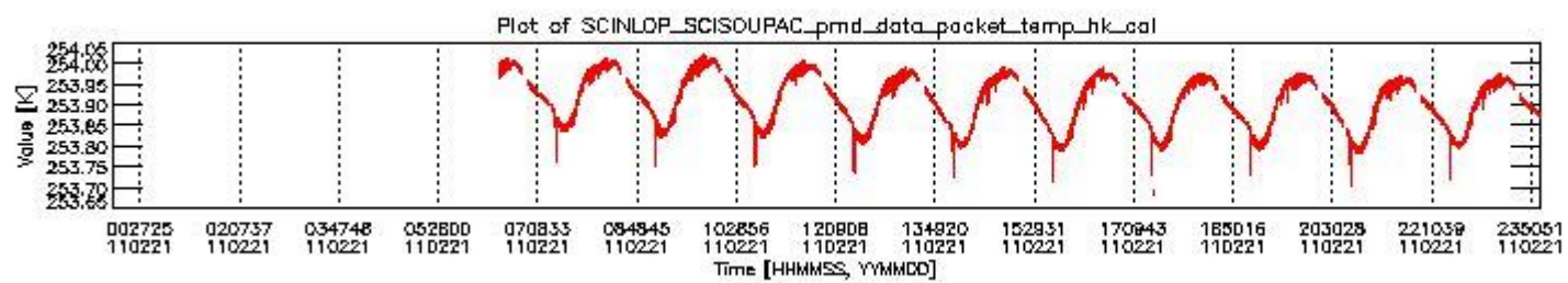
sciamachy_daily_report_level0_KSPT_L0_4504_N_20110221_3.PNG
