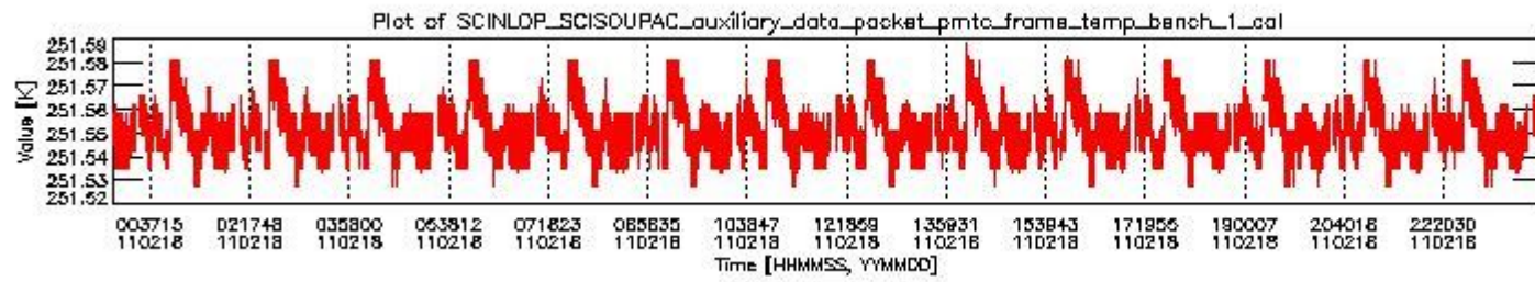
sciamachy_daily_report_level0_KSPT_L0_4504_N_20110218_0.PNG
