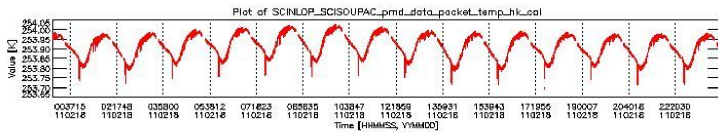
sciamachy_daily_report_level0_KSPT_L0_4504_N_20110218_3.PNG
