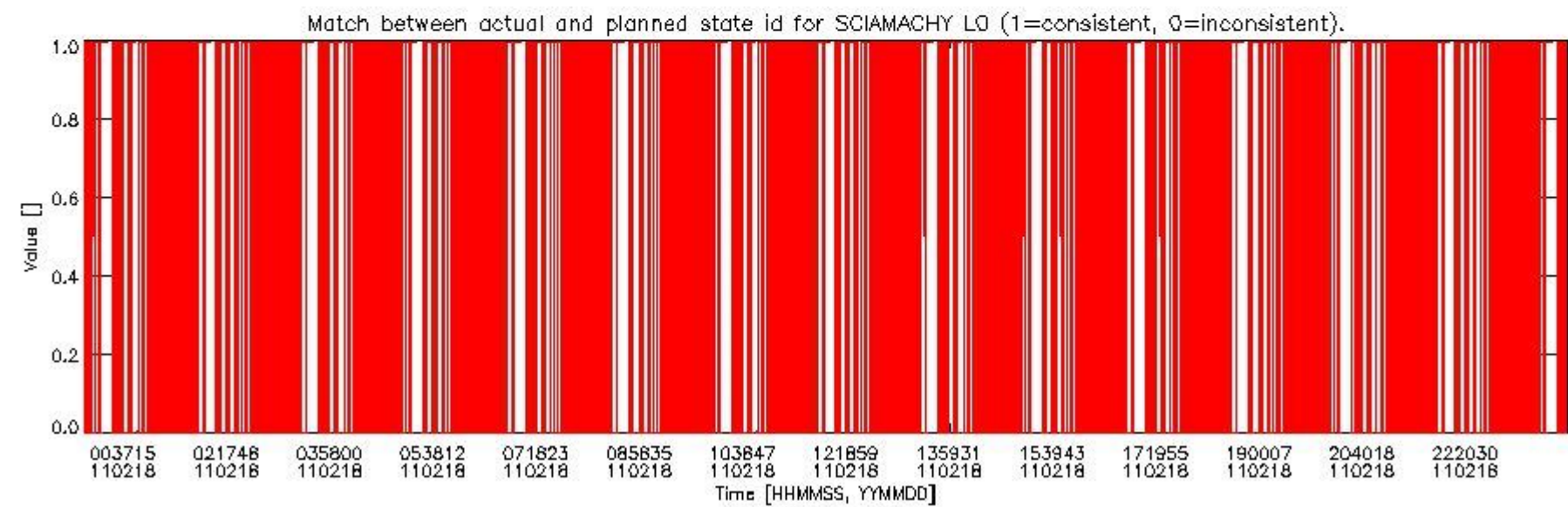
sciamachy_daily_report_level0_KSPT_L0_4504_N_20110218_5.PNG
