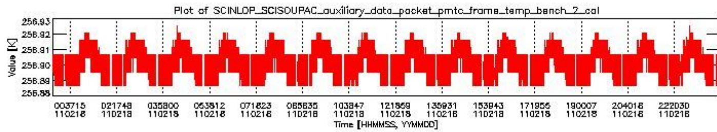
sciamachy_daily_report_level0_KSPT_L0_4504_N_20110218_1.PNG
