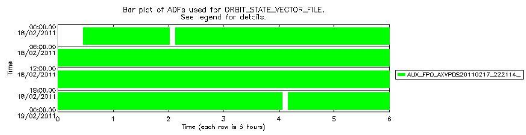
sciamachy_daily_report_level0_KSPT_L0_4504_N_20110218_8.PNG
