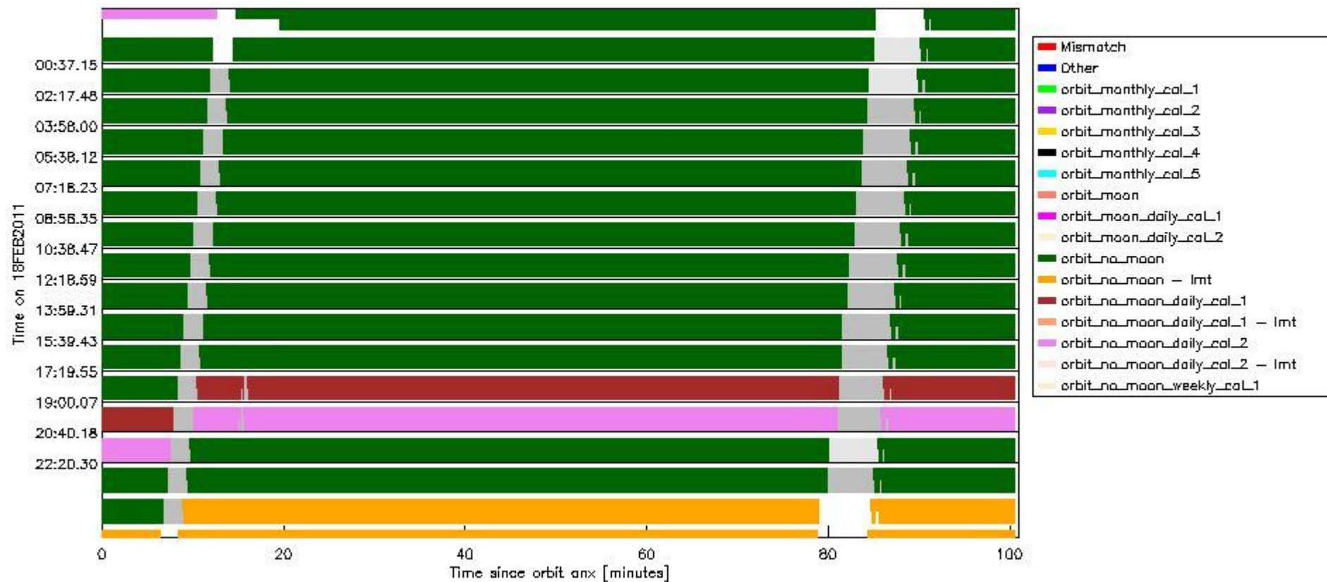
sciamachy_daily_report_level0_KSPT_L0_4504_N_20110218_6.PNG
