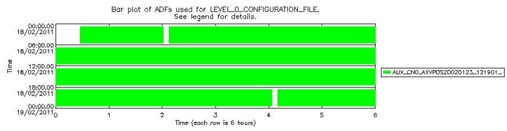
sciamachy_daily_report_level0_KSPT_L0_4504_N_20110218_7.PNG
