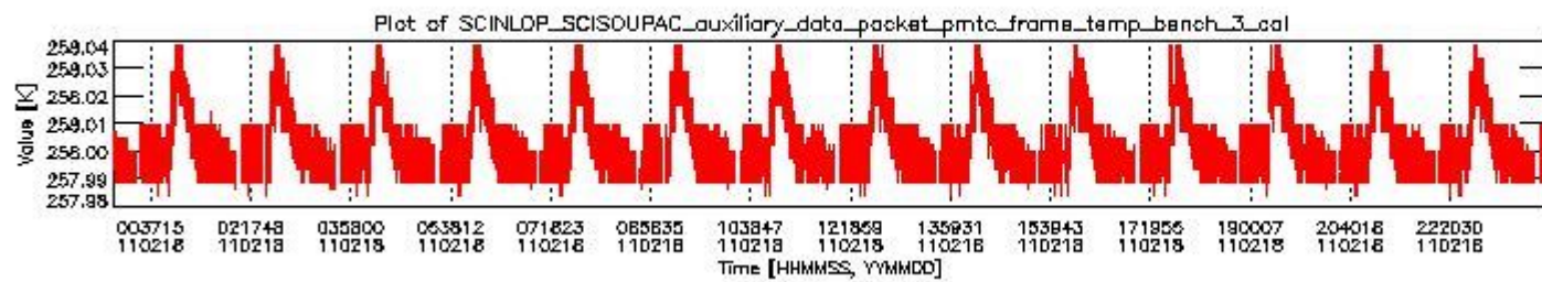
sciamachy_daily_report_level0_KSPT_L0_4504_N_20110218_2.PNG
