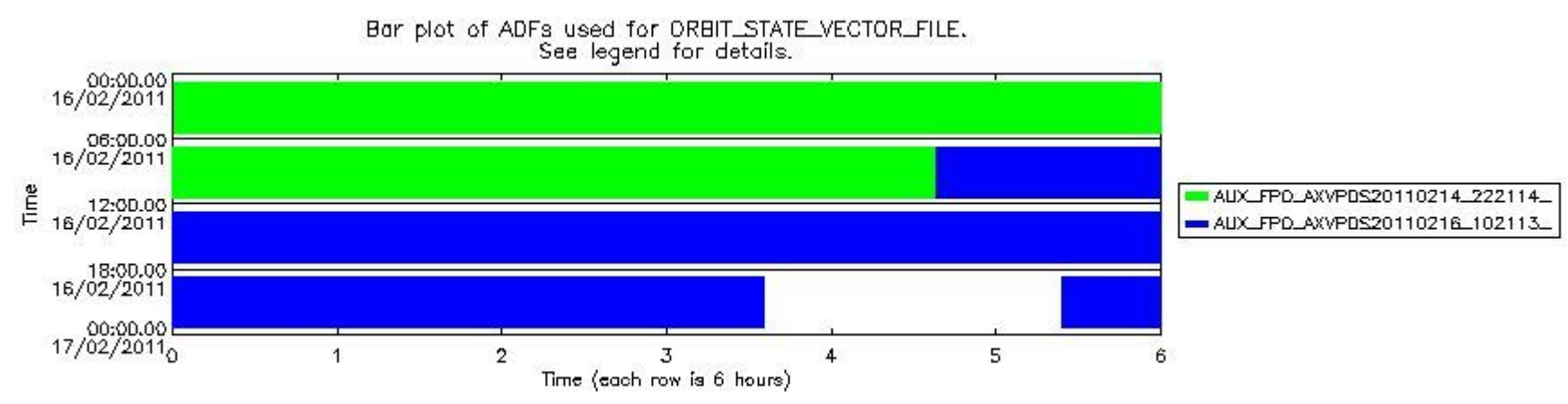
sciamachy_daily_report_level0_KSPT_L0_4504_N_20110216_8.PNG
