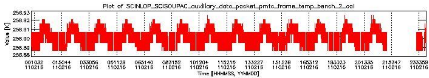
sciamachy_daily_report_level0_KSPT_L0_4504_N_20110216_1.PNG
