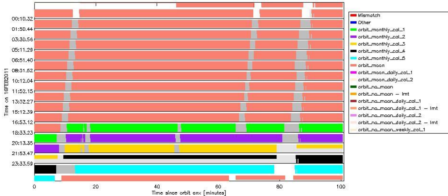
sciamachy_daily_report_level0_KSPT_L0_4504_N_20110216_6.PNG
