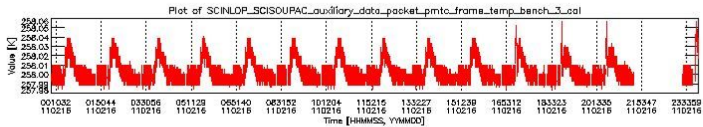
sciamachy_daily_report_level0_KSPT_L0_4504_N_20110216_2.PNG
