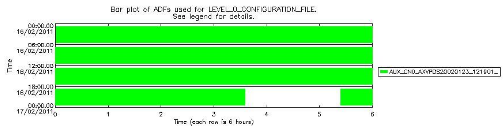
sciamachy_daily_report_level0_KSPT_L0_4504_N_20110216_7.PNG
