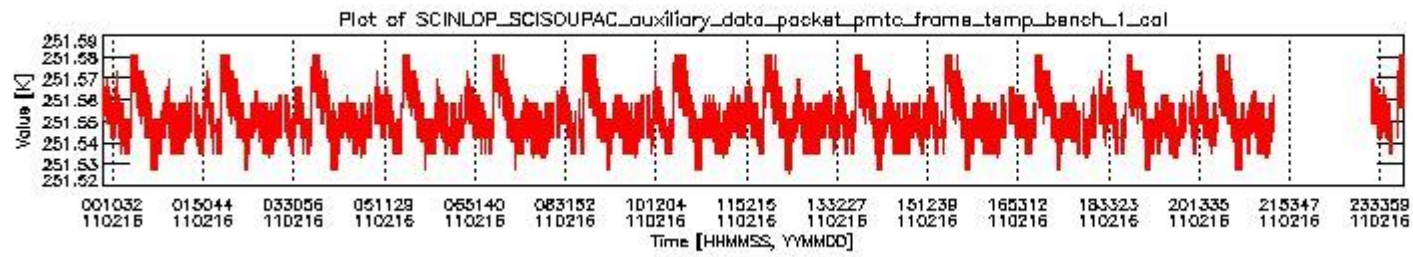
sciamachy_daily_report_level0_KSPT_L0_4504_N_20110216_0.PNG
