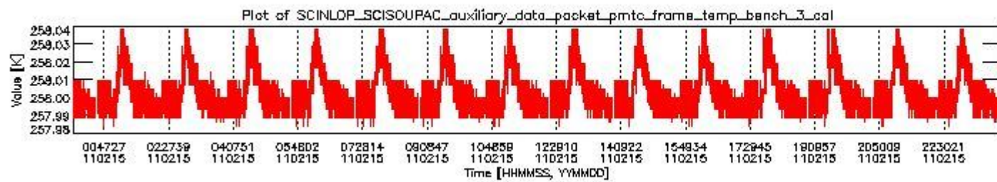
sciamachy_daily_report_level0_KSPT_L0_4504_N_20110215_2.PNG
