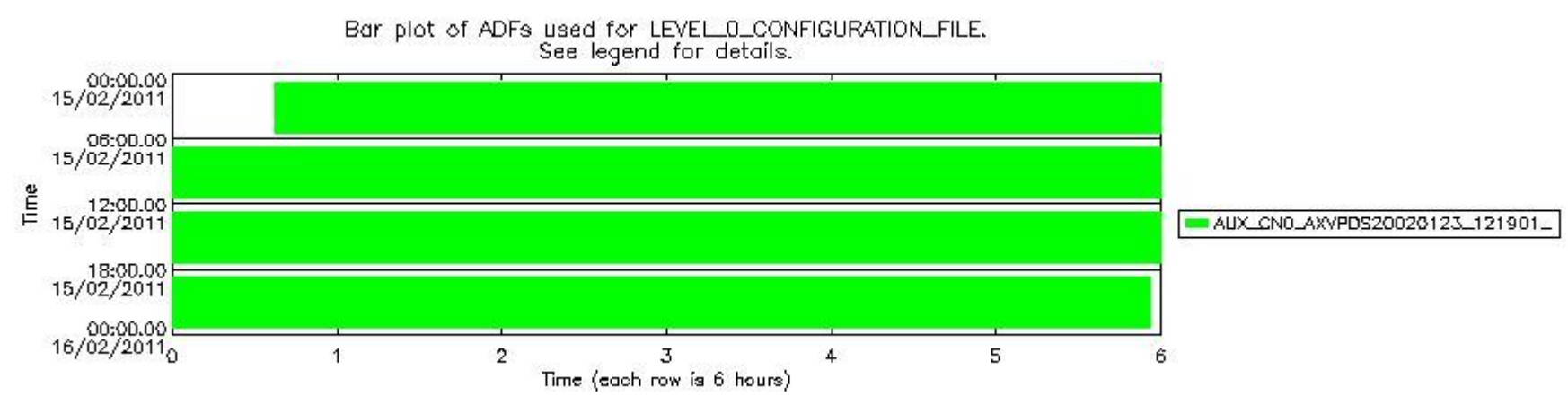
sciamachy_daily_report_level0_KSPT_L0_4504_N_20110215_7.PNG
