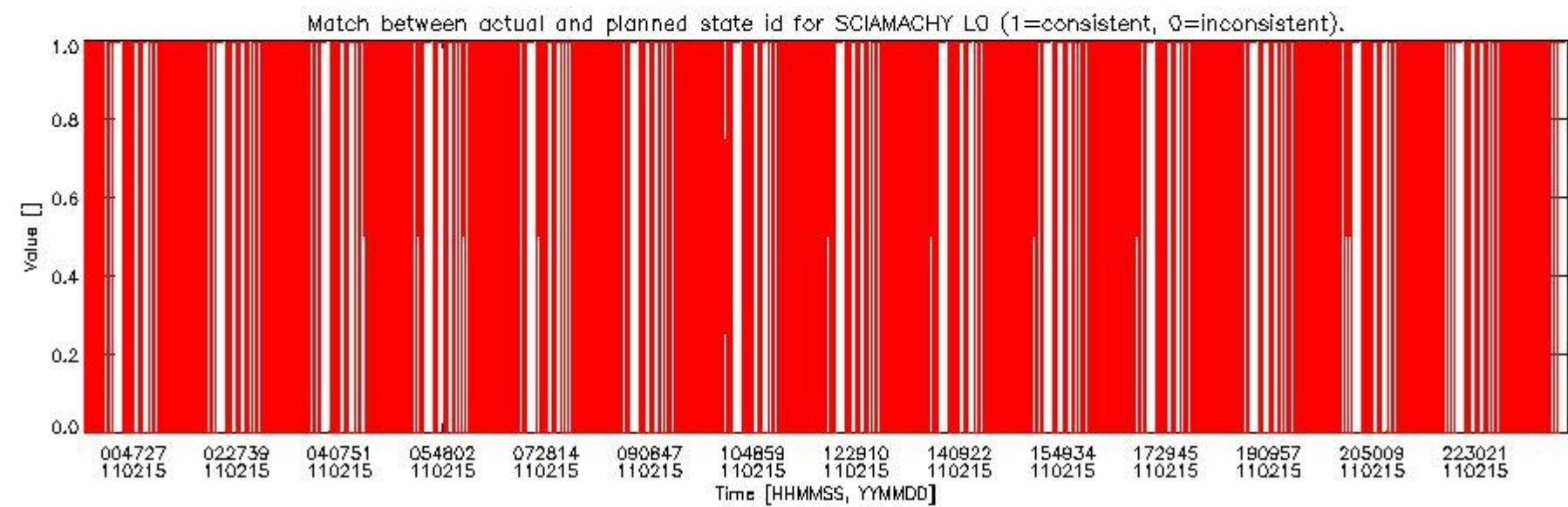
sciamachy_daily_report_level0_KSPT_L0_4504_N_20110215_5.PNG
