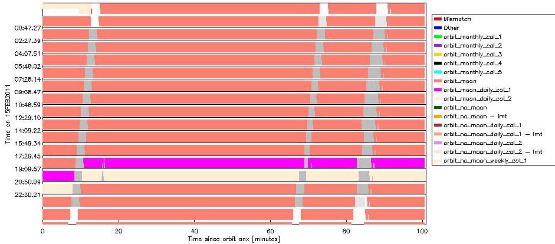
sciamachy_daily_report_level0_KSPT_L0_4504_N_20110215_6.PNG
