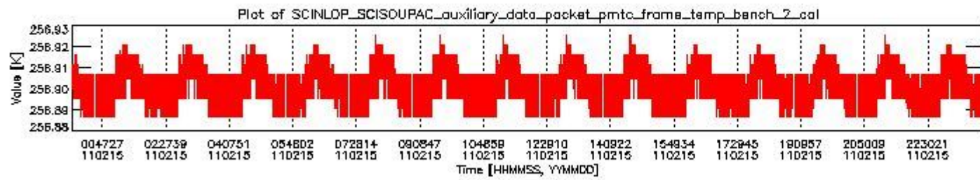
sciamachy_daily_report_level0_KSPT_L0_4504_N_20110215_1.PNG
