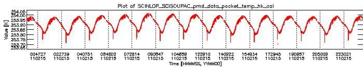
sciamachy_daily_report_level0_KSPT_L0_4504_N_20110215_3.PNG
