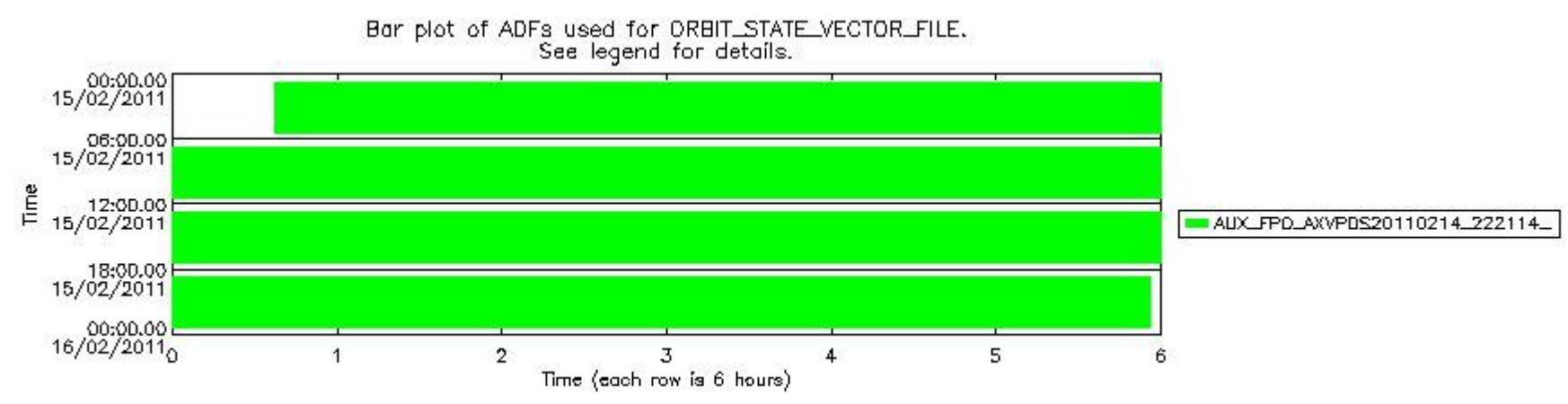
sciamachy_daily_report_level0_KSPT_L0_4504_N_20110215_8.PNG
