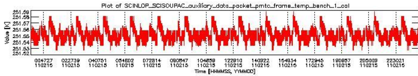
sciamachy_daily_report_level0_KSPT_L0_4504_N_20110215_0.PNG
