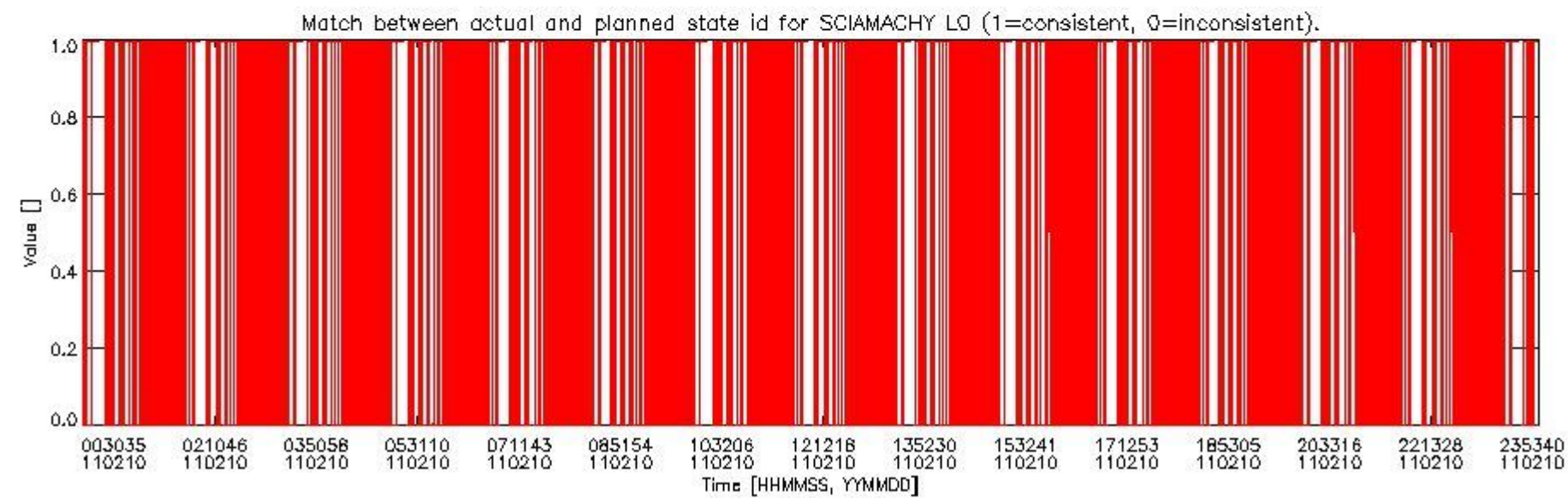
sciamachy_daily_report_level0_KSPT_L0_4504_N_20110210_5.PNG
