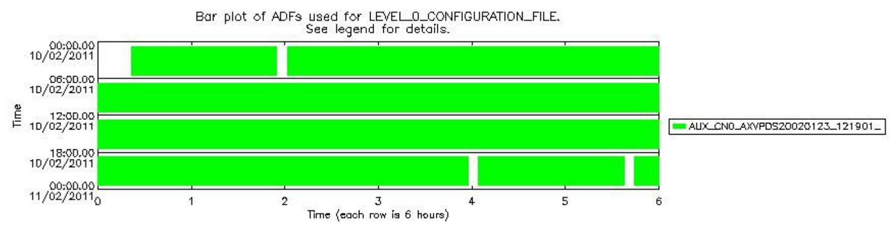
sciamachy_daily_report_level0_KSPT_L0_4504_N_20110210_7.PNG
