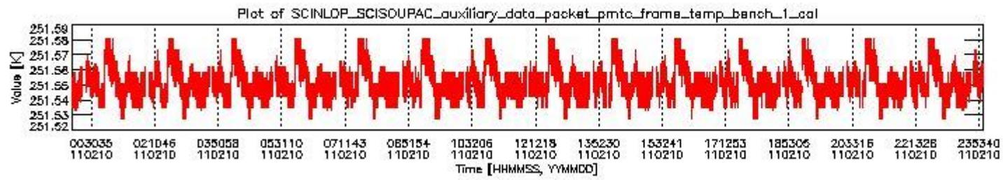
sciamachy_daily_report_level0_KSPT_L0_4504_N_20110210_0.PNG
