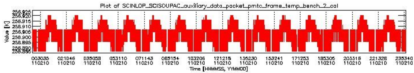
sciamachy_daily_report_level0_KSPT_L0_4504_N_20110210_1.PNG
