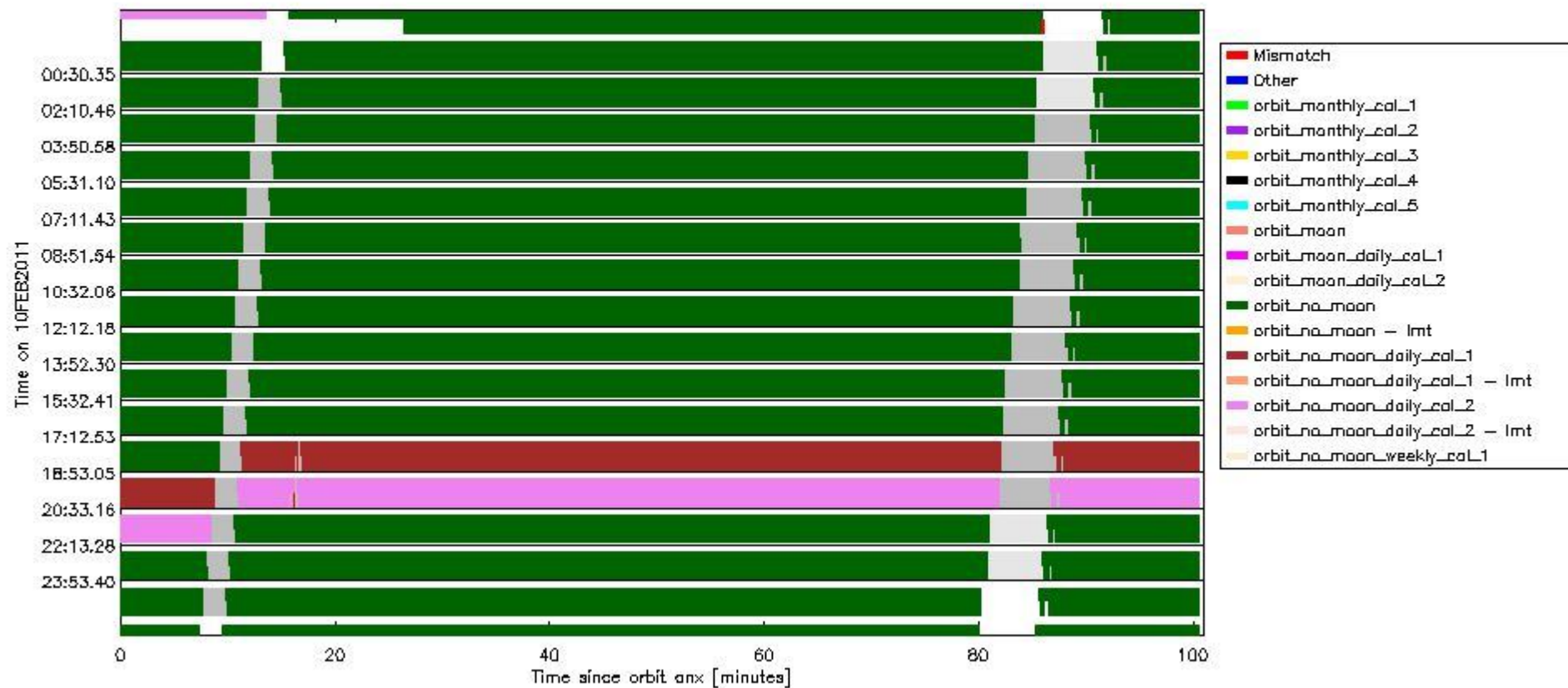
sciamachy_daily_report_level0_KSPT_L0_4504_N_20110210_6.PNG
