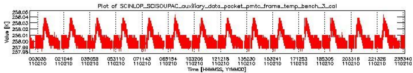
sciamachy_daily_report_level0_KSPT_L0_4504_N_20110210_2.PNG
