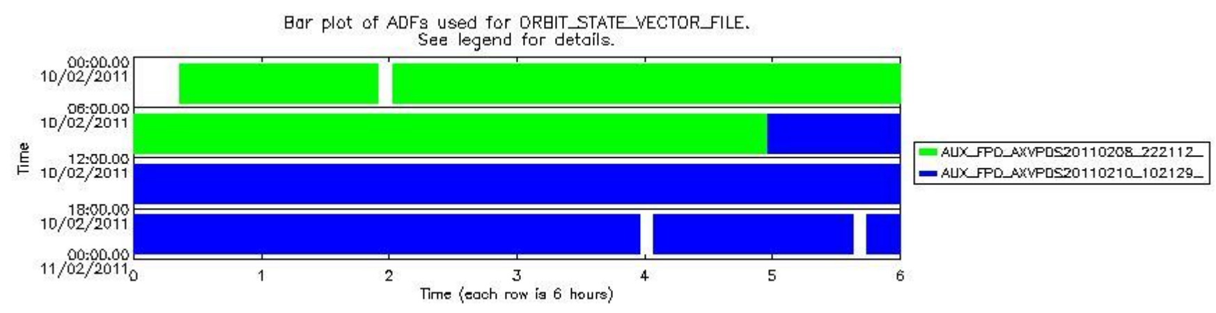
sciamachy_daily_report_level0_KSPT_L0_4504_N_20110210_8.PNG
