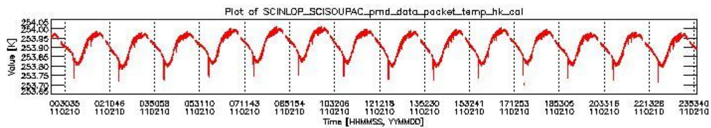
sciamachy_daily_report_level0_KSPT_L0_4504_N_20110210_3.PNG
