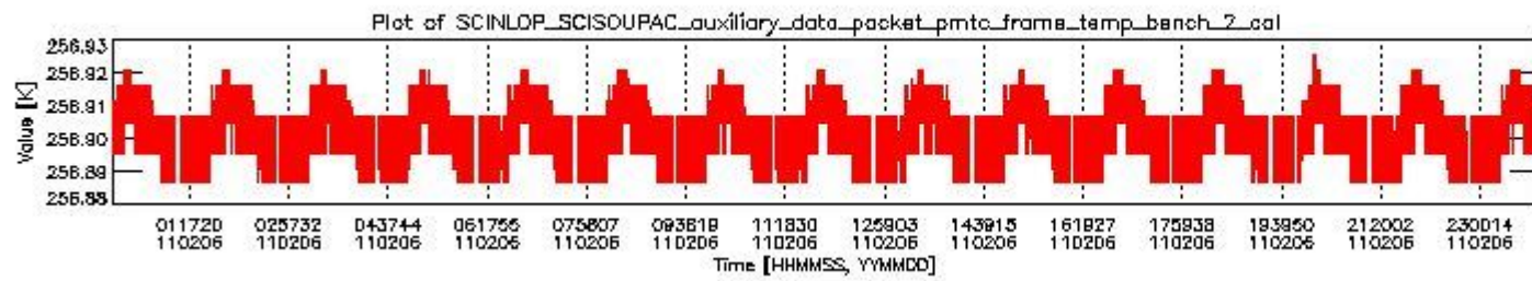
sciamachy_daily_report_level0_KSPT_L0_4504_N_20110206_1.PNG
