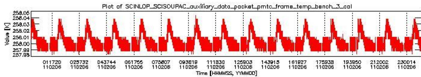
sciamachy_daily_report_level0_KSPT_L0_4504_N_20110206_2.PNG
