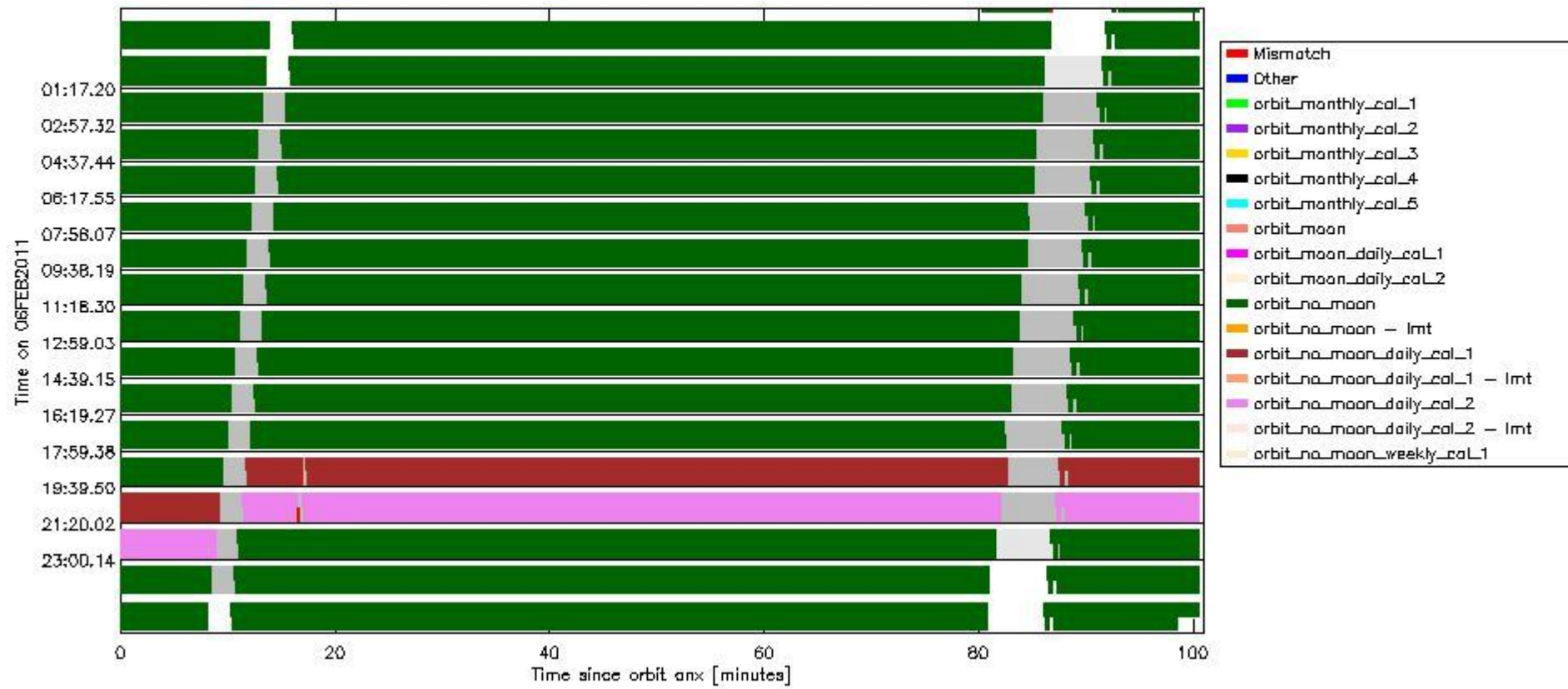
sciamachy_daily_report_level0_KSPT_L0_4504_N_20110206_6.PNG
