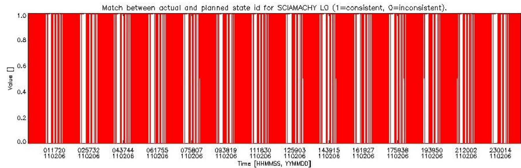
sciamachy_daily_report_level0_KSPT_L0_4504_N_20110206_5.PNG
