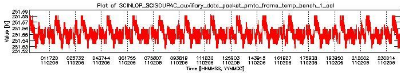
sciamachy_daily_report_level0_KSPT_L0_4504_N_20110206_0.PNG
