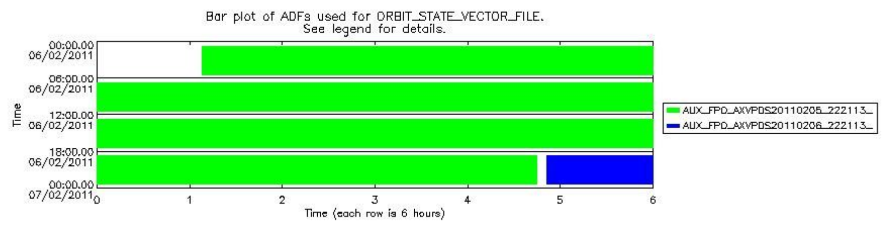
sciamachy_daily_report_level0_KSPT_L0_4504_N_20110206_8.PNG
