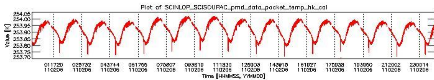
sciamachy_daily_report_level0_KSPT_L0_4504_N_20110206_3.PNG
