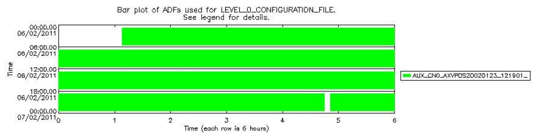
sciamachy_daily_report_level0_KSPT_L0_4504_N_20110206_7.PNG
