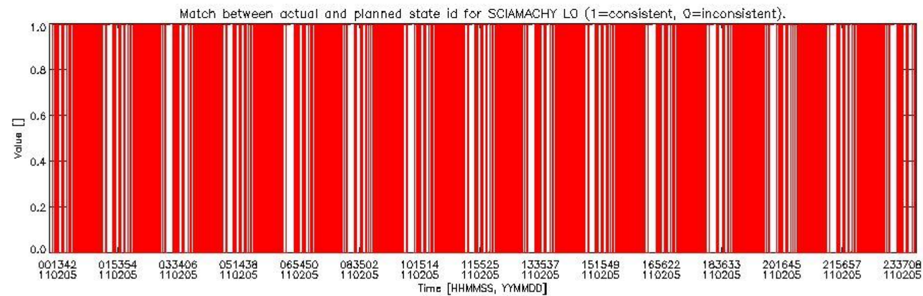
sciamachy_daily_report_level0_KSPT_L0_4504_N_20110205_5.PNG
