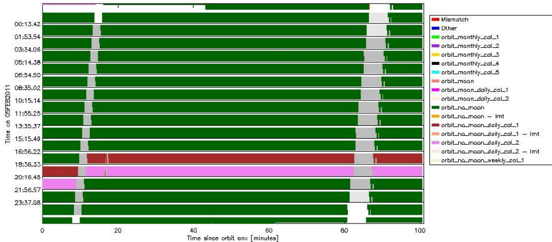
sciamachy_daily_report_level0_KSPT_L0_4504_N_20110205_6.PNG
