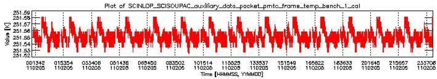
sciamachy_daily_report_level0_KSPT_L0_4504_N_20110205_0.PNG
