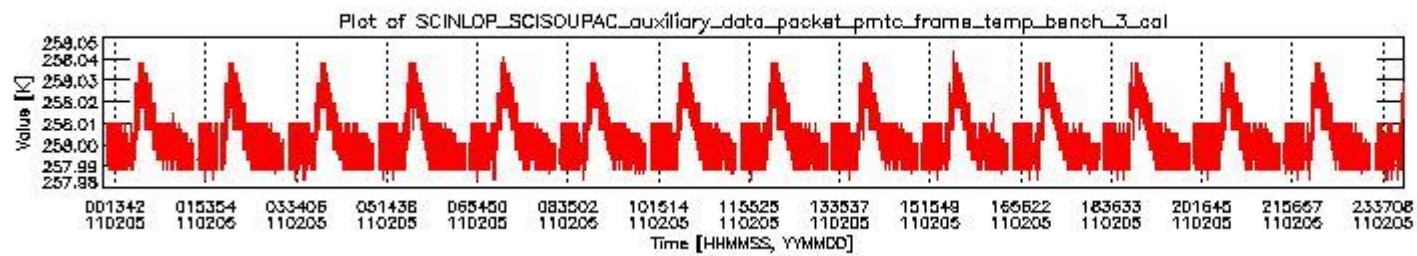
sciamachy_daily_report_level0_KSPT_L0_4504_N_20110205_2.PNG
