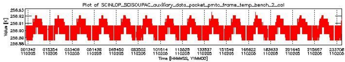
sciamachy_daily_report_level0_KSPT_L0_4504_N_20110205_1.PNG
