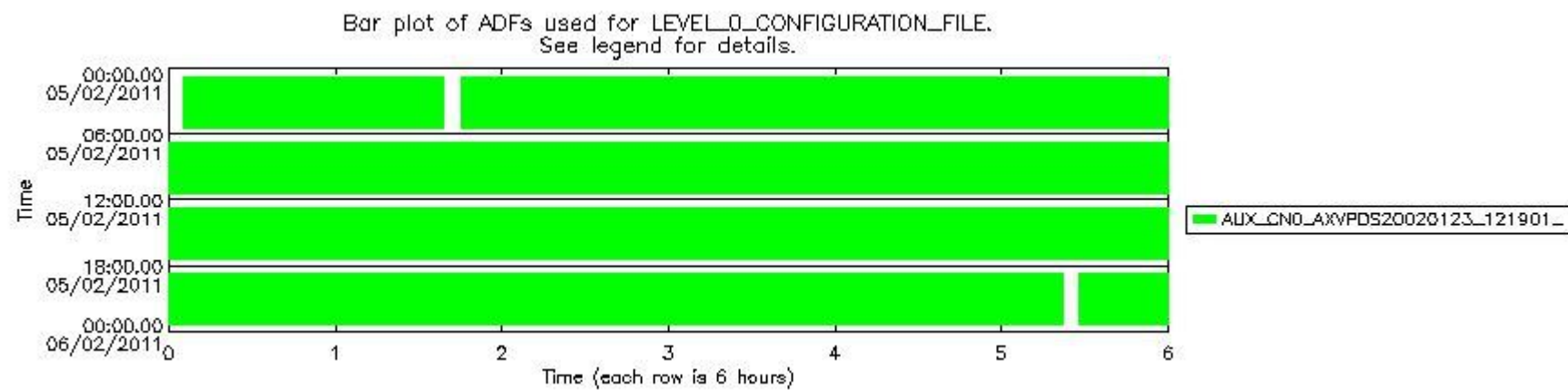
sciamachy_daily_report_level0_KSPT_L0_4504_N_20110205_7.PNG
