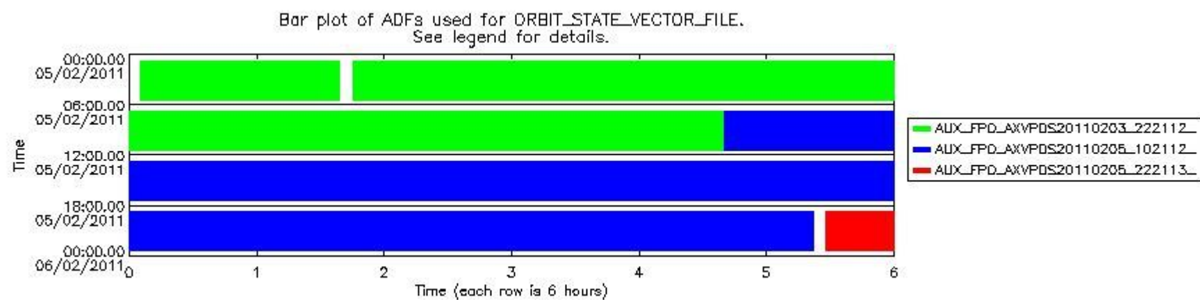
sciamachy_daily_report_level0_KSPT_L0_4504_N_20110205_8.PNG
