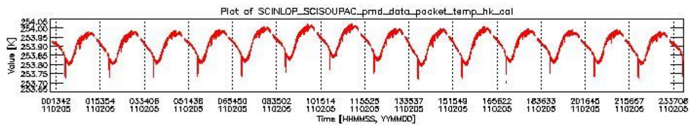
sciamachy_daily_report_level0_KSPT_L0_4504_N_20110205_3.PNG
