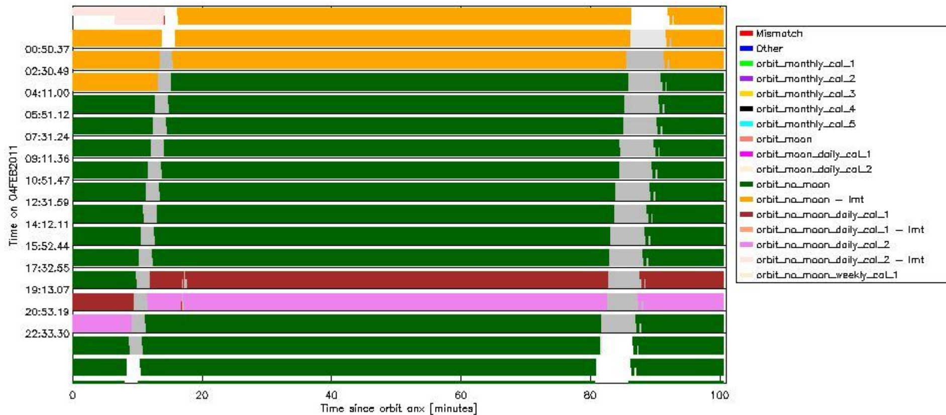
sciamachy_daily_report_level0_KSPT_L0_4504_N_20110204_6.PNG
