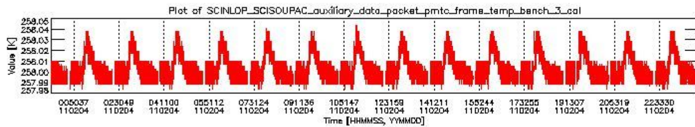
sciamachy_daily_report_level0_KSPT_L0_4504_N_20110204_2.PNG
