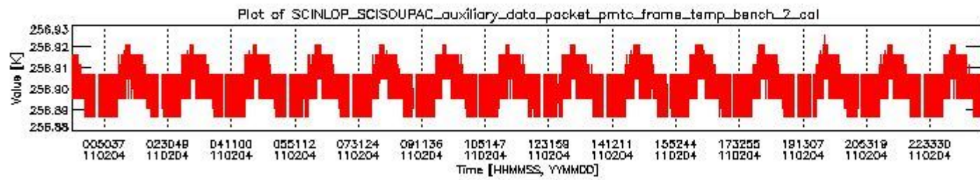
sciamachy_daily_report_level0_KSPT_L0_4504_N_20110204_1.PNG
