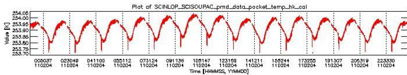
sciamachy_daily_report_level0_KSPT_L0_4504_N_20110204_3.PNG
