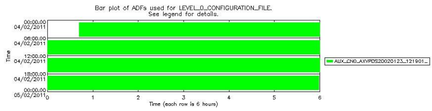
sciamachy_daily_report_level0_KSPT_L0_4504_N_20110204_7.PNG
