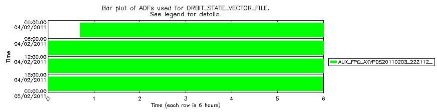
sciamachy_daily_report_level0_KSPT_L0_4504_N_20110204_8.PNG
