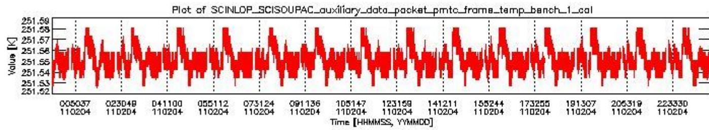
sciamachy_daily_report_level0_KSPT_L0_4504_N_20110204_0.PNG
