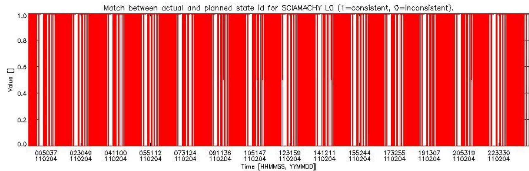
sciamachy_daily_report_level0_KSPT_L0_4504_N_20110204_5.PNG
