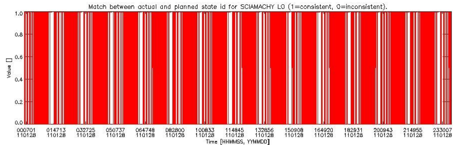
sciamachy_daily_report_level0_KSPT_L0_4504_N_20110128_5.PNG
