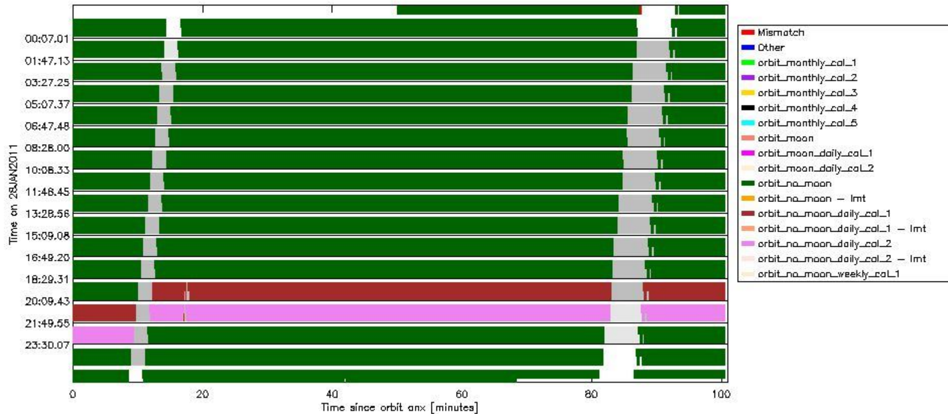
sciamachy_daily_report_level0_KSPT_L0_4504_N_20110128_6.PNG
