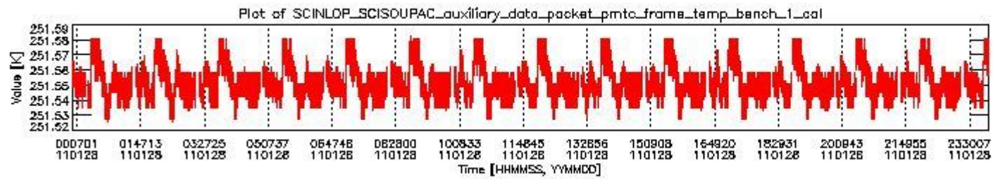
sciamachy_daily_report_level0_KSPT_L0_4504_N_20110128_0.PNG
