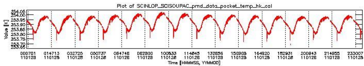
sciamachy_daily_report_level0_KSPT_L0_4504_N_20110128_3.PNG
