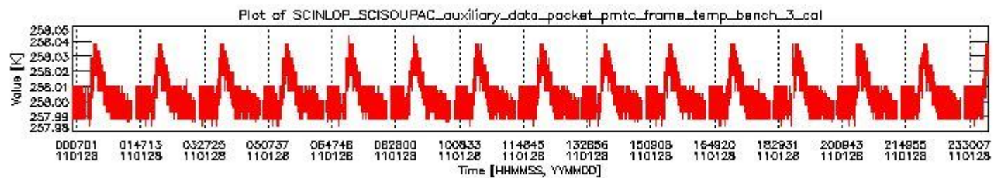
sciamachy_daily_report_level0_KSPT_L0_4504_N_20110128_2.PNG
