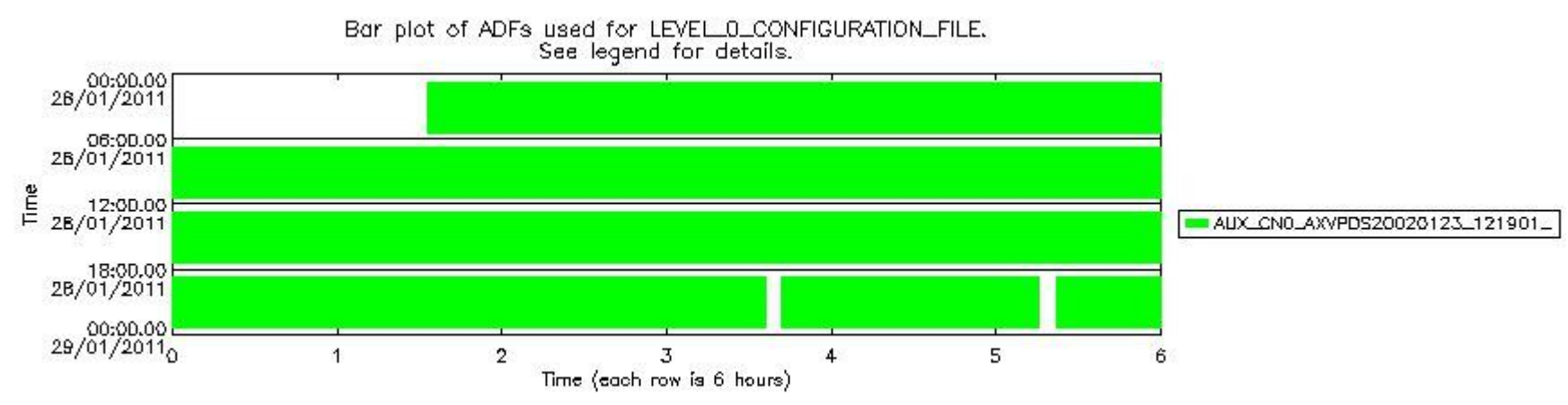
sciamachy_daily_report_level0_KSPT_L0_4504_N_20110128_7.PNG
