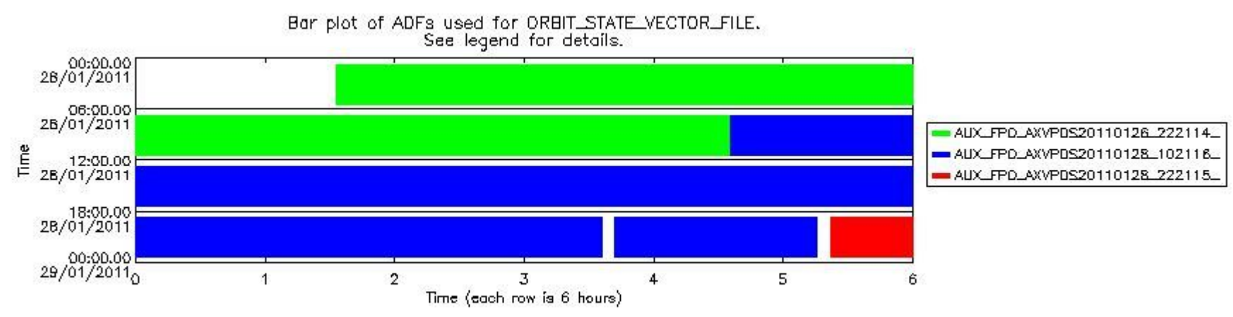
sciamachy_daily_report_level0_KSPT_L0_4504_N_20110128_8.PNG
