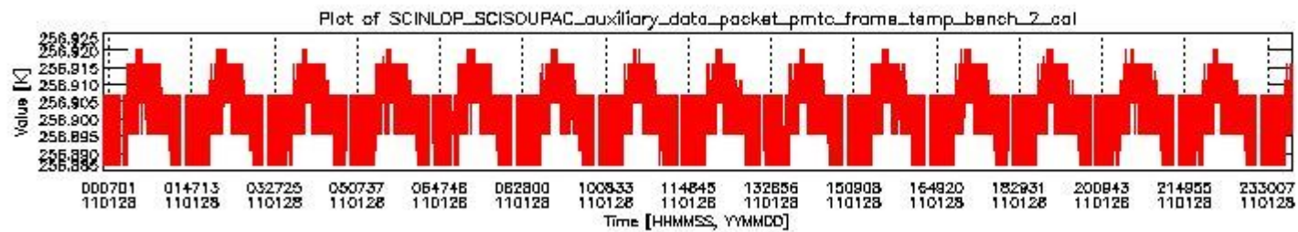
sciamachy_daily_report_level0_KSPT_L0_4504_N_20110128_1.PNG
