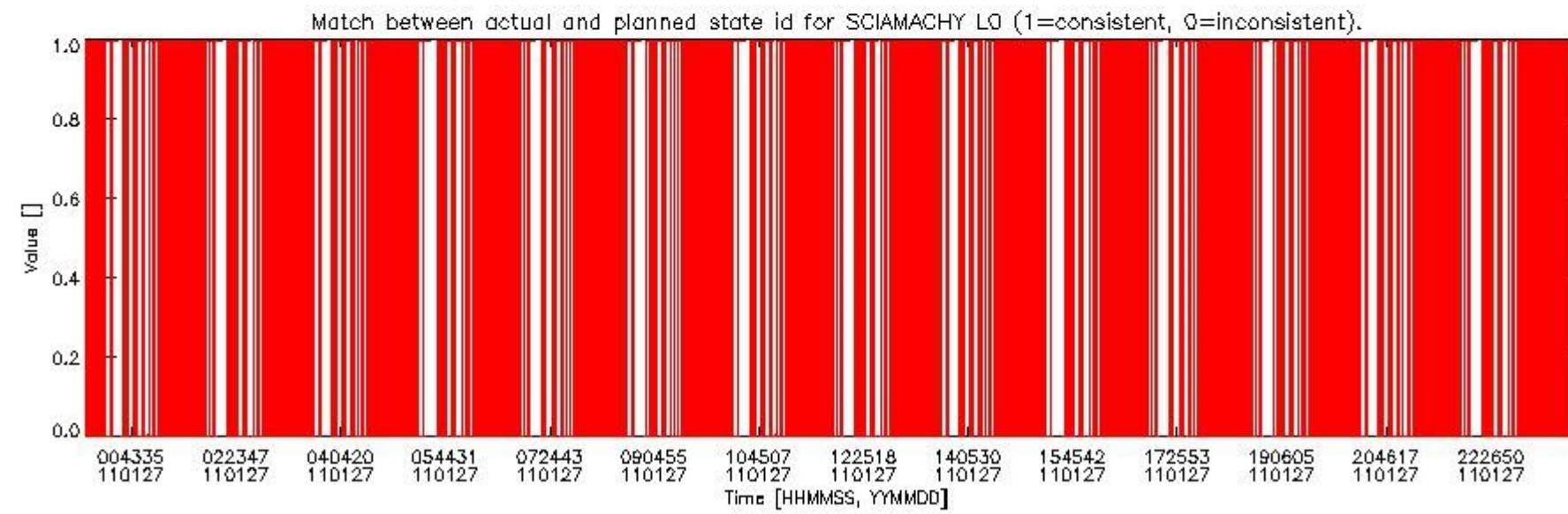
sciamachy_daily_report_level0_KSPT_L0_4504_N_20110127_5.PNG
