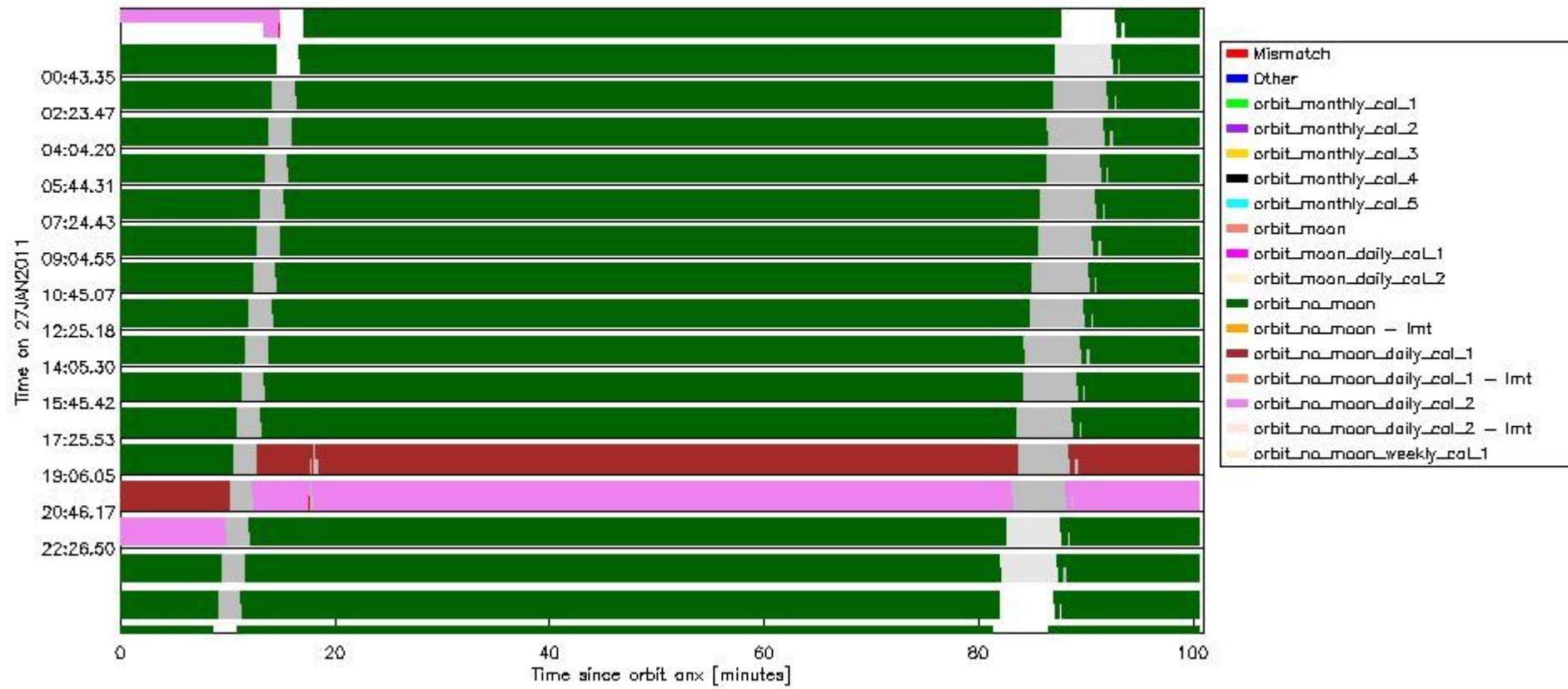
sciamachy_daily_report_level0_KSPT_L0_4504_N_20110127_6.PNG
