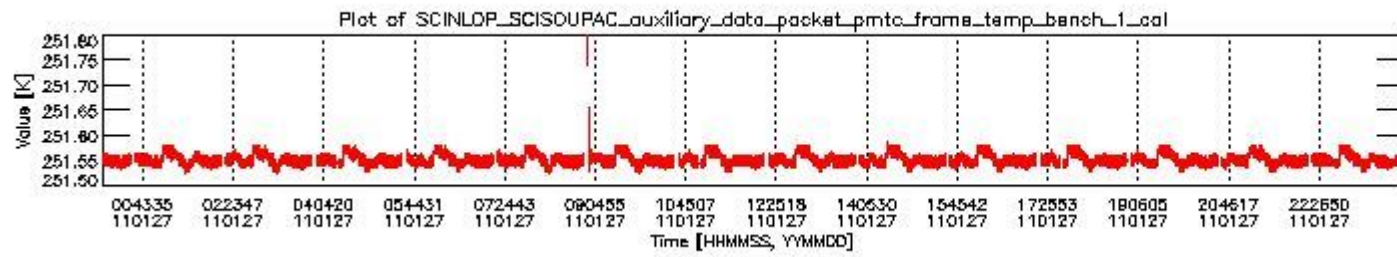
sciamachy_daily_report_level0_KSPT_L0_4504_N_20110127_0.PNG
