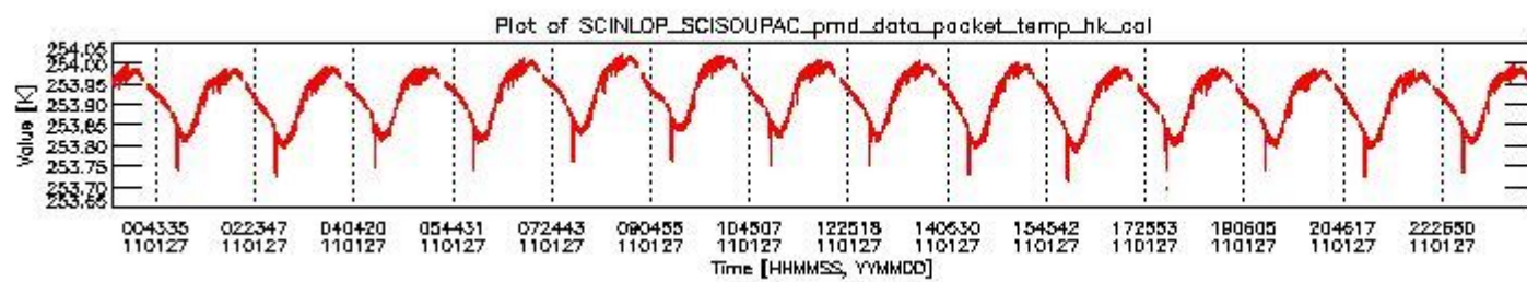
sciamachy_daily_report_level0_KSPT_L0_4504_N_20110127_3.PNG
