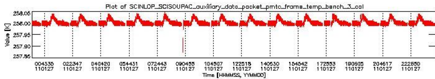
sciamachy_daily_report_level0_KSPT_L0_4504_N_20110127_2.PNG
