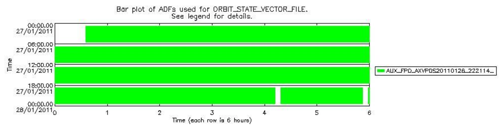
sciamachy_daily_report_level0_KSPT_L0_4504_N_20110127_8.PNG
