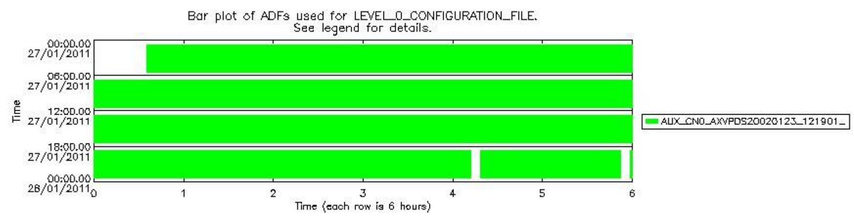
sciamachy_daily_report_level0_KSPT_L0_4504_N_20110127_7.PNG
