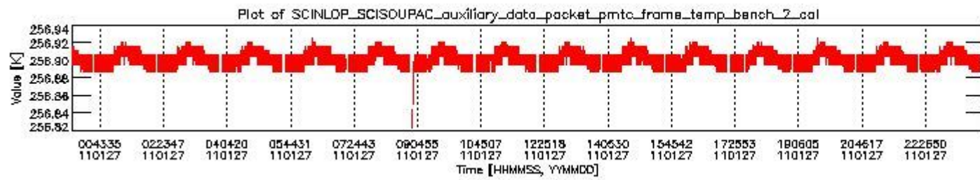
sciamachy_daily_report_level0_KSPT_L0_4504_N_20110127_1.PNG
