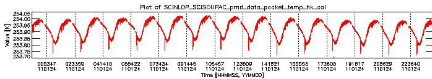
sciamachy_daily_report_level0_KSPT_L0_4504_N_20110124_3.PNG
