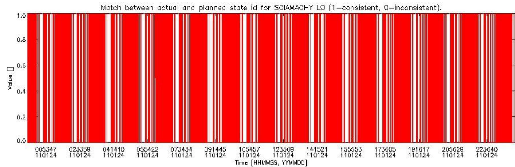
sciamachy_daily_report_level0_KSPT_L0_4504_N_20110124_5.PNG
