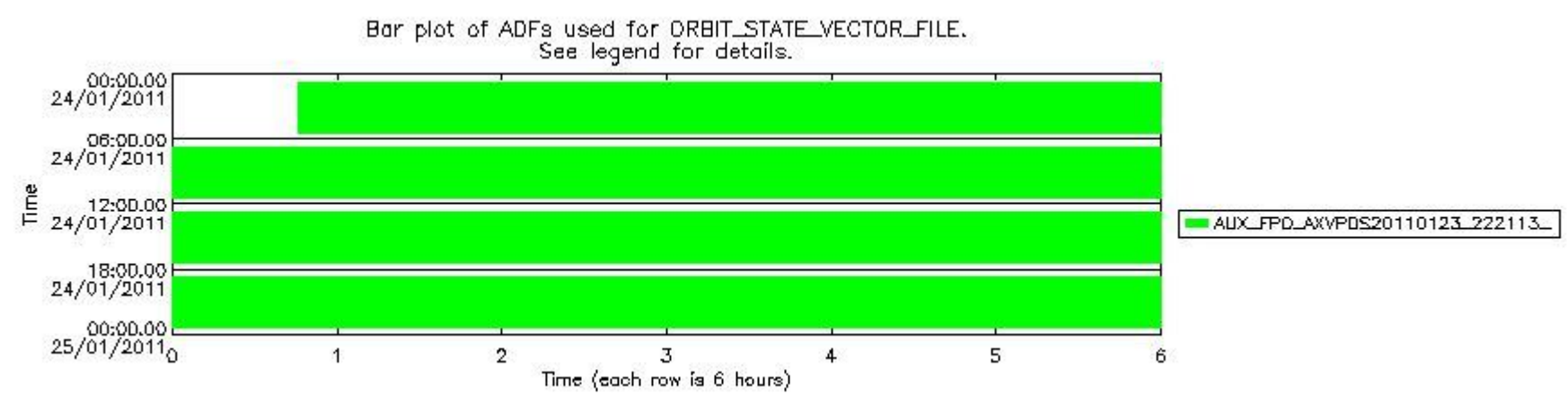
sciamachy_daily_report_level0_KSPT_L0_4504_N_20110124_8.PNG
