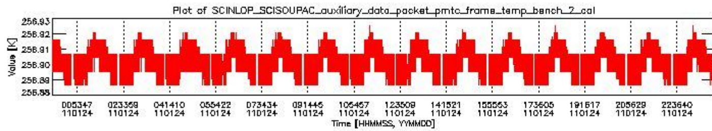
sciamachy_daily_report_level0_KSPT_L0_4504_N_20110124_1.PNG
