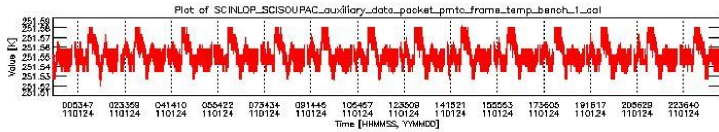
sciamachy_daily_report_level0_KSPT_L0_4504_N_20110124_0.PNG
