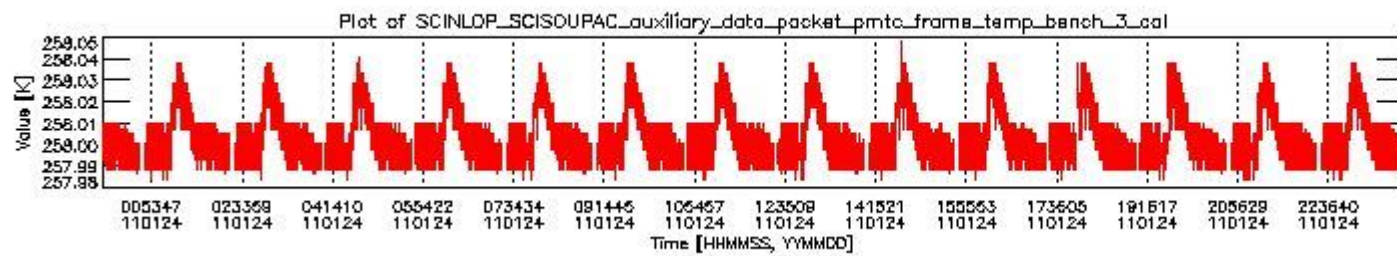
sciamachy_daily_report_level0_KSPT_L0_4504_N_20110124_2.PNG
