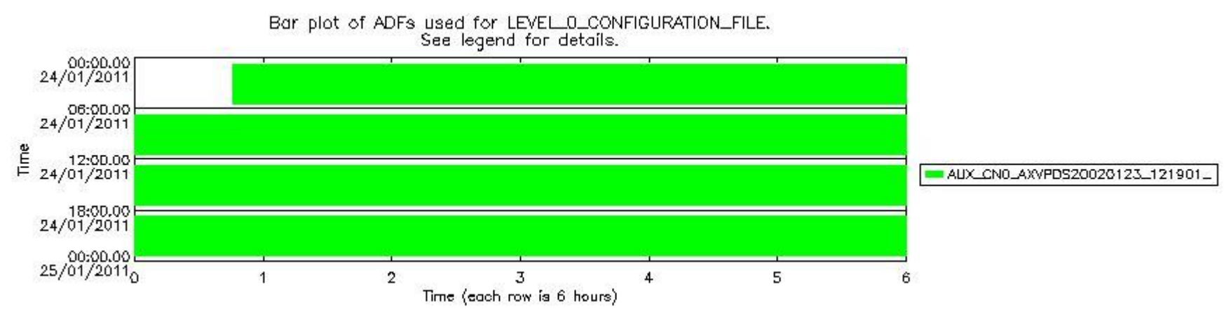
sciamachy_daily_report_level0_KSPT_L0_4504_N_20110124_7.PNG
