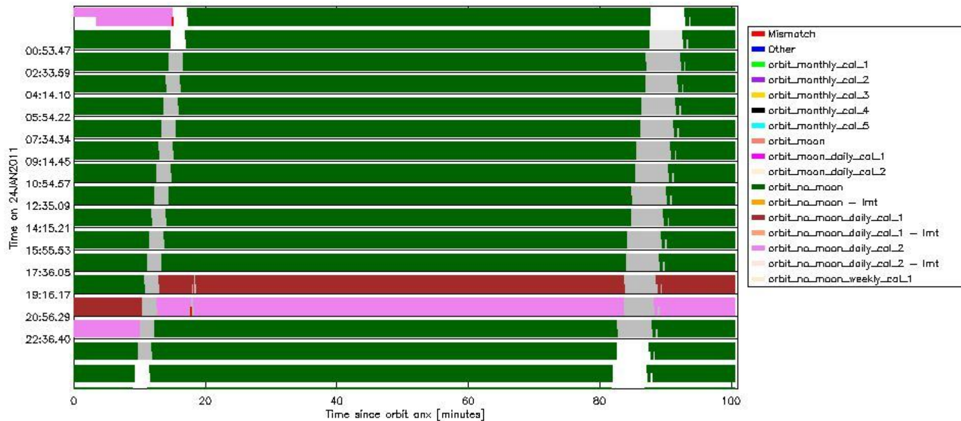
sciamachy_daily_report_level0_KSPT_L0_4504_N_20110124_6.PNG
