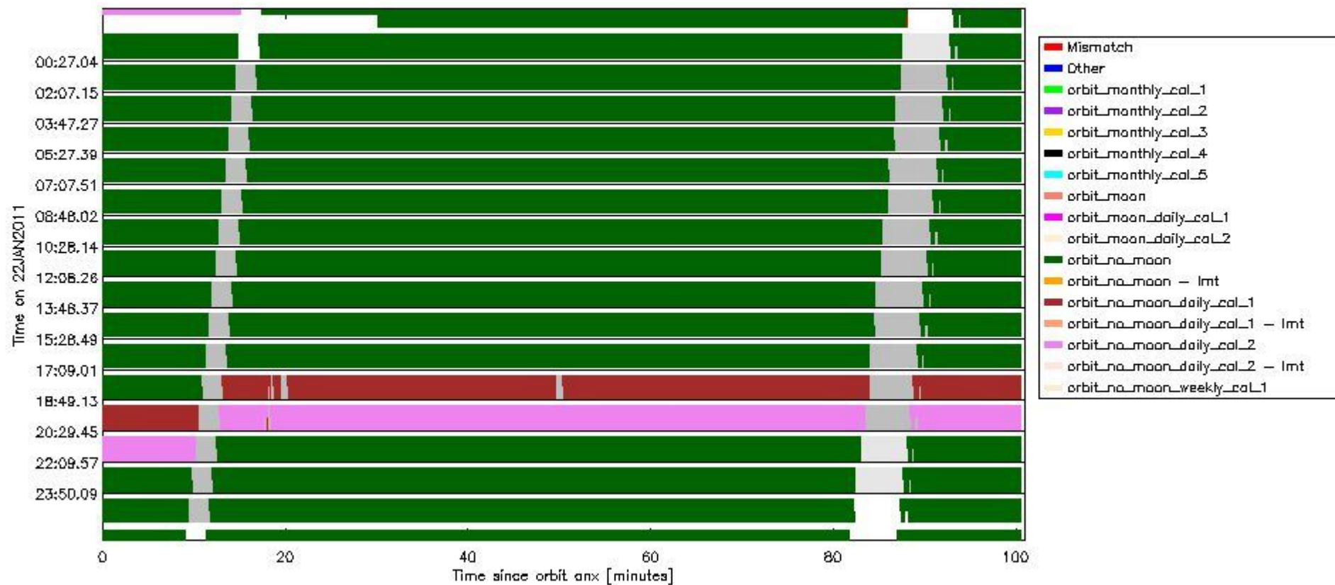
sciamachy_daily_report_level0_KSPT_L0_4504_N_20110122_6.PNG
