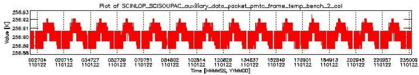
sciamachy_daily_report_level0_KSPT_L0_4504_N_20110122_1.PNG
