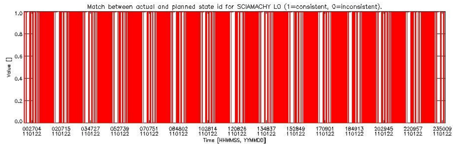
sciamachy_daily_report_level0_KSPT_L0_4504_N_20110122_5.PNG
