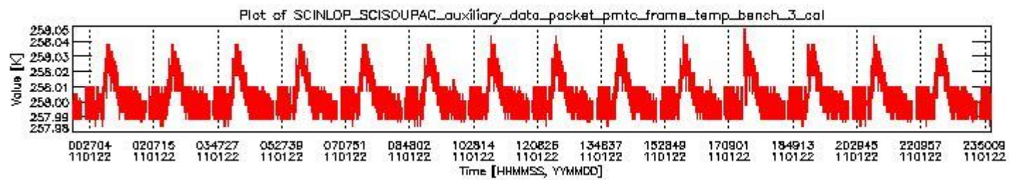
sciamachy_daily_report_level0_KSPT_L0_4504_N_20110122_2.PNG
