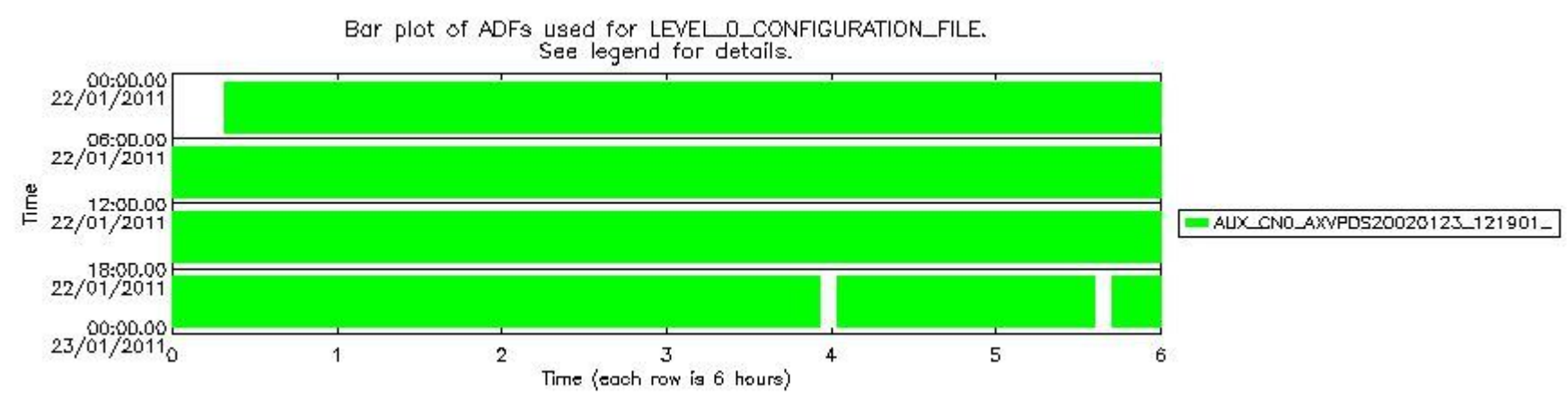
sciamachy_daily_report_level0_KSPT_L0_4504_N_20110122_7.PNG
