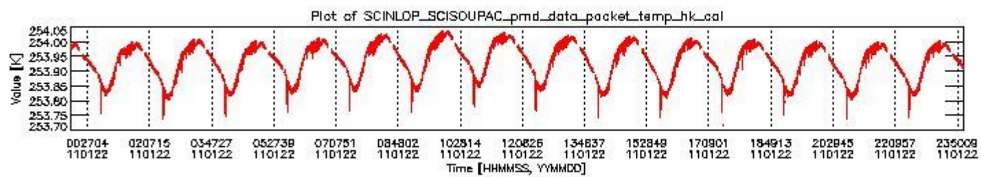
sciamachy_daily_report_level0_KSPT_L0_4504_N_20110122_3.PNG
