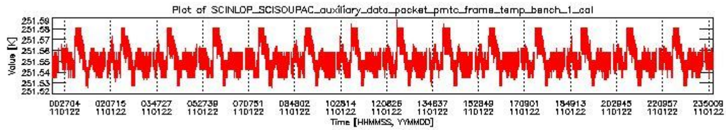
sciamachy_daily_report_level0_KSPT_L0_4504_N_20110122_0.PNG
