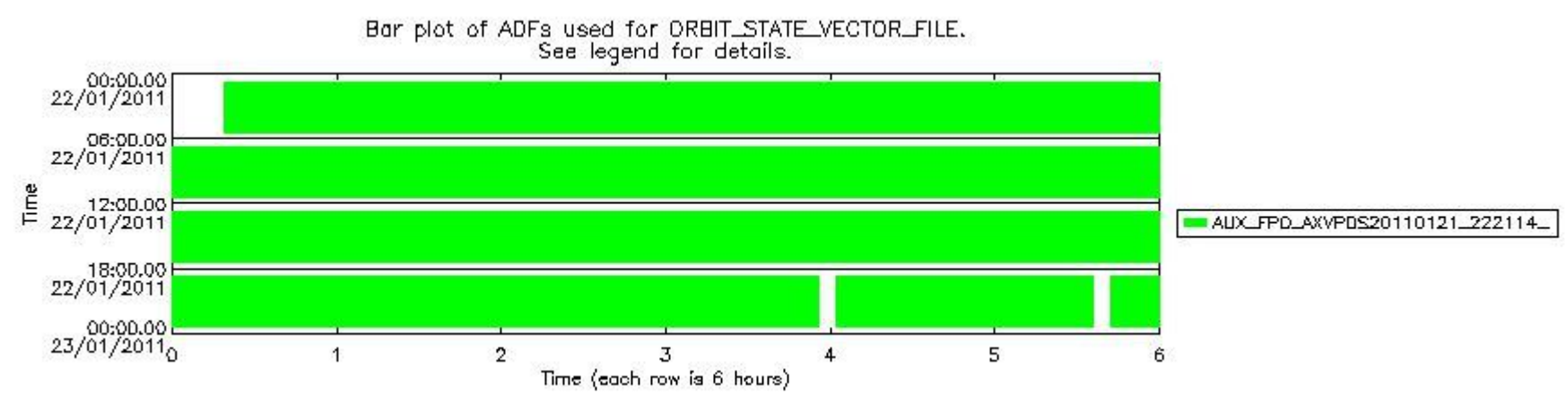
sciamachy_daily_report_level0_KSPT_L0_4504_N_20110122_8.PNG
