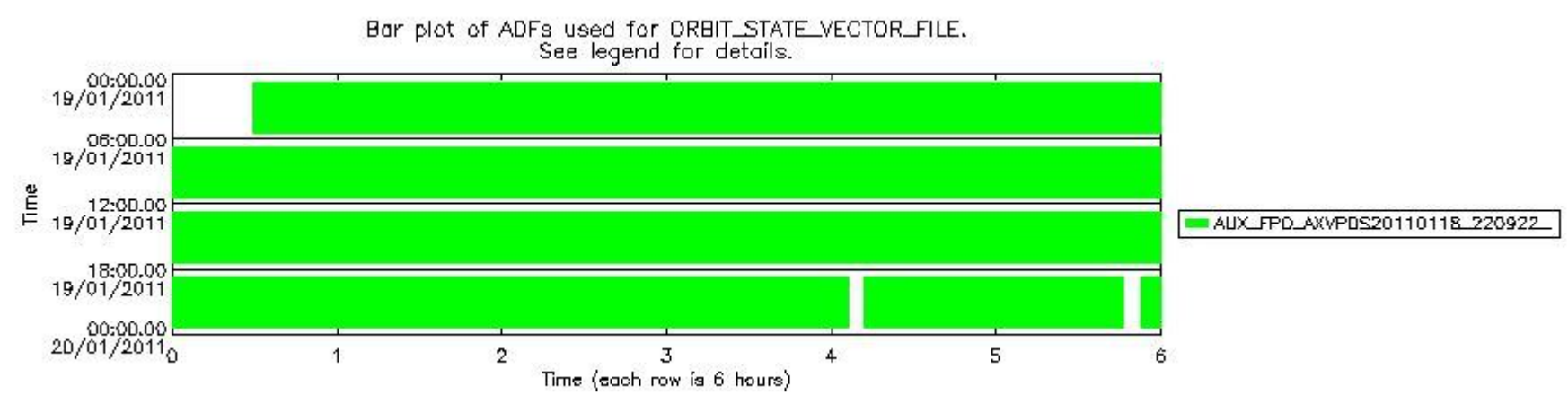
sciamachy_daily_report_level0_KSPT_L0_4504_N_20110119_8.PNG
