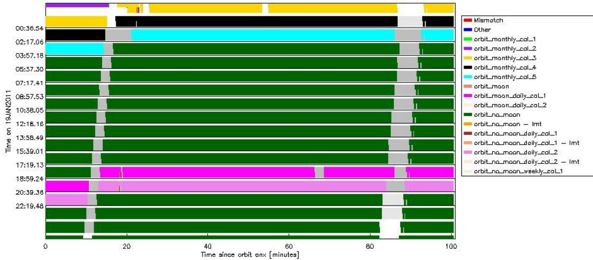
sciamachy_daily_report_level0_KSPT_L0_4504_N_20110119_6.PNG
