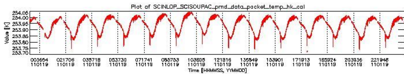
sciamachy_daily_report_level0_KSPT_L0_4504_N_20110119_3.PNG
