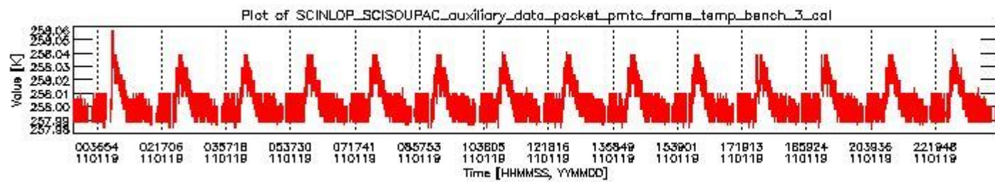
sciamachy_daily_report_level0_KSPT_L0_4504_N_20110119_2.PNG
