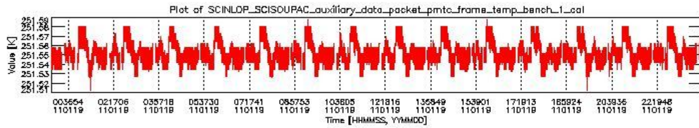
sciamachy_daily_report_level0_KSPT_L0_4504_N_20110119_0.PNG
