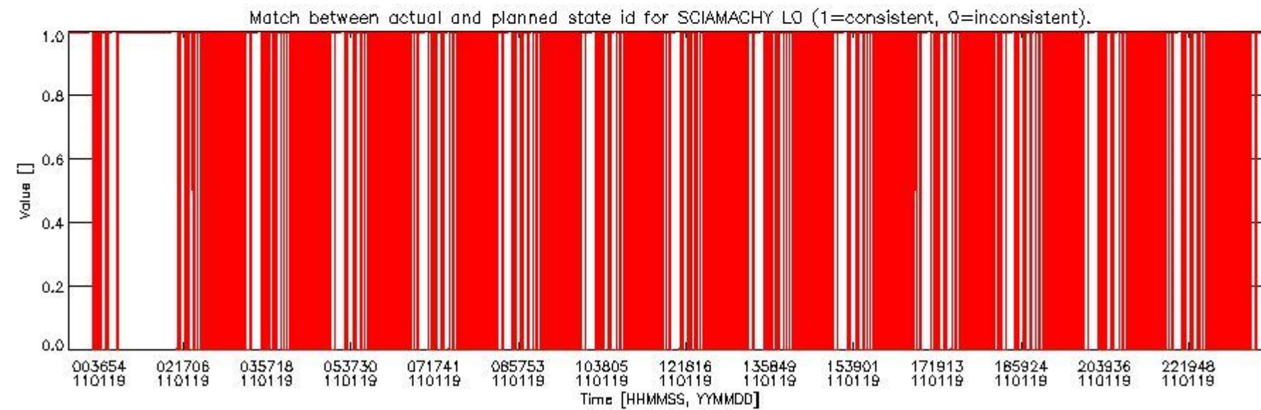
sciamachy_daily_report_level0_KSPT_L0_4504_N_20110119_5.PNG
