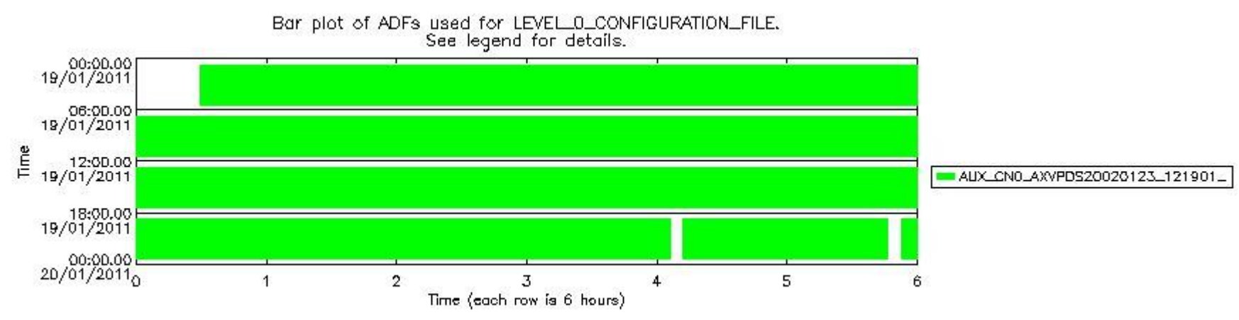
sciamachy_daily_report_level0_KSPT_L0_4504_N_20110119_7.PNG
