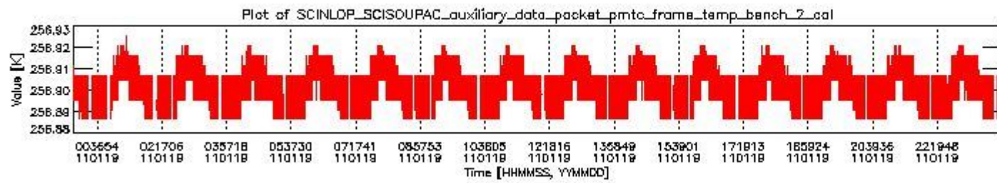
sciamachy_daily_report_level0_KSPT_L0_4504_N_20110119_1.PNG
