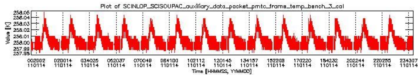
sciamachy_daily_report_level0_KSPT_L0_4504_N_20110114_2.PNG
