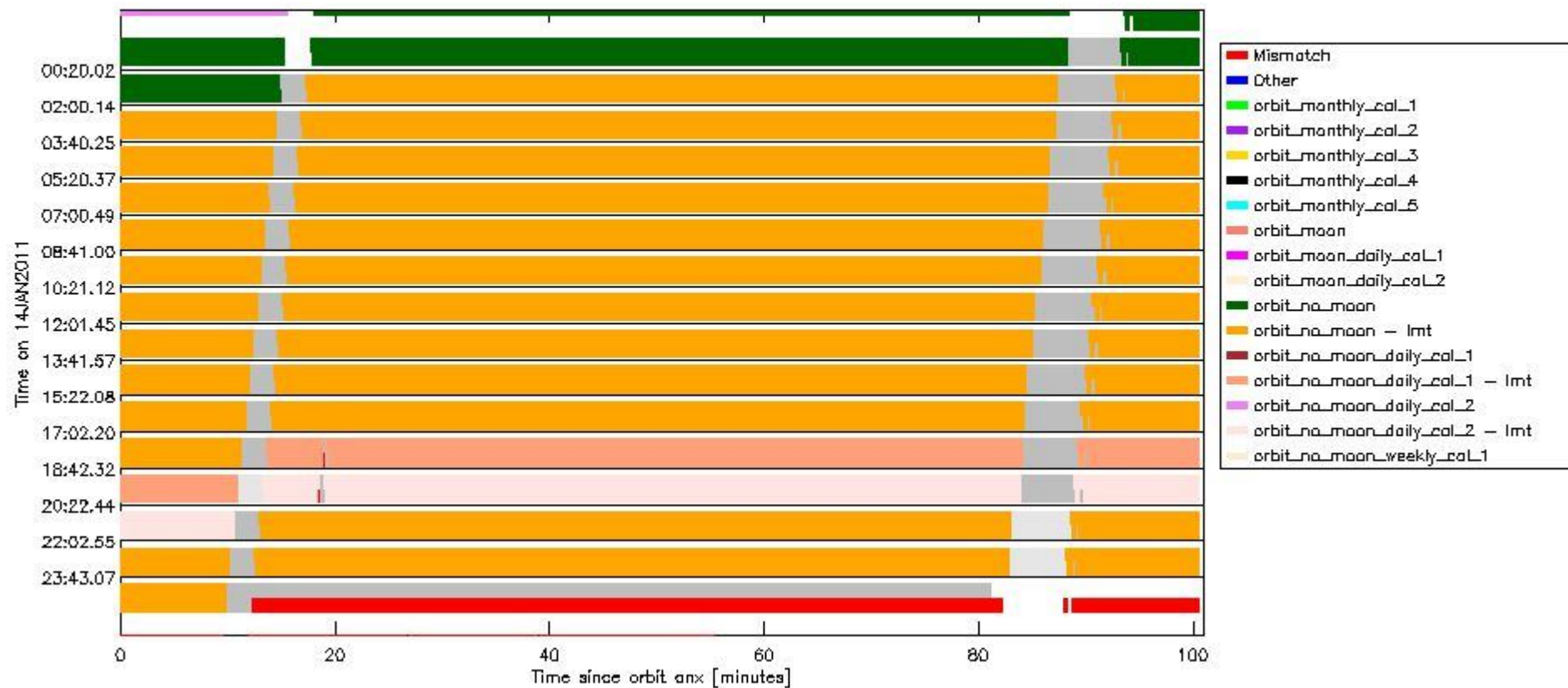
sciamachy_daily_report_level0_KSPT_L0_4504_N_20110114_6.PNG
