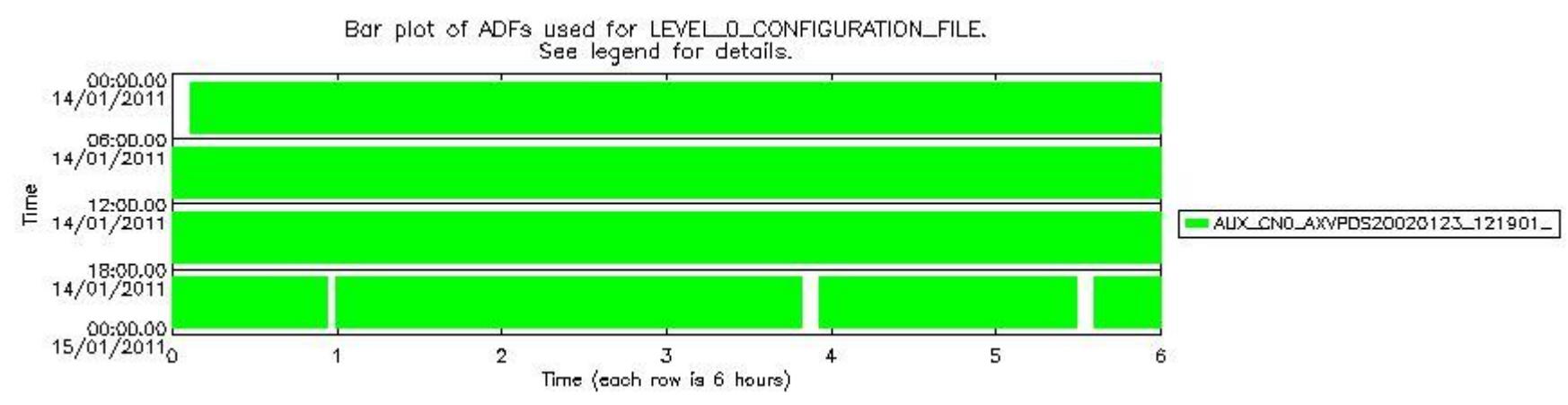
sciamachy_daily_report_level0_KSPT_L0_4504_N_20110114_7.PNG
