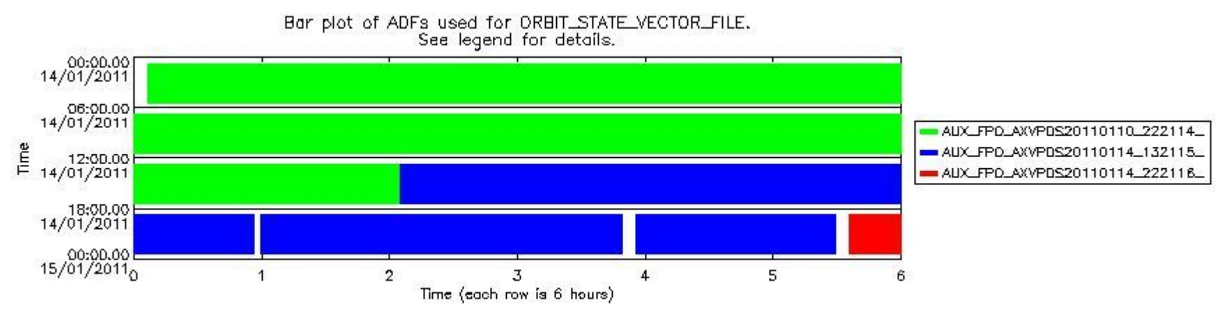
sciamachy_daily_report_level0_KSPT_L0_4504_N_20110114_8.PNG
