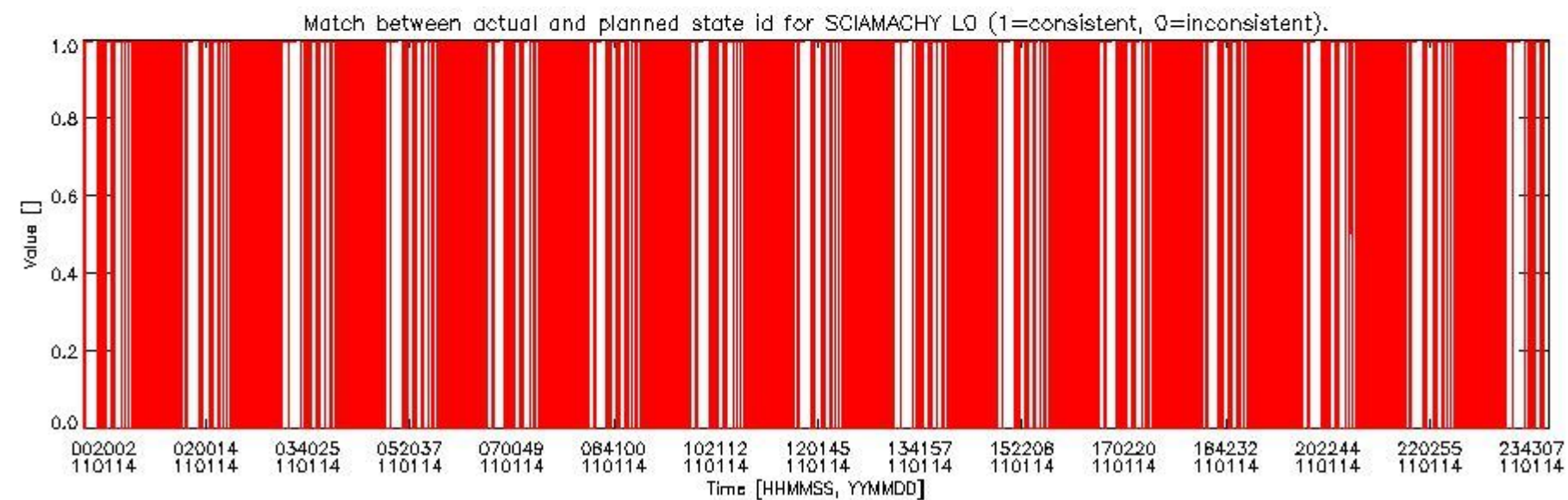
sciamachy_daily_report_level0_KSPT_L0_4504_N_20110114_5.PNG
