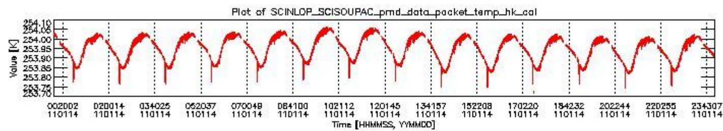
sciamachy_daily_report_level0_KSPT_L0_4504_N_20110114_3.PNG
