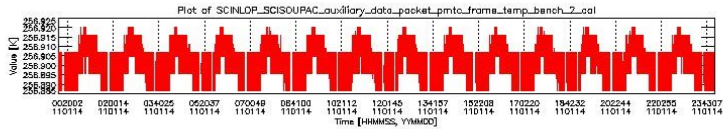
sciamachy_daily_report_level0_KSPT_L0_4504_N_20110114_1.PNG
