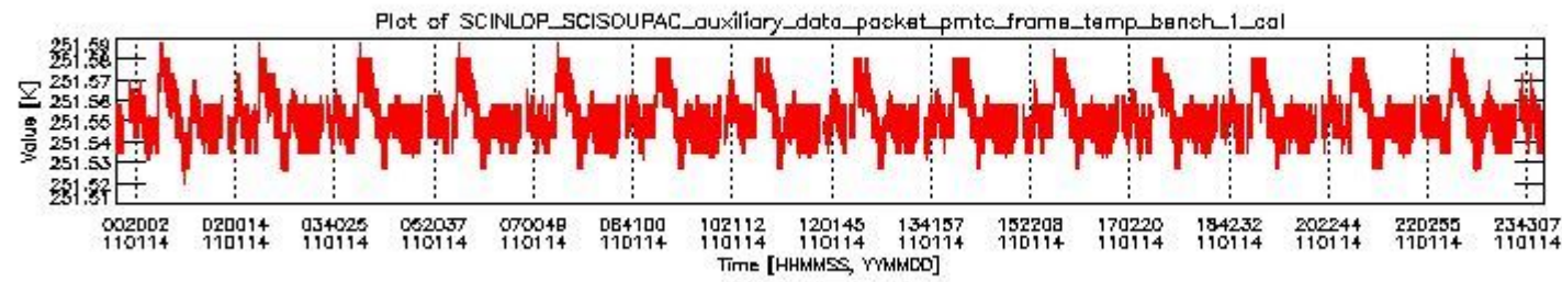
sciamachy_daily_report_level0_KSPT_L0_4504_N_20110114_0.PNG
