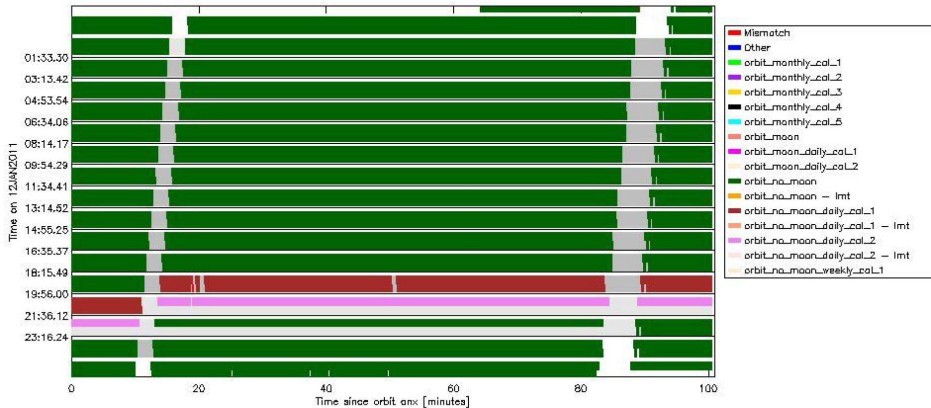
sciamachy_daily_report_level0_KSPT_L0_4504_N_20110112_6.PNG
