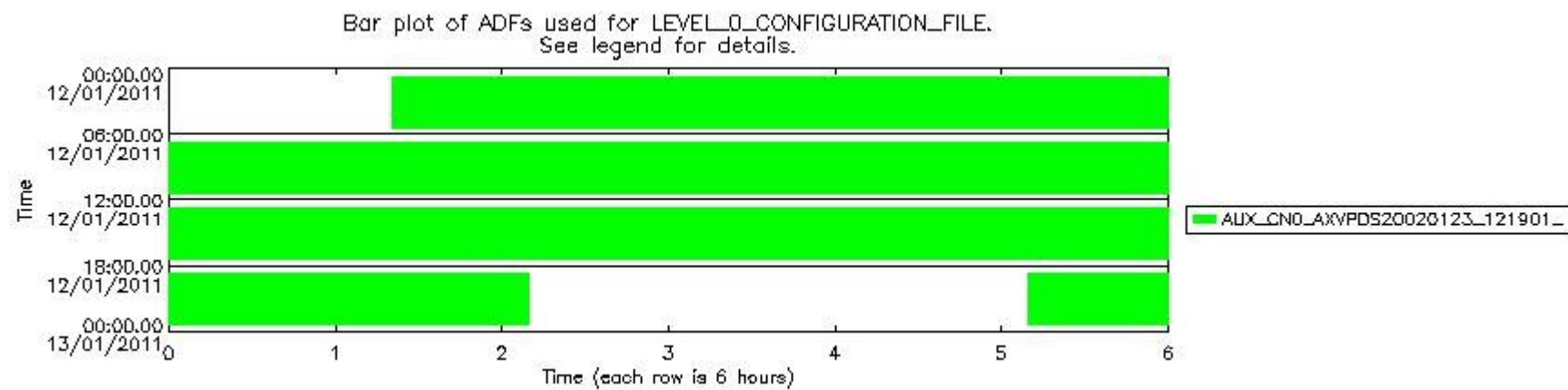
sciamachy_daily_report_level0_KSPT_L0_4504_N_20110112_7.PNG
