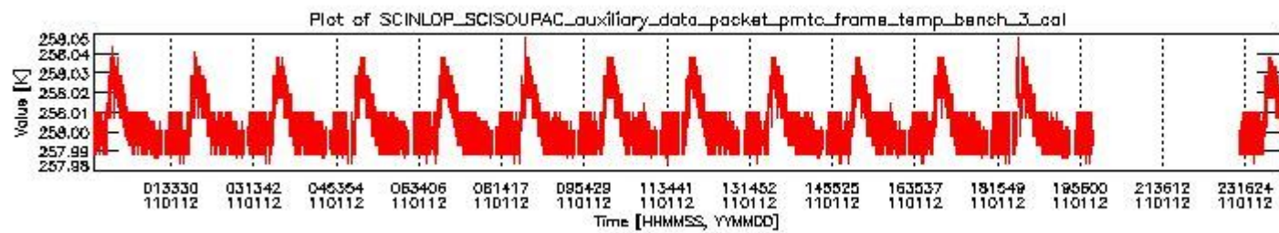
sciamachy_daily_report_level0_KSPT_L0_4504_N_20110112_2.PNG
