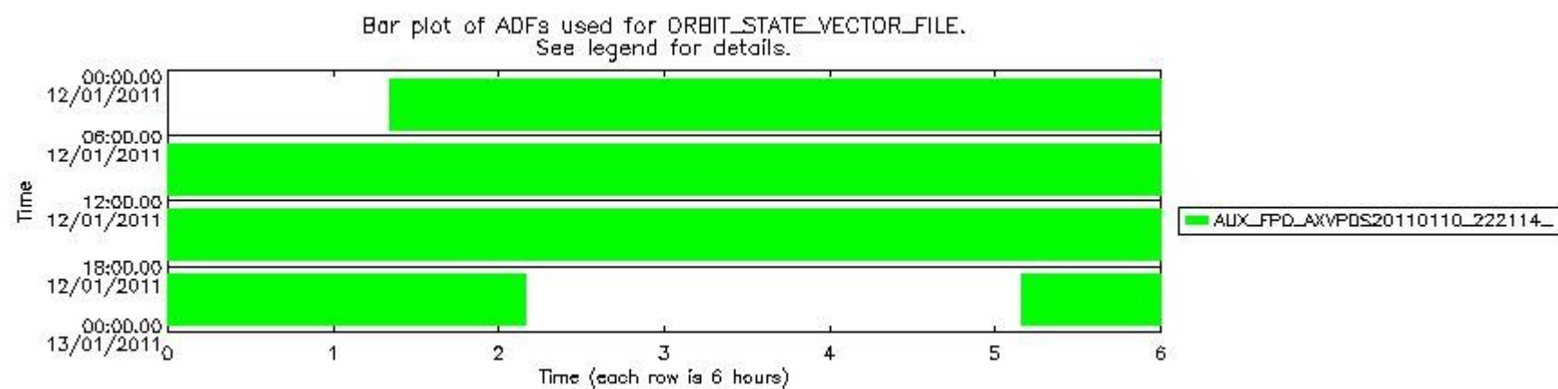
sciamachy_daily_report_level0_KSPT_L0_4504_N_20110112_8.PNG
