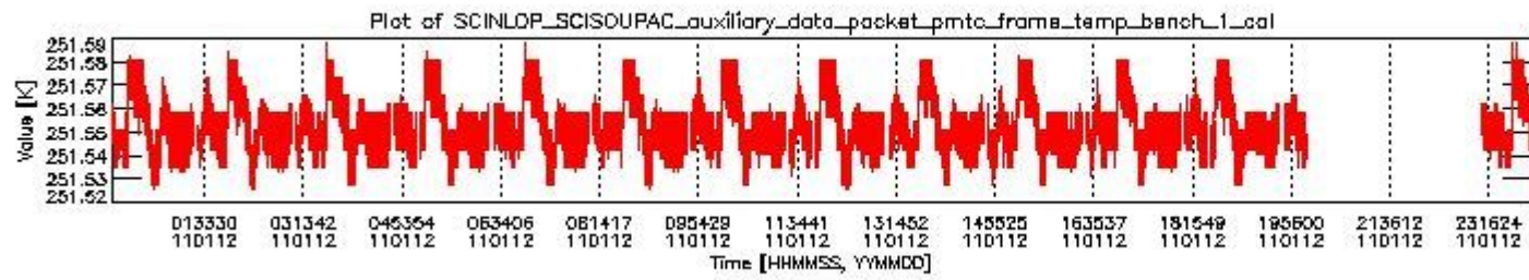
sciamachy_daily_report_level0_KSPT_L0_4504_N_20110112_0.PNG
