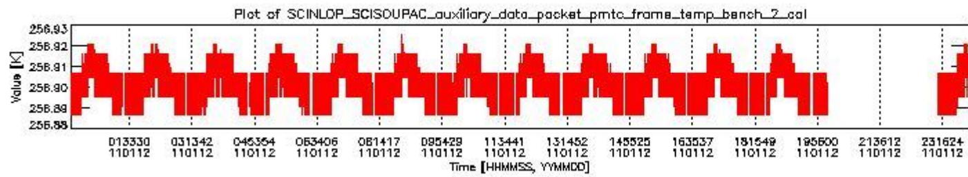
sciamachy_daily_report_level0_KSPT_L0_4504_N_20110112_1.PNG
