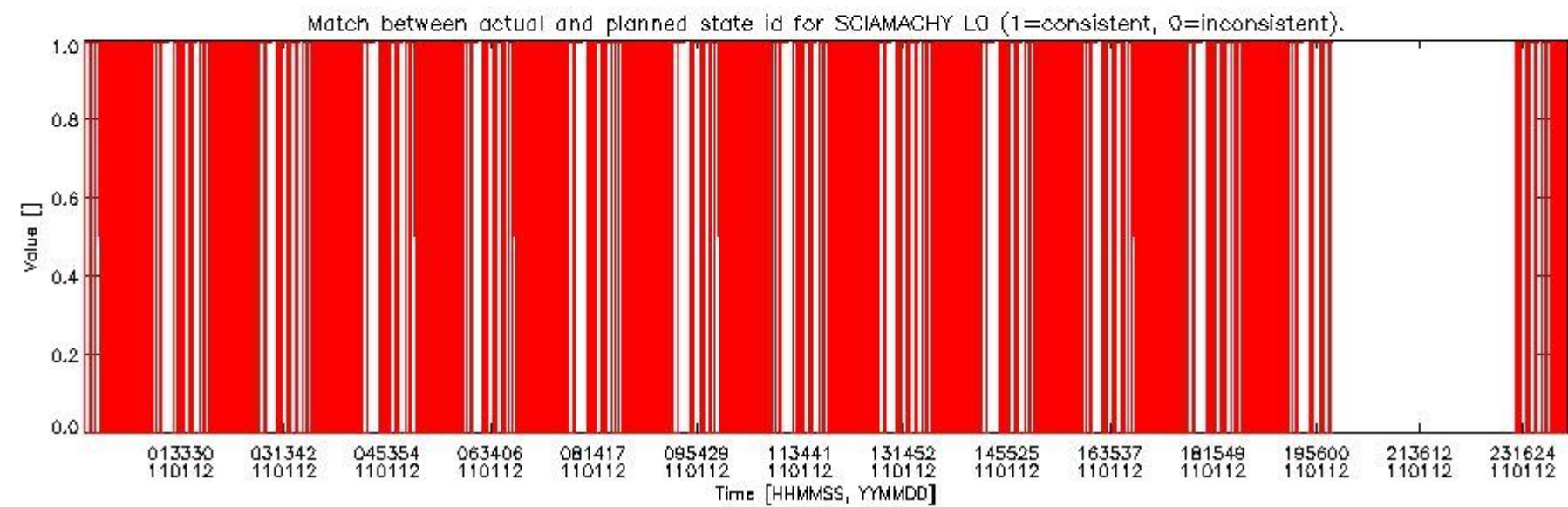
sciamachy_daily_report_level0_KSPT_L0_4504_N_20110112_5.PNG
