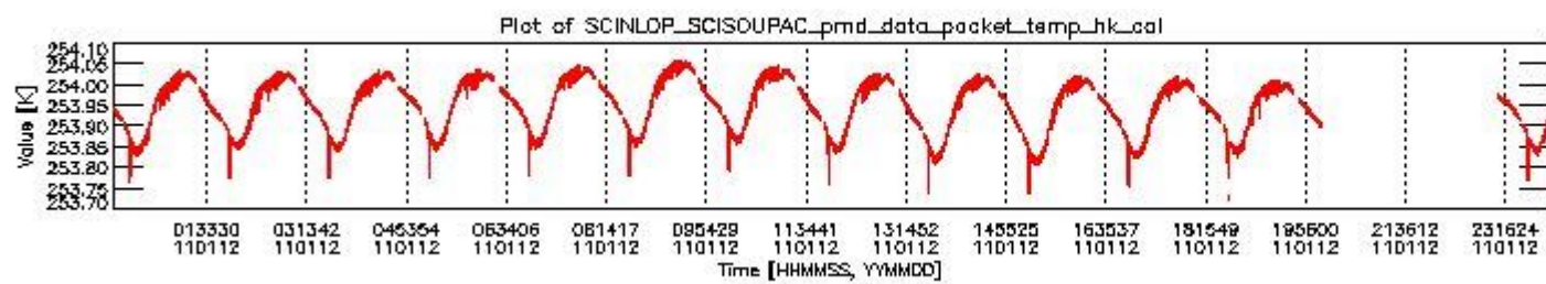
sciamachy_daily_report_level0_KSPT_L0_4504_N_20110112_3.PNG
