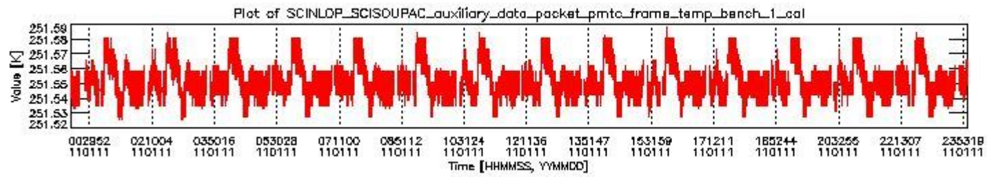
sciamachy_daily_report_level0_KSPT_L0_4504_N_20110111_0.PNG
