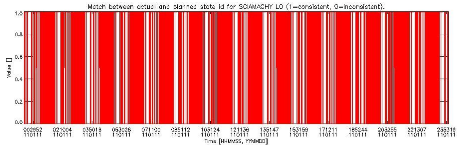
sciamachy_daily_report_level0_KSPT_L0_4504_N_20110111_5.PNG
