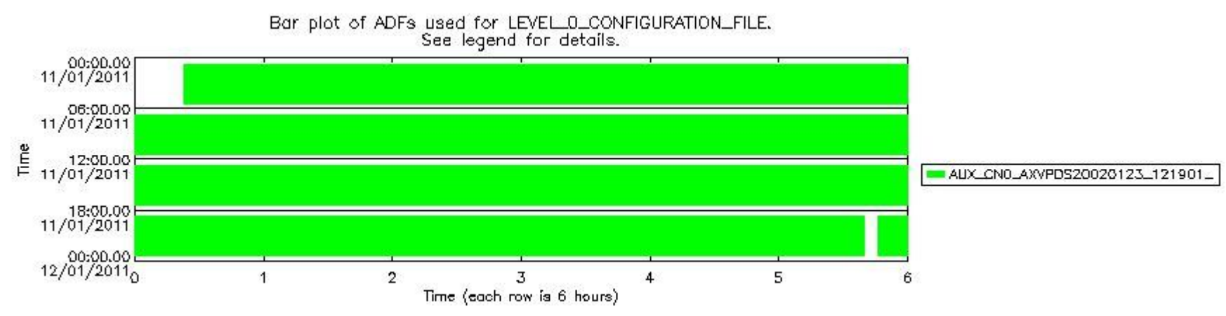
sciamachy_daily_report_level0_KSPT_L0_4504_N_20110111_7.PNG
