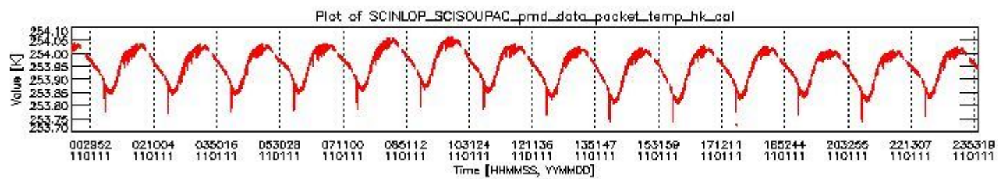
sciamachy_daily_report_level0_KSPT_L0_4504_N_20110111_3.PNG
