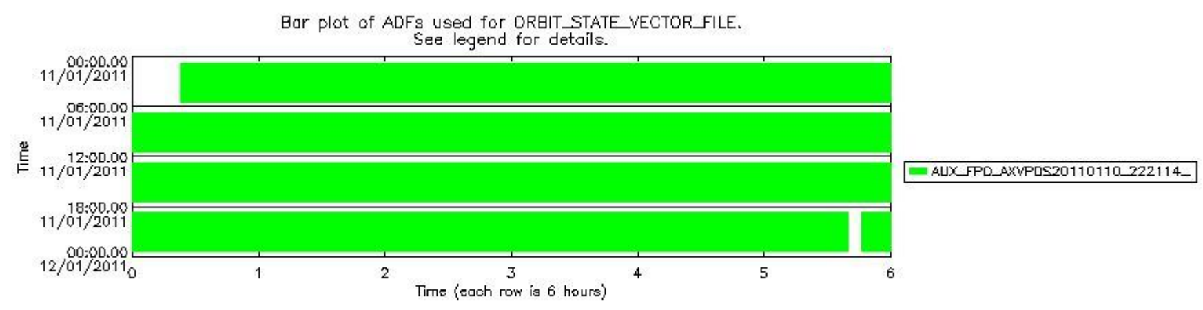
sciamachy_daily_report_level0_KSPT_L0_4504_N_20110111_8.PNG
