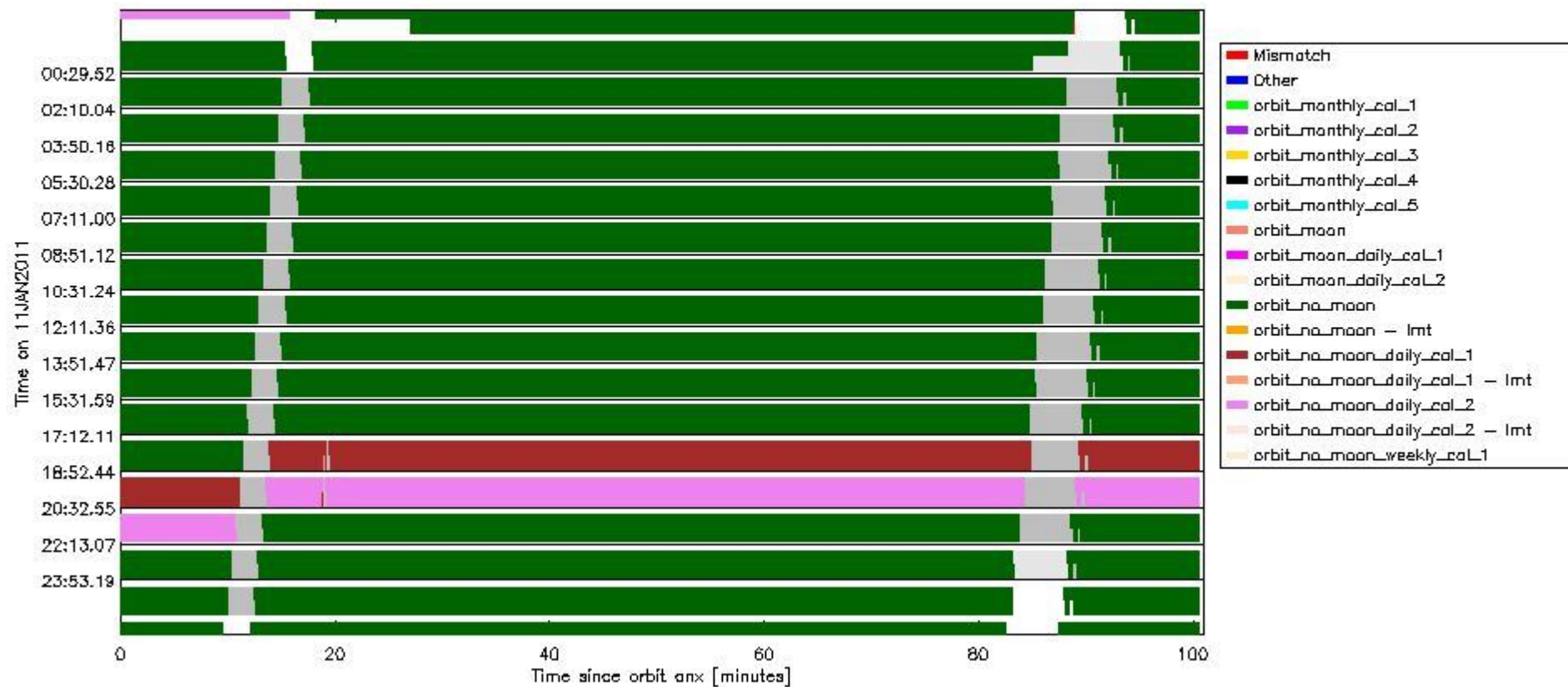
sciamachy_daily_report_level0_KSPT_L0_4504_N_20110111_6.PNG
