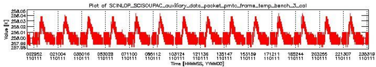
sciamachy_daily_report_level0_KSPT_L0_4504_N_20110111_2.PNG
