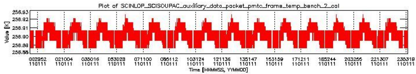
sciamachy_daily_report_level0_KSPT_L0_4504_N_20110111_1.PNG
