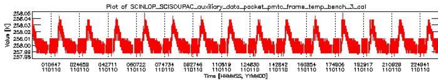
sciamachy_daily_report_level0_KSPT_L0_4504_N_20110110_2.PNG
