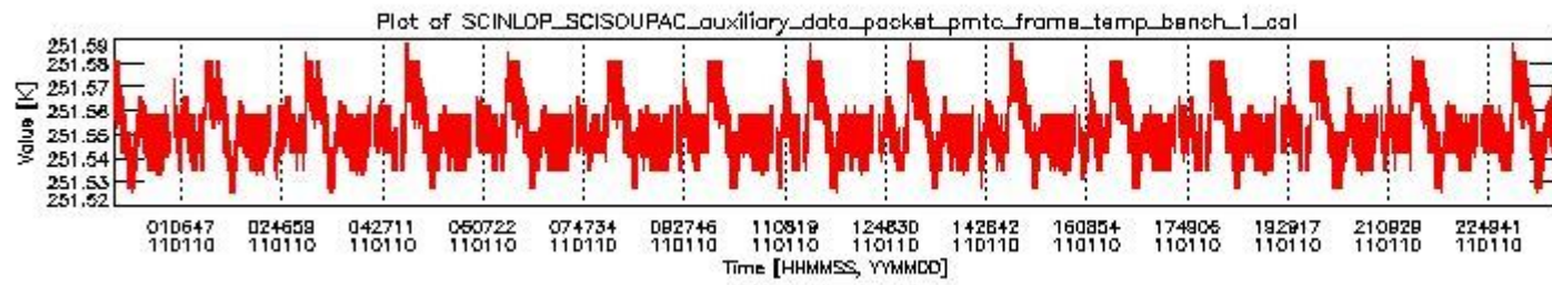
sciamachy_daily_report_level0_KSPT_L0_4504_N_20110110_0.PNG
