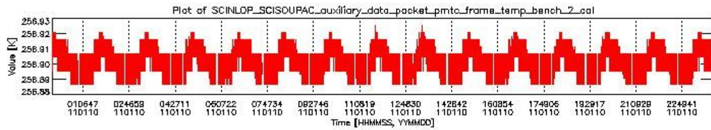
sciamachy_daily_report_level0_KSPT_L0_4504_N_20110110_1.PNG
