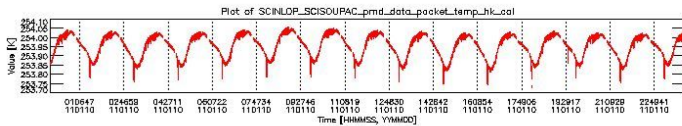
sciamachy_daily_report_level0_KSPT_L0_4504_N_20110110_3.PNG
