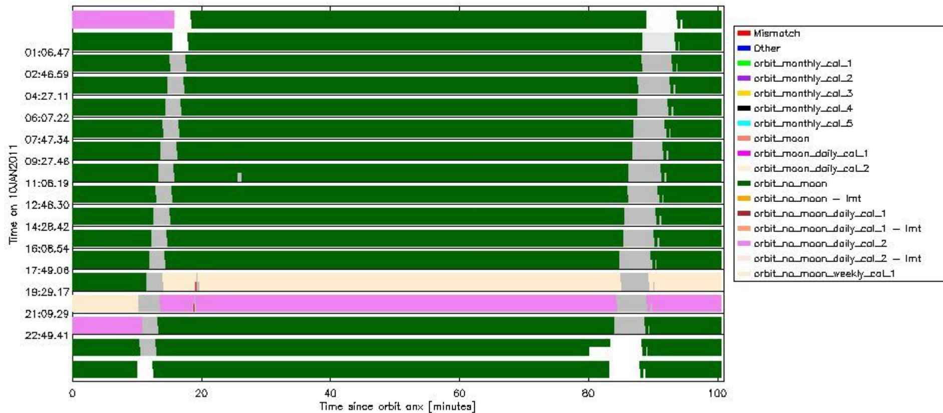
sciamachy_daily_report_level0_KSPT_L0_4504_N_20110110_6.PNG
