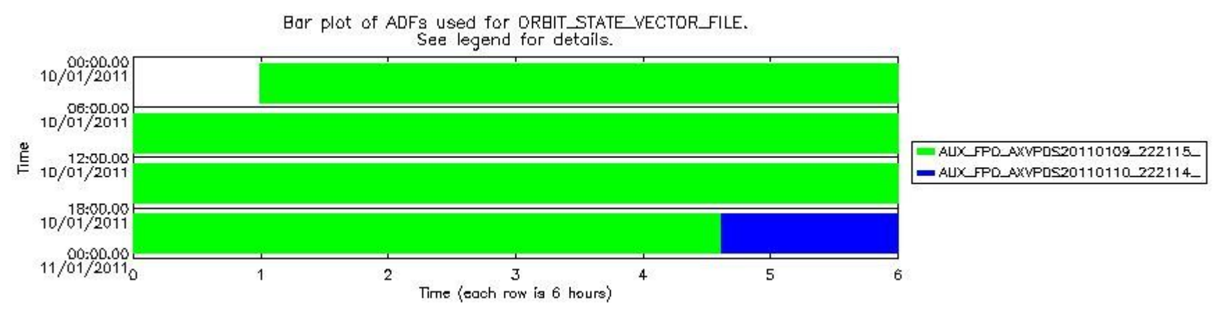
sciamachy_daily_report_level0_KSPT_L0_4504_N_20110110_8.PNG
