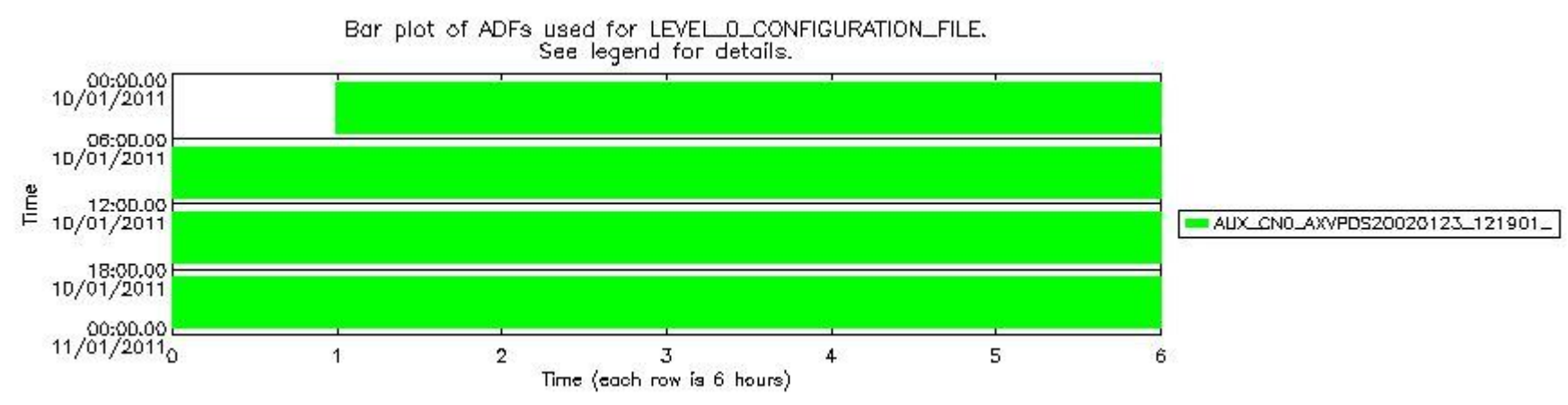
sciamachy_daily_report_level0_KSPT_L0_4504_N_20110110_7.PNG
