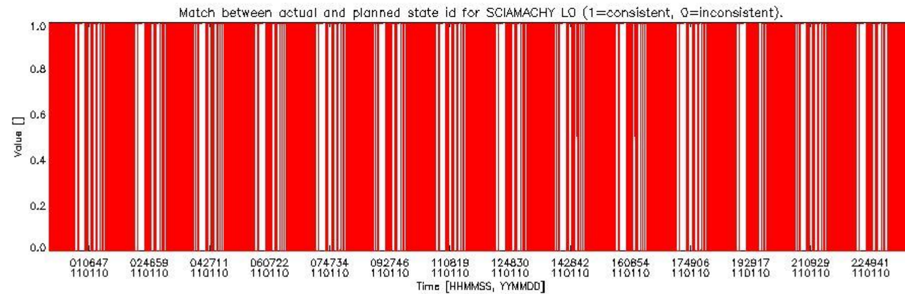
sciamachy_daily_report_level0_KSPT_L0_4504_N_20110110_5.PNG
