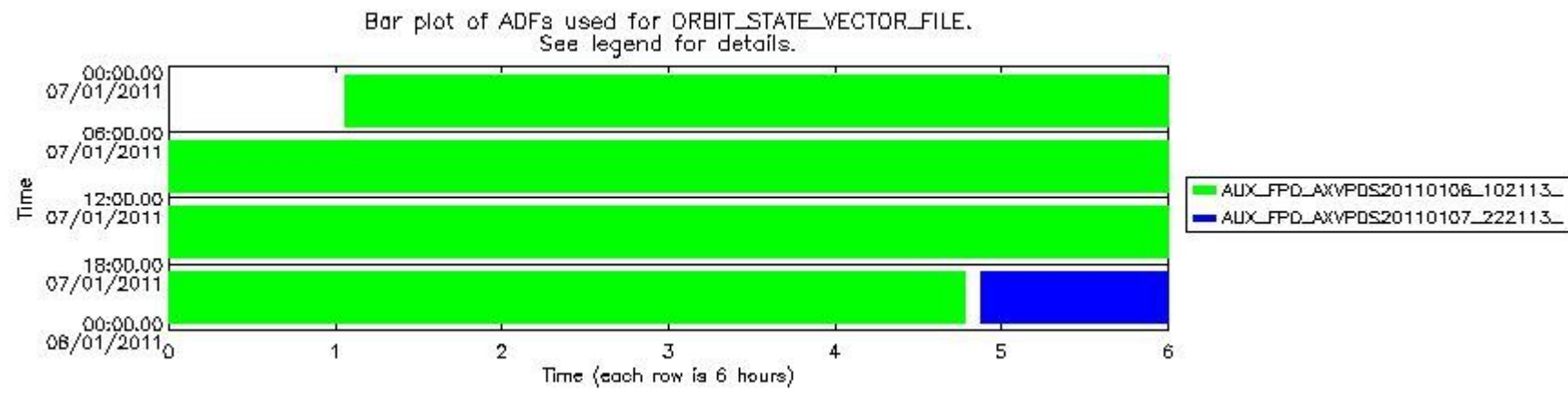
sciamachy_daily_report_level0_KSPT_L0_4504_N_20110107_8.PNG
