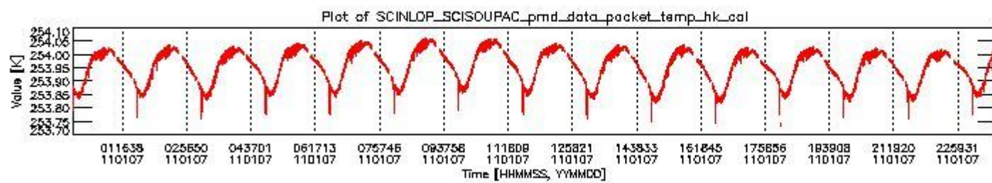
sciamachy_daily_report_level0_KSPT_L0_4504_N_20110107_3.PNG
