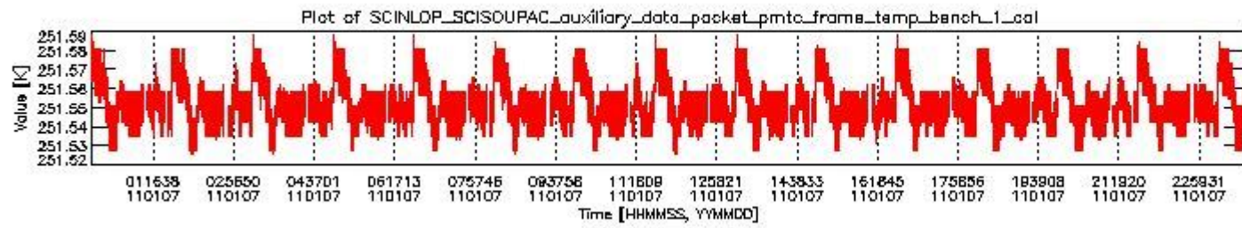
sciamachy_daily_report_level0_KSPT_L0_4504_N_20110107_0.PNG
