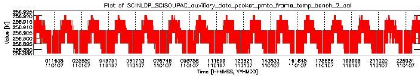
sciamachy_daily_report_level0_KSPT_L0_4504_N_20110107_1.PNG
