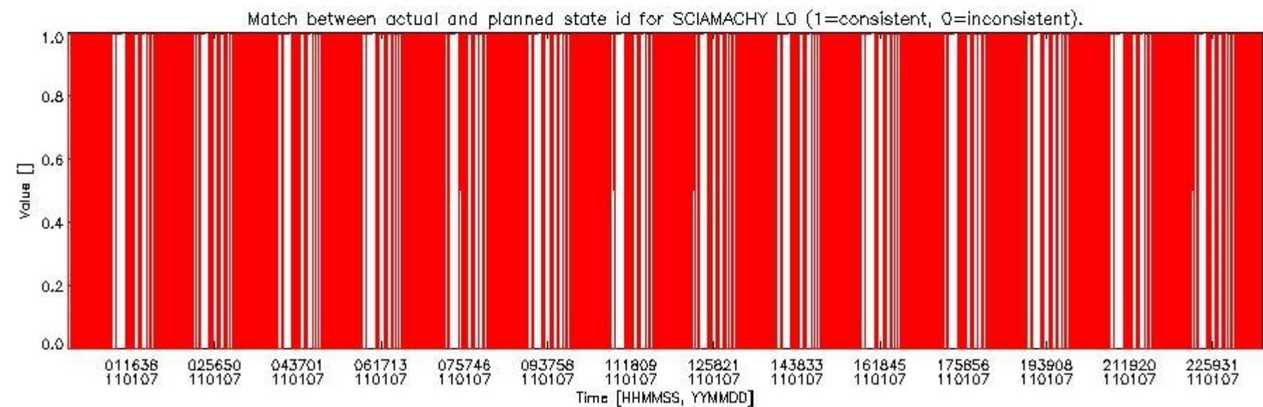
sciamachy_daily_report_level0_KSPT_L0_4504_N_20110107_5.PNG
