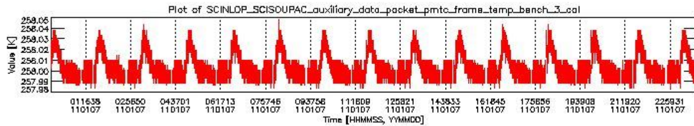
sciamachy_daily_report_level0_KSPT_L0_4504_N_20110107_2.PNG
