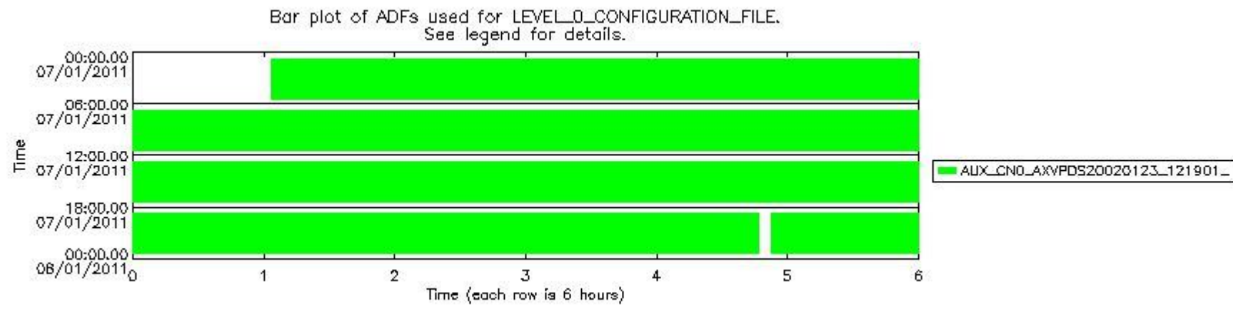
sciamachy_daily_report_level0_KSPT_L0_4504_N_20110107_7.PNG
