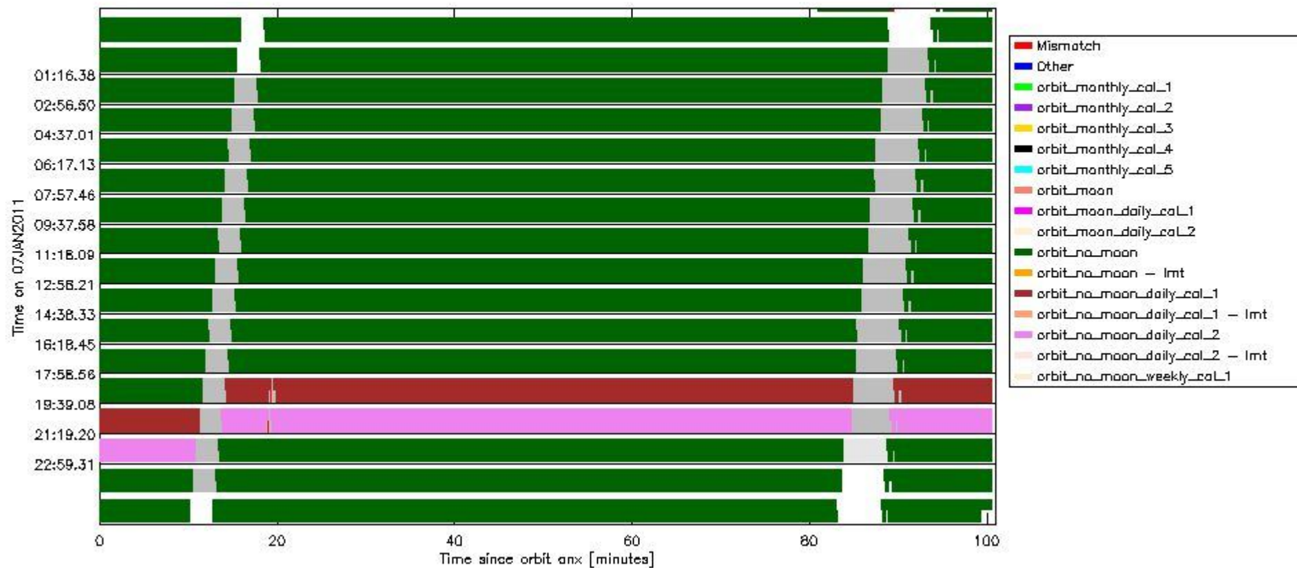
sciamachy_daily_report_level0_KSPT_L0_4504_N_20110107_6.PNG
