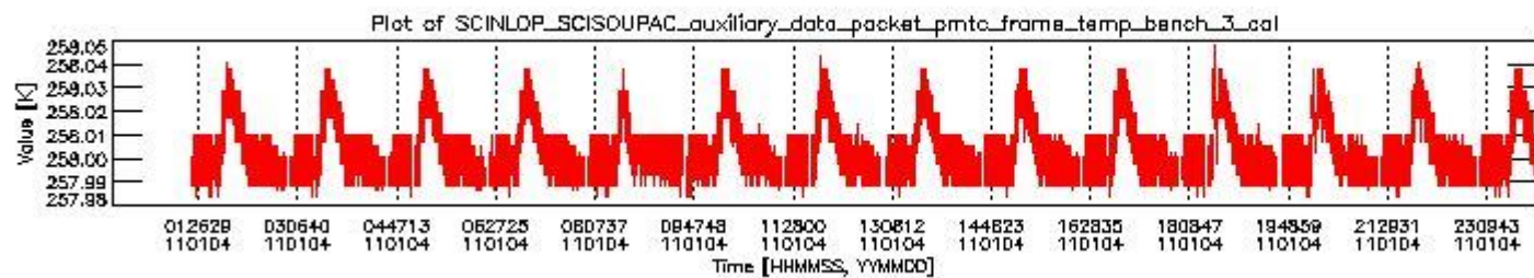
sciamachy_daily_report_level0_KSPT_L0_4504_N_20110104_2.PNG
