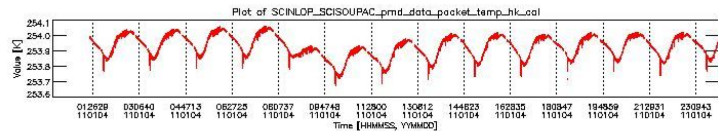
sciamachy_daily_report_level0_KSPT_L0_4504_N_20110104_3.PNG
