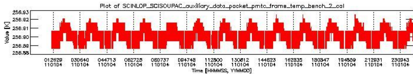
sciamachy_daily_report_level0_KSPT_L0_4504_N_20110104_1.PNG
