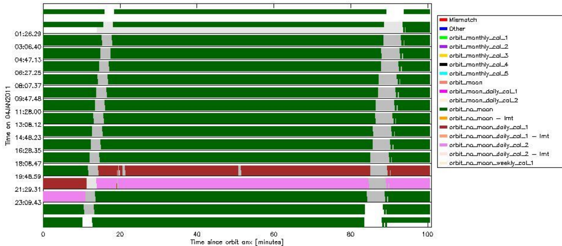
sciamachy_daily_report_level0_KSPT_L0_4504_N_20110104_6.PNG
