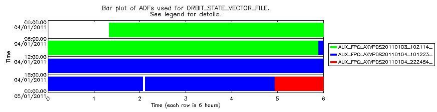
sciamachy_daily_report_level0_KSPT_L0_4504_N_20110104_8.PNG
