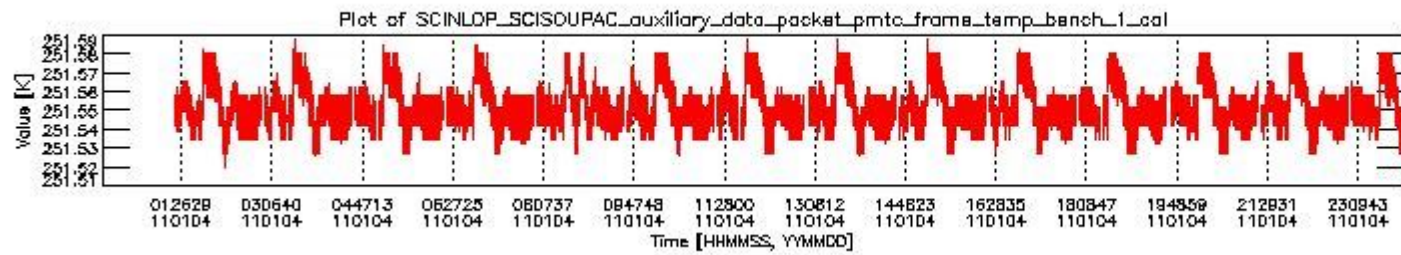
sciamachy_daily_report_level0_KSPT_L0_4504_N_20110104_0.PNG
