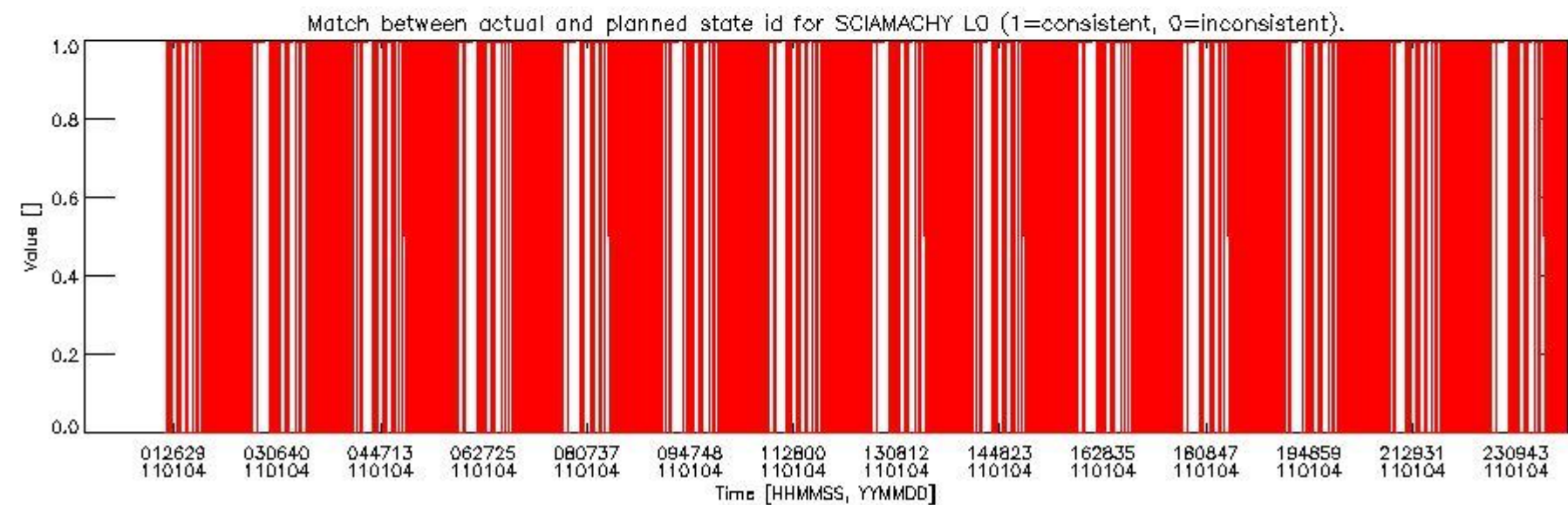
sciamachy_daily_report_level0_KSPT_L0_4504_N_20110104_5.PNG
