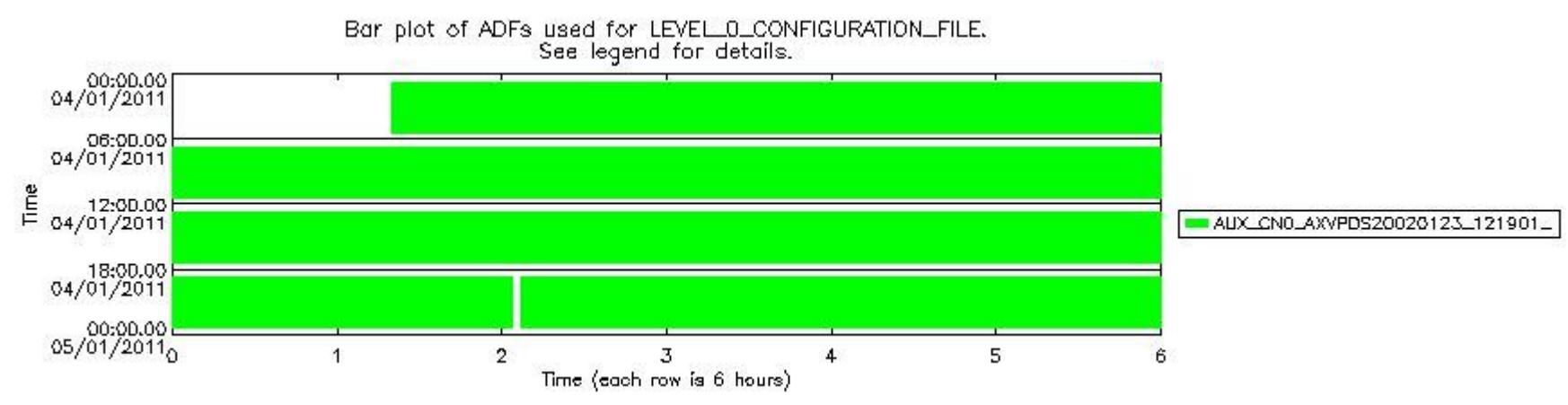
sciamachy_daily_report_level0_KSPT_L0_4504_N_20110104_7.PNG
