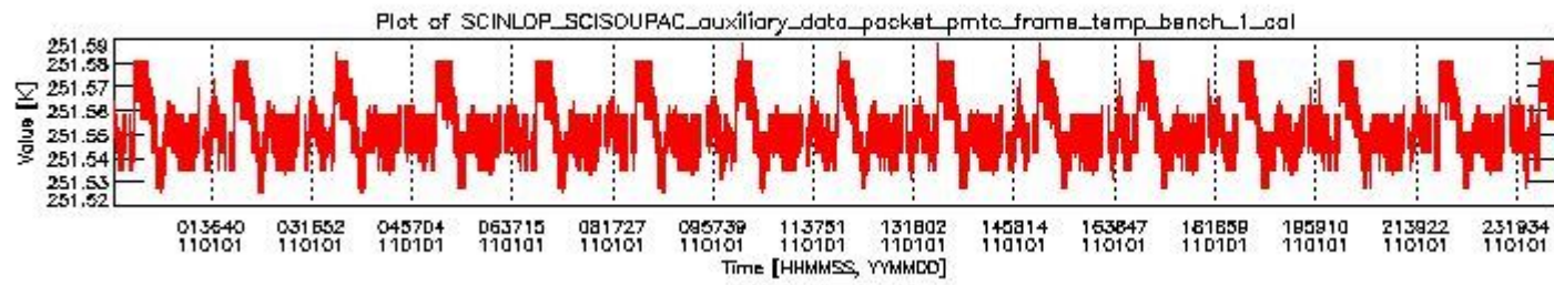
sciamachy_daily_report_level0_KSPT_L0_4504_N_20110101_0.PNG
