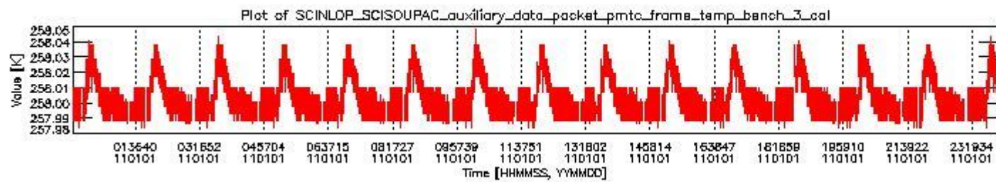
sciamachy_daily_report_level0_KSPT_L0_4504_N_20110101_2.PNG
