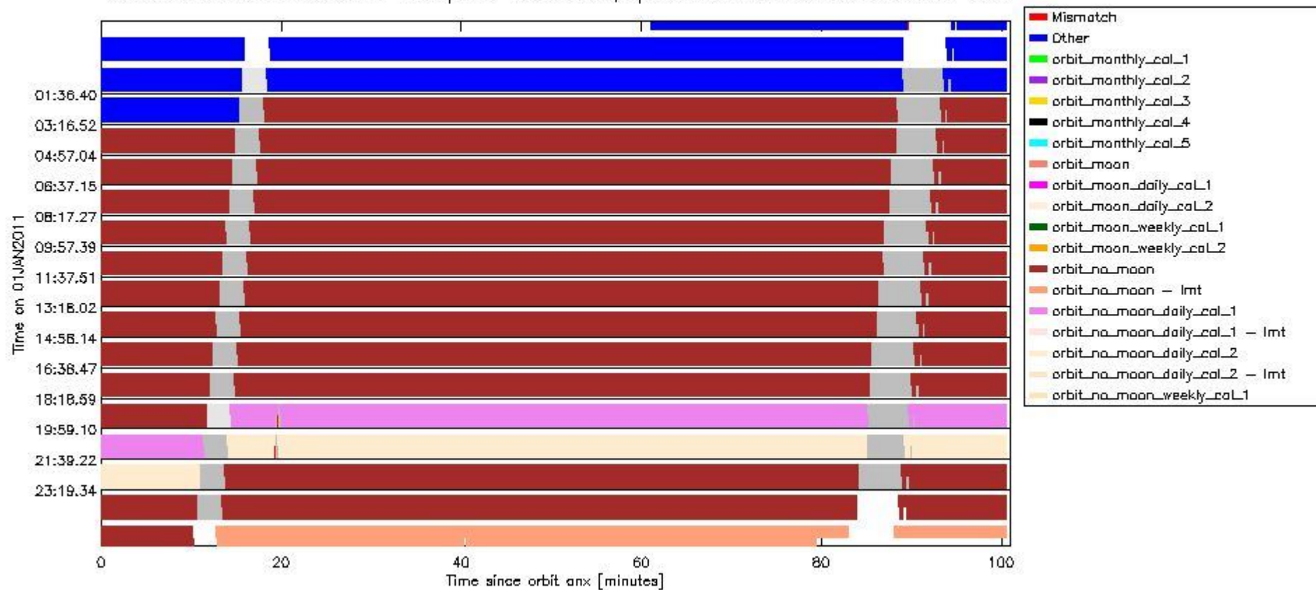
sciamachy_daily_report_level0_KSPT_L0_4504_N_20110101_6.PNG
