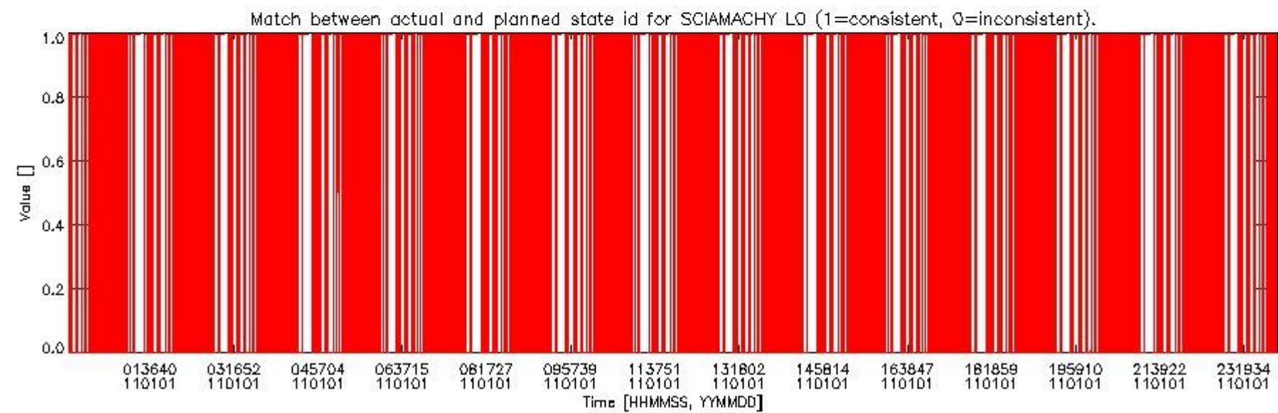
sciamachy_daily_report_level0_KSPT_L0_4504_N_20110101_5.PNG
