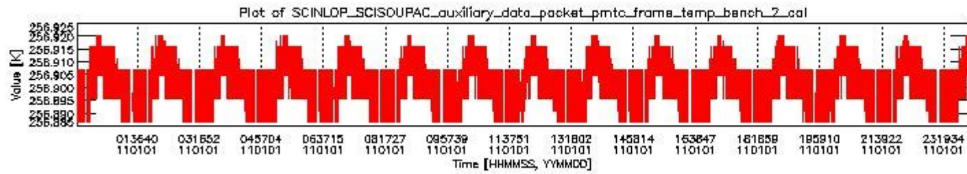
sciamachy_daily_report_level0_KSPT_L0_4504_N_20110101_1.PNG
