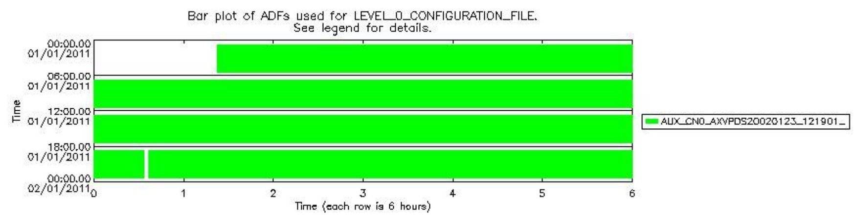
sciamachy_daily_report_level0_KSPT_L0_4504_N_20110101_7.PNG
