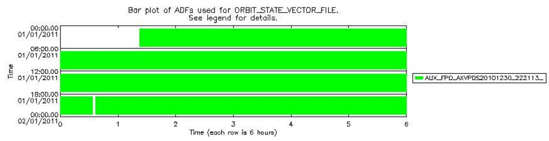
sciamachy_daily_report_level0_KSPT_L0_4504_N_20110101_8.PNG
